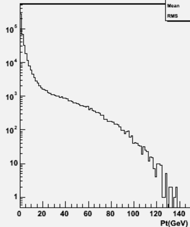
Start point Z : w100998 ddn1e1e1n1_o
