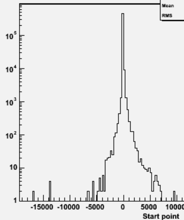
Start point Z : w100998 ddn1e1e1n1_o
