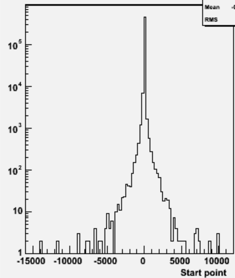
Start point Z : w100996 ddn1e1e1n1_o
