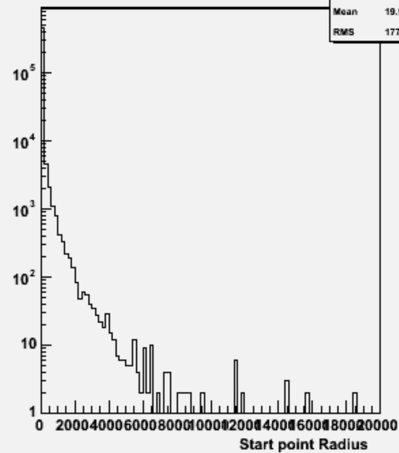
Start point R : w100996 ddn1e1e1n1_o
