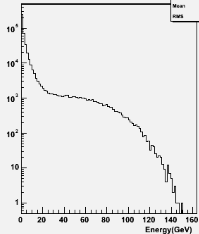
Start point R : w100996 ddn1e1e1n1_o
