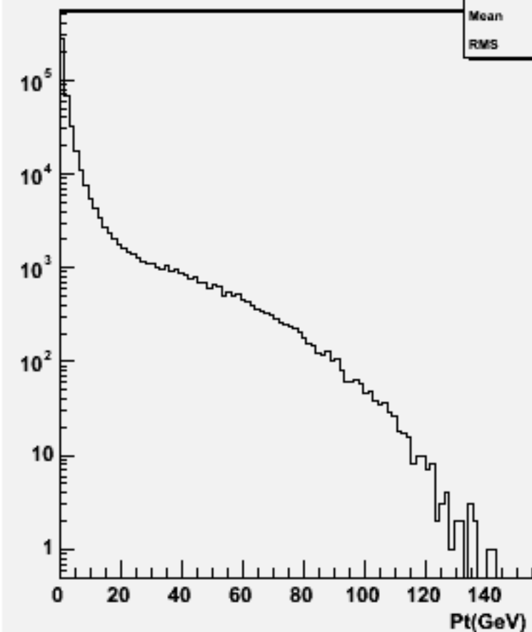
Start point Z : w100995 ddn1e1e1n1_o
