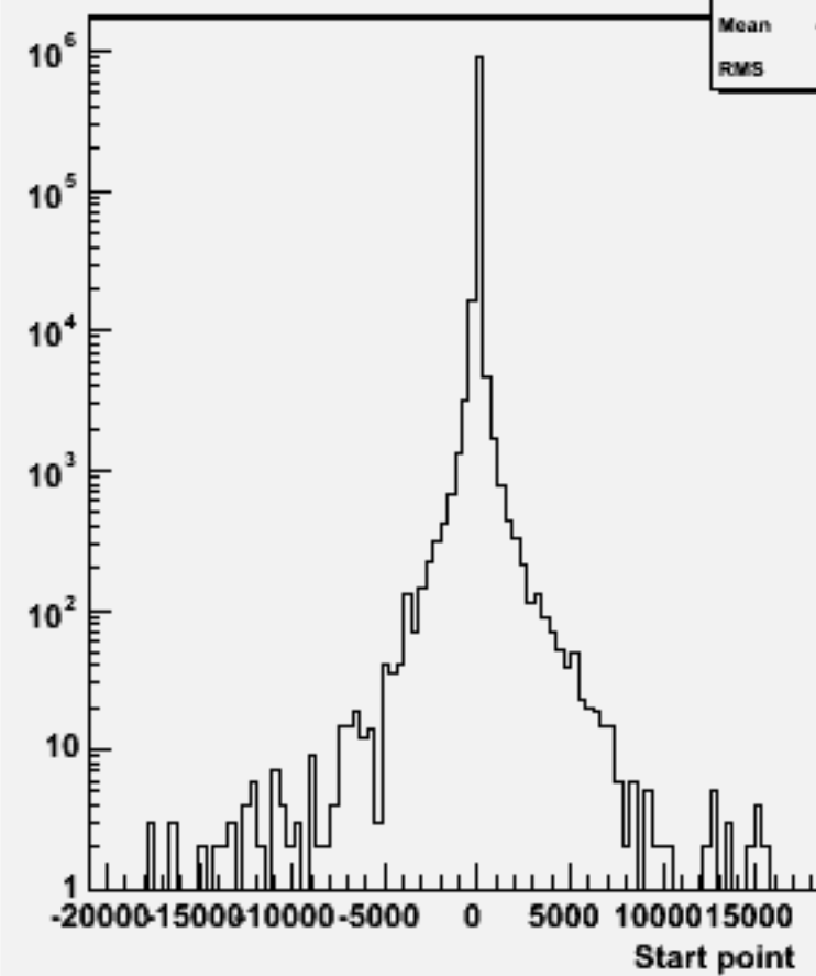
Start point Z : w100992 e3e3cssc_o
