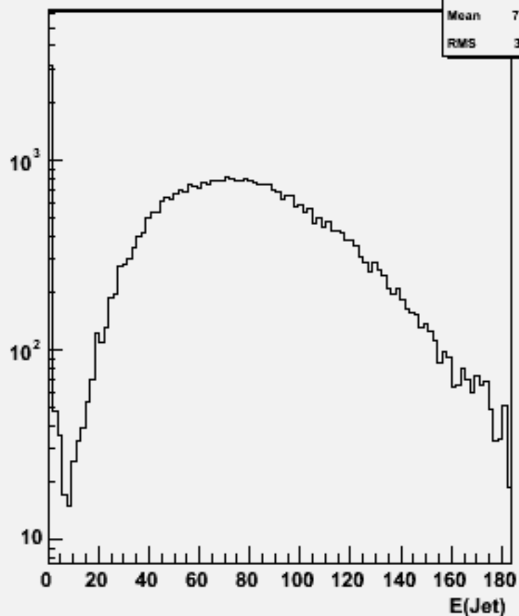
Jet energies(All jets)w100992 e3e3cssc_o
