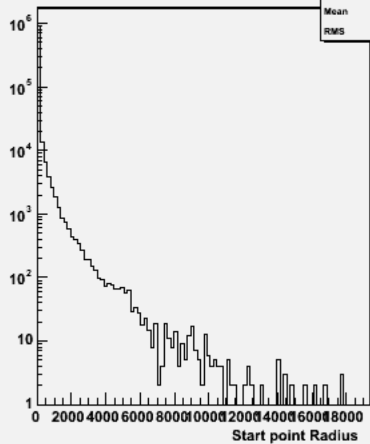
Start point R : w100992 e3e3cssc_o
