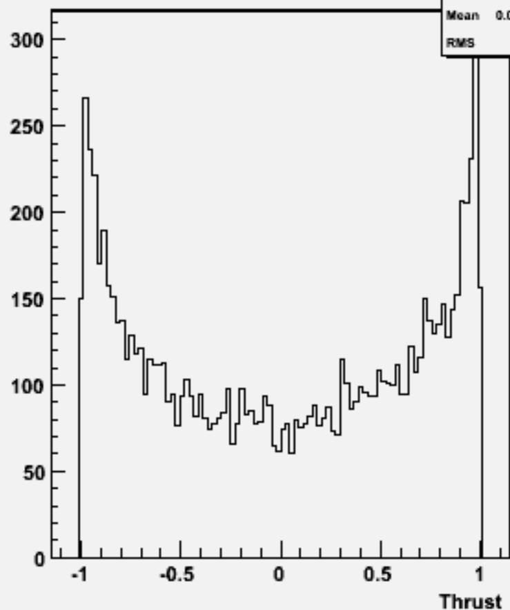
cos \Theta (thrust) w100992 e3e3cssc_o
