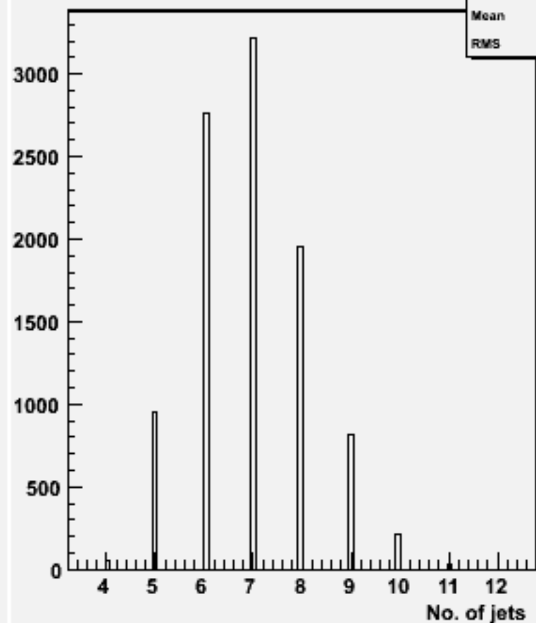
No. jets (ycut=0.001) : w100992 e3e3cssc_o
