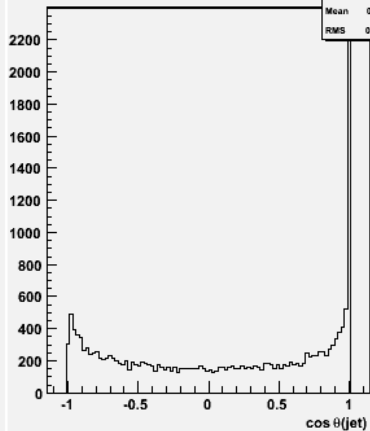
cos \theta for 2-jets :w100992 e3e3cssc_o
