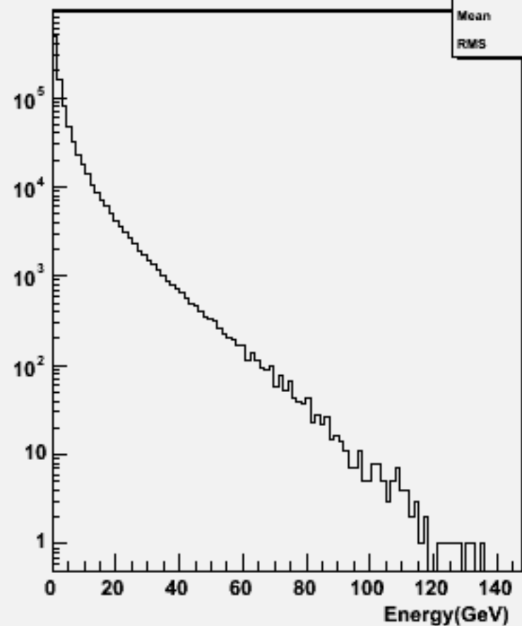
Particle Energy : w100992 e3e3cssc_o
