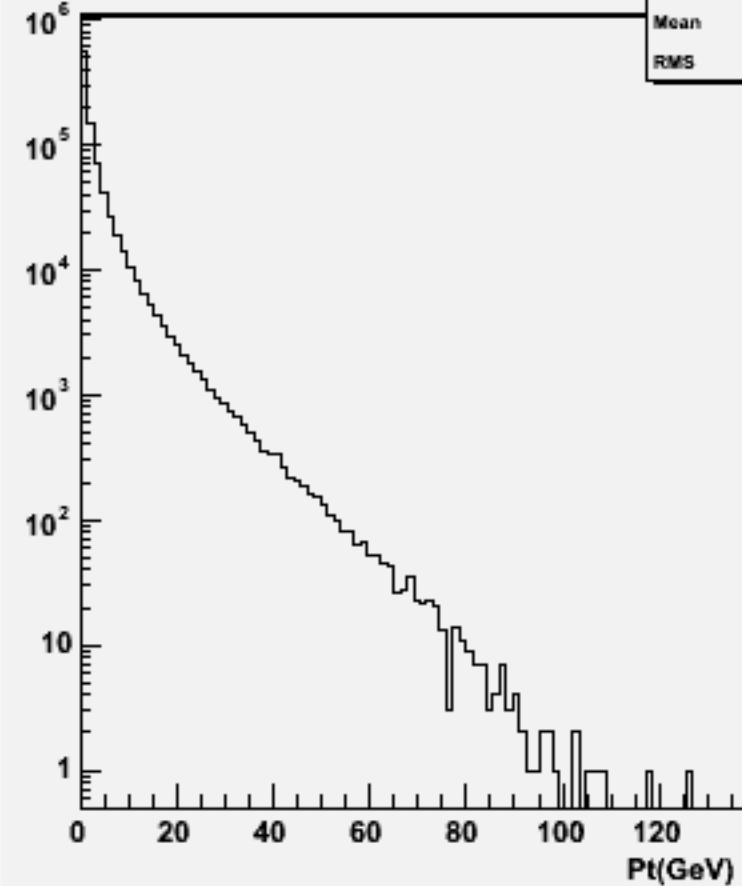
Particle Pt : w100992 e3e3cssc_o
