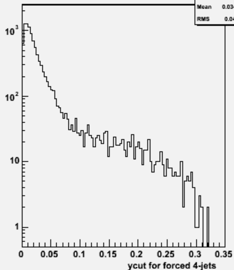
Ycut for 4-jets :w100992 e3e3cssc_o
