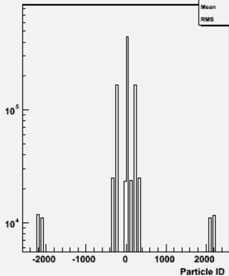
Particle ID : w100992 e3e3cssc_o
