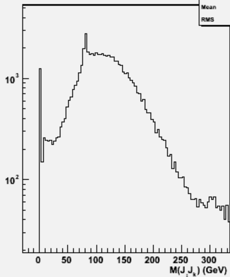
2jets mass(All comb)w100992 e3e3cssc_o
