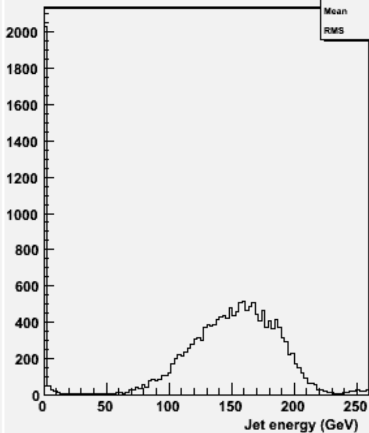
energy for 2-jets :w100992 e3e3cssc_o
