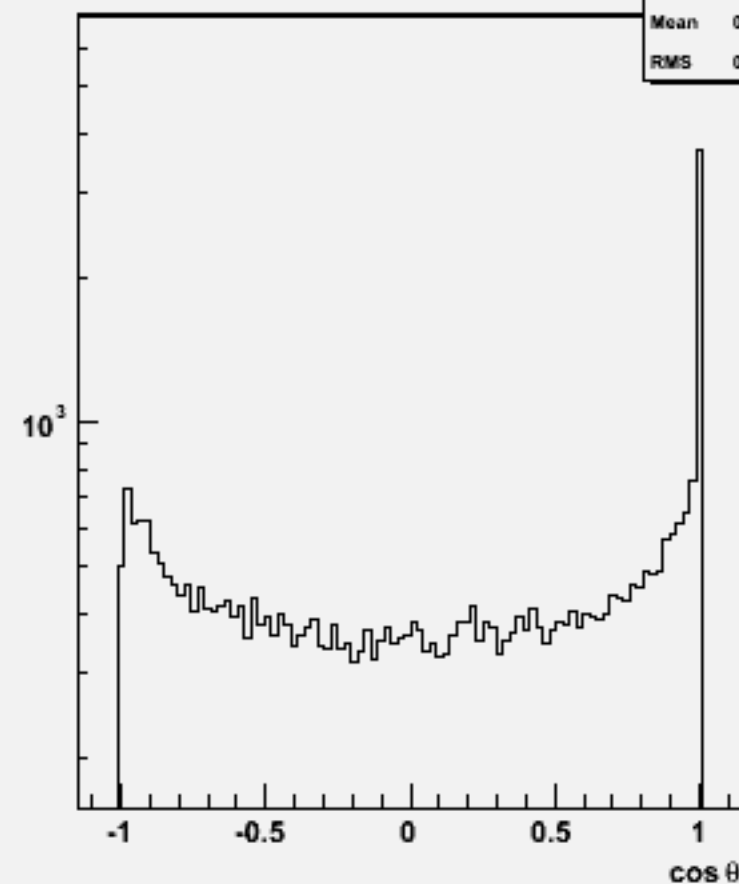
Jet cosθ (All jets)w100992 e3e3cssc_o
