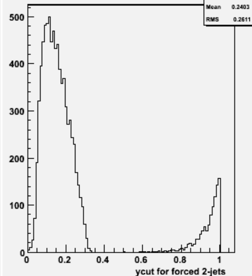
Ycut for 2-jets :w100992 e3e3cssc_o
