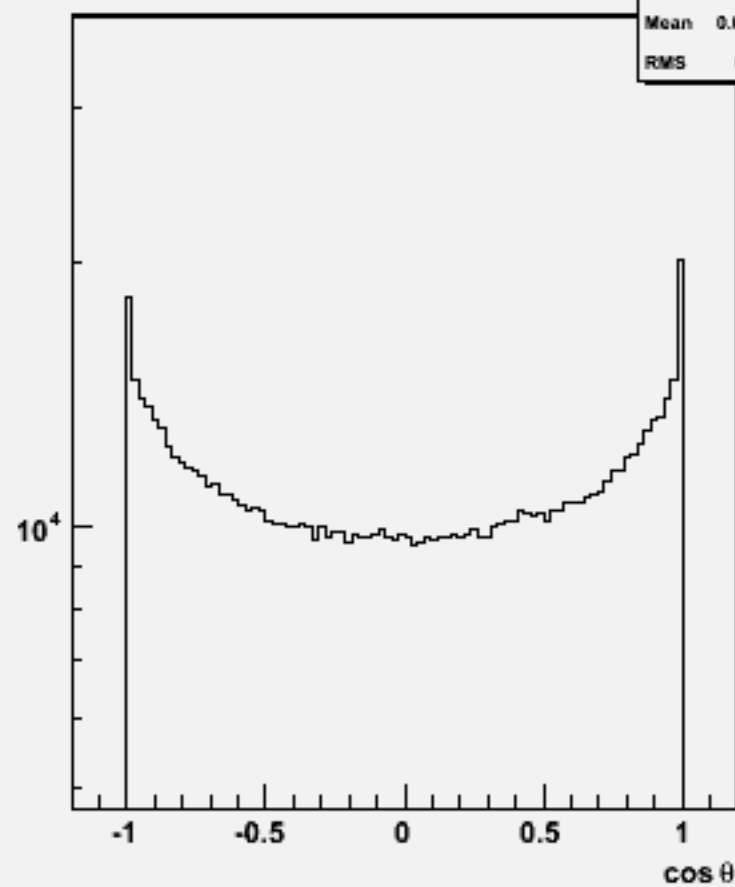
Particle cosθ : w100992 e3e3cssc_o
