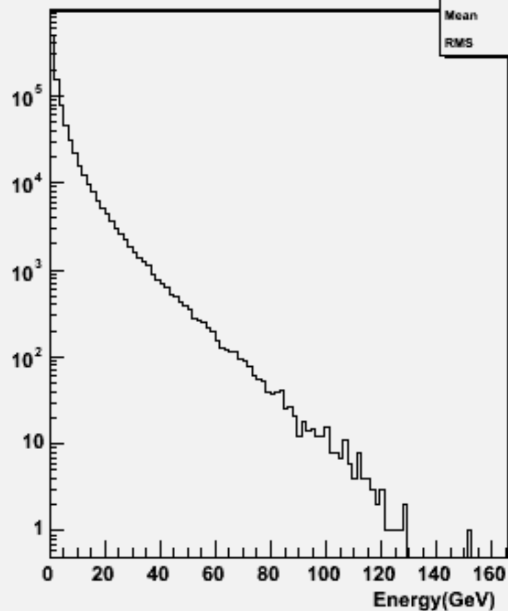
Particle Energy : w100989 e3e3csdu_o
