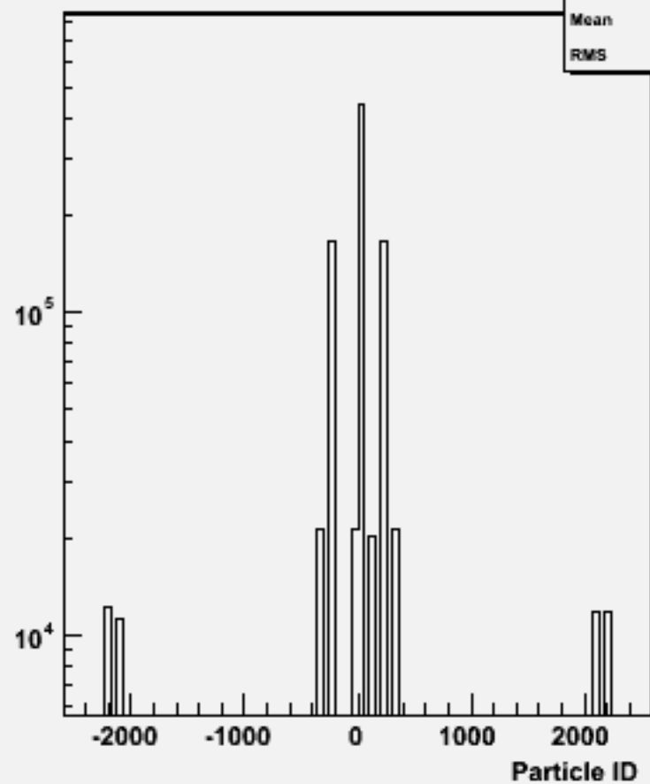
Particle ID : w100989 e3e3csdu_o
