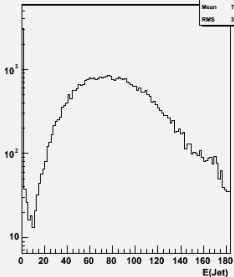
Jet energies(All jets)w100989 e3e3csdu_o
