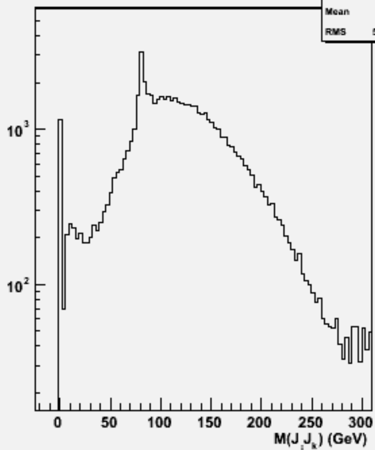
2jets mass(All comb)w100989 e3e3csdu_o
