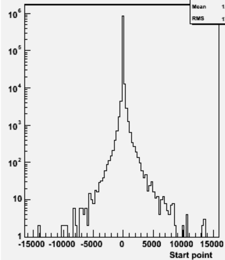
Start point Z : w100989 e3e3csdu_o
