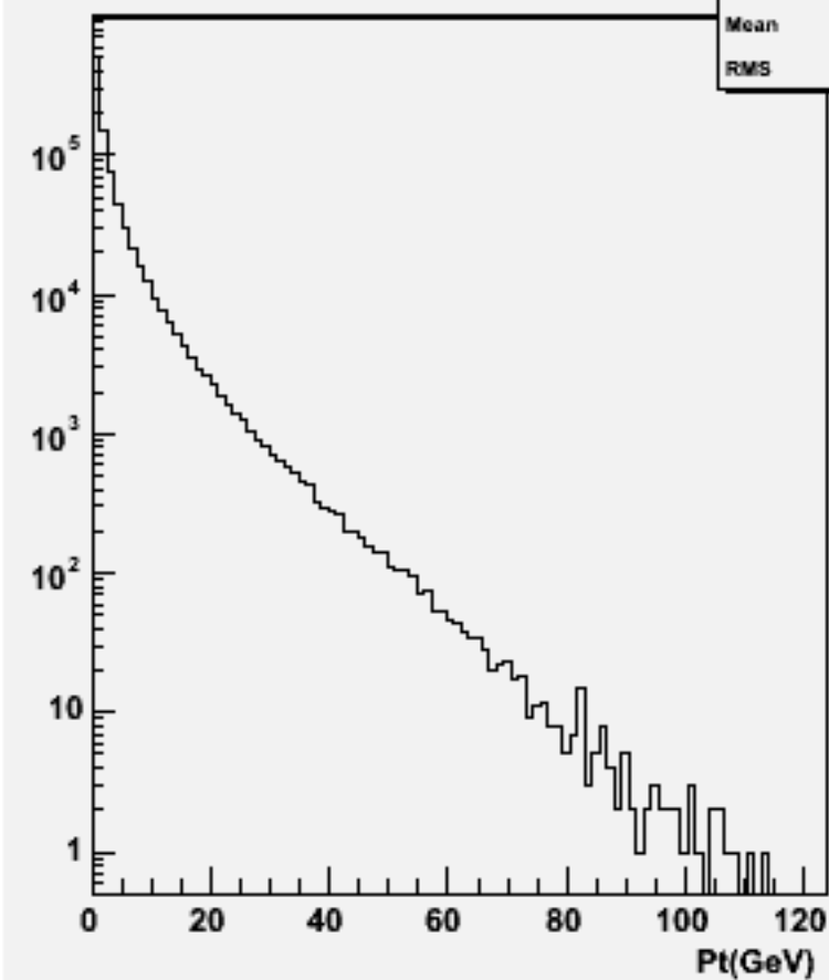
Particle Pt : w100989 e3e3csdu_o
