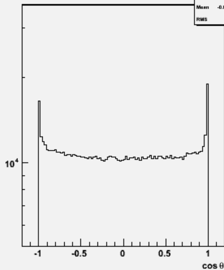
Particle cos \theta : w100989 e3e3csdu_o
