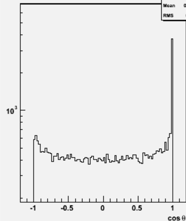
Jet cosθ (All jets)w100989 e3e3csdu_o
