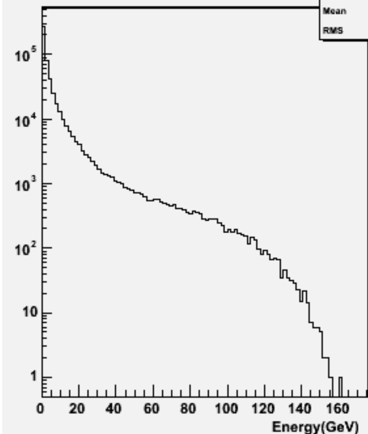
Particle Energy : w100978 e3e3cse1n1_o
