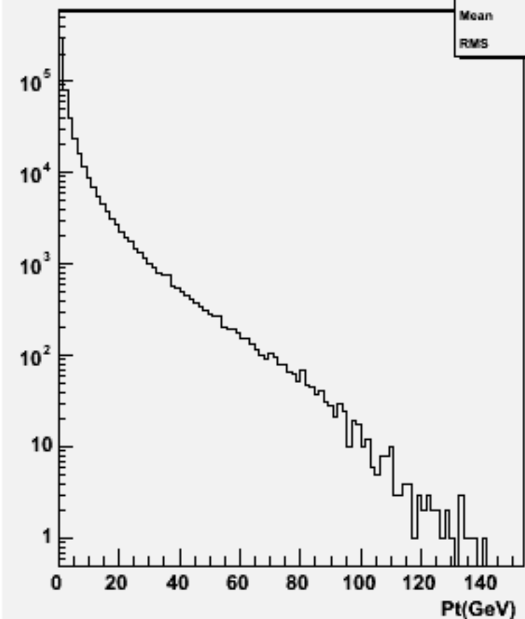
Particle Pt : w100978 e3e3cse1n1_o
