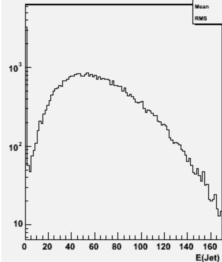
Jet energies(All jets)w100978 e3e3cse1n1_o
