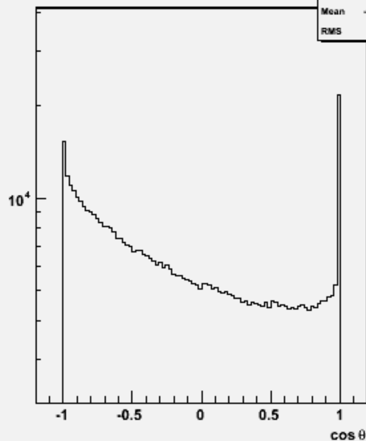
Particle cos \theta : w100978 e3e3cse1n1_o
