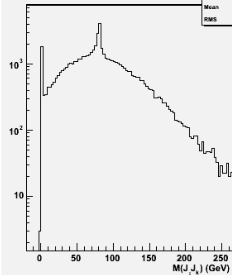
2jets mass(All comb)w100978 e3e3cse1n1_o
