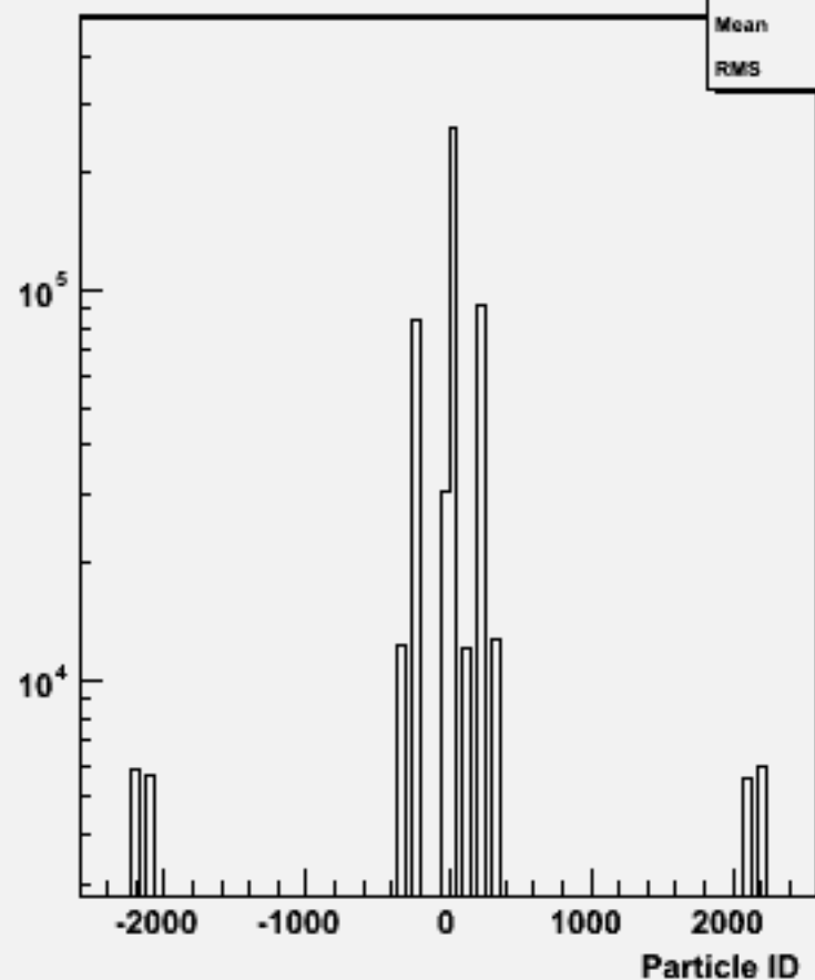
Particle ID : w100978 e3e3cse1n1_o
