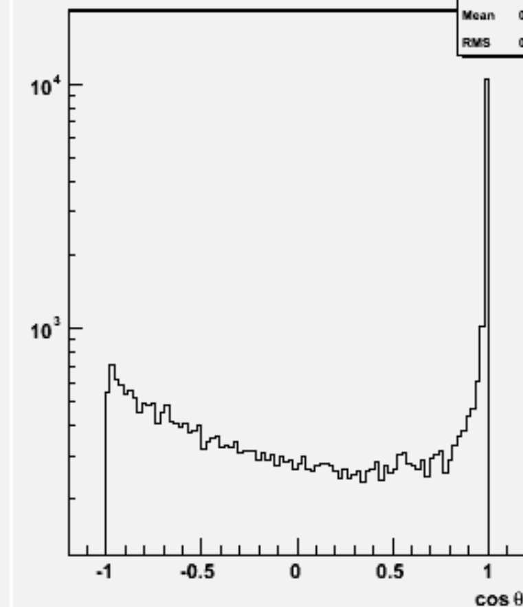
Jet cos \theta (All jets)w100978 e3e3cse1n1_o
