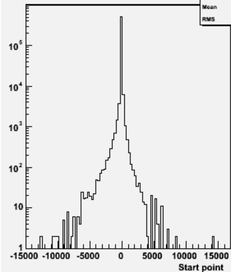
Start point Z : w100978 e3e3cse1n1_o
