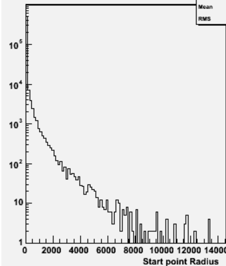
Start point R : w100978 e3e3cse1n1_o
