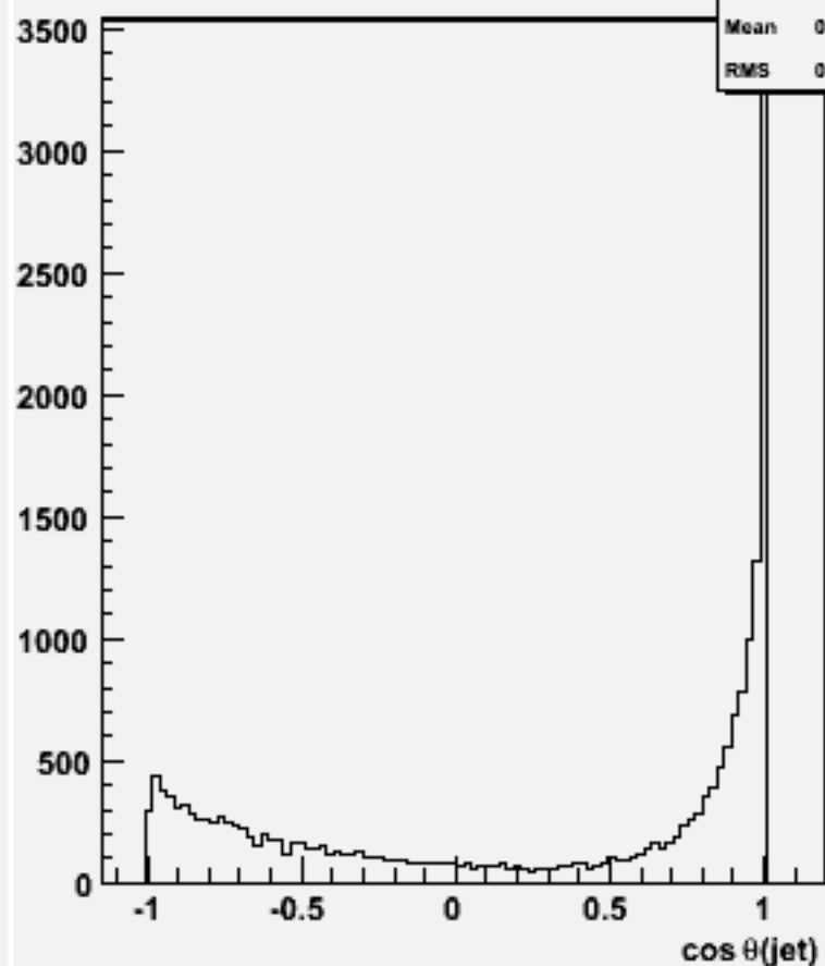
cos \theta for 2-jets :w100978 e3e3cse1n1_o
