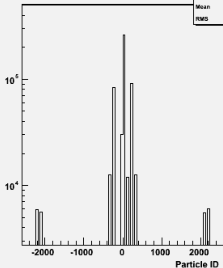
Particle ID : w100977 e3e3cse1n1_o
