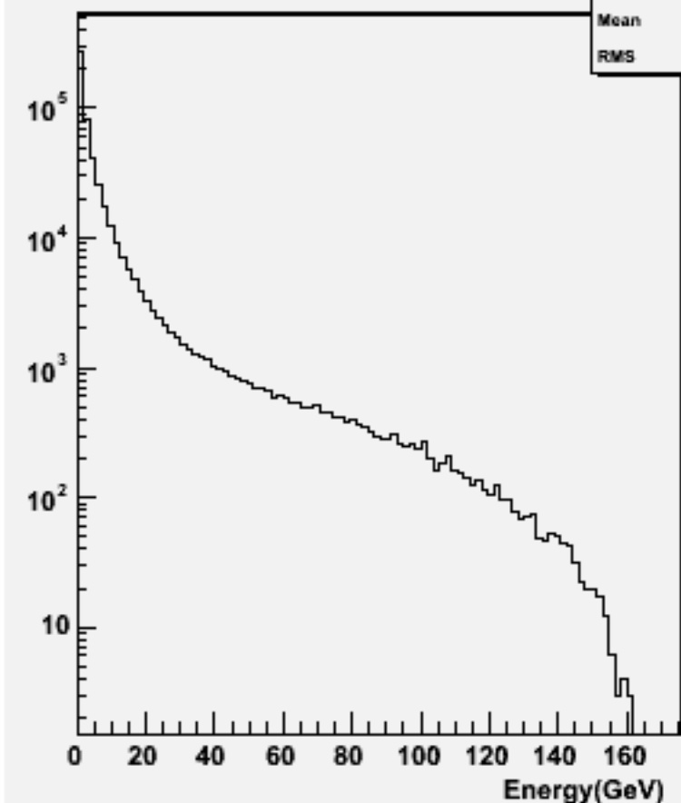
Particle Energy : w100977 e3e3cse1n1_o
