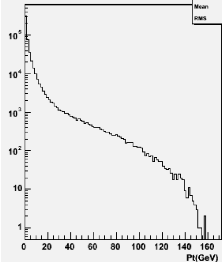
Particle Pt : w100977 e3e3cse1n1_o
