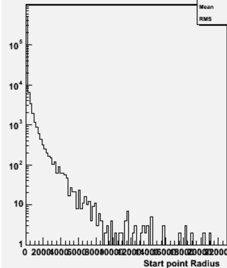
Start point R : w100977 e3e3cse1n1_o
