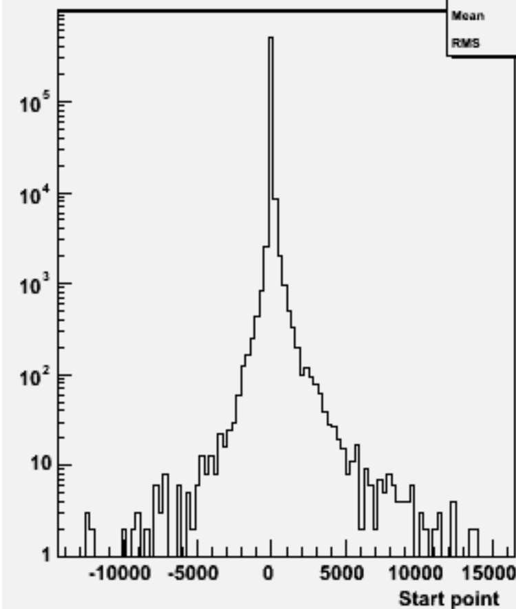
Start point Z : w100977 e3e3cse1n1_o
