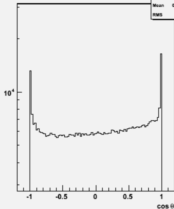
Particle \cos\theta : w100977 e3e3cse1n1_o
