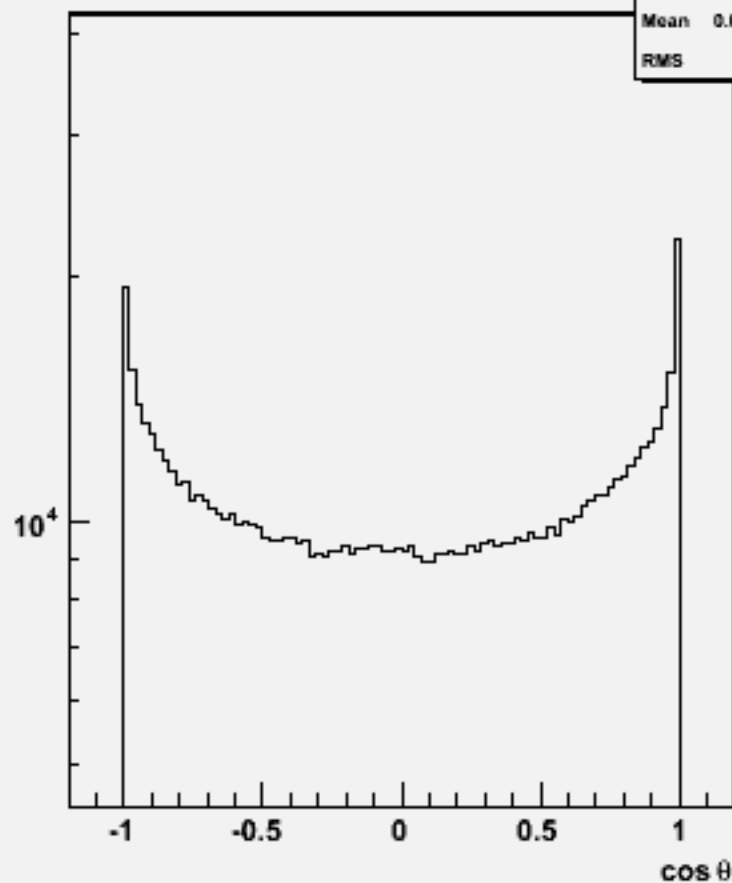
Particle cos \theta : w100969 e3e3uddu_o
