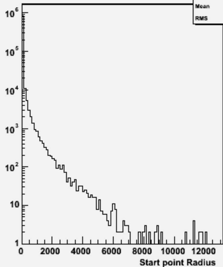
Start point R : w100969 e3e3uddu_o
