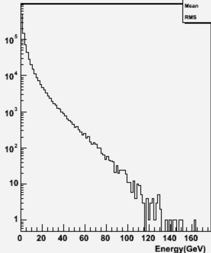
Particle Energy : w100969 e3e3uddu_o
