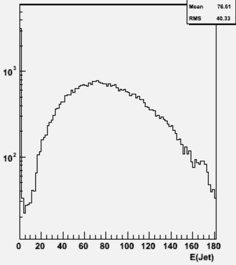
Jet energies(All jets)w100969 e3e3uddu_o
