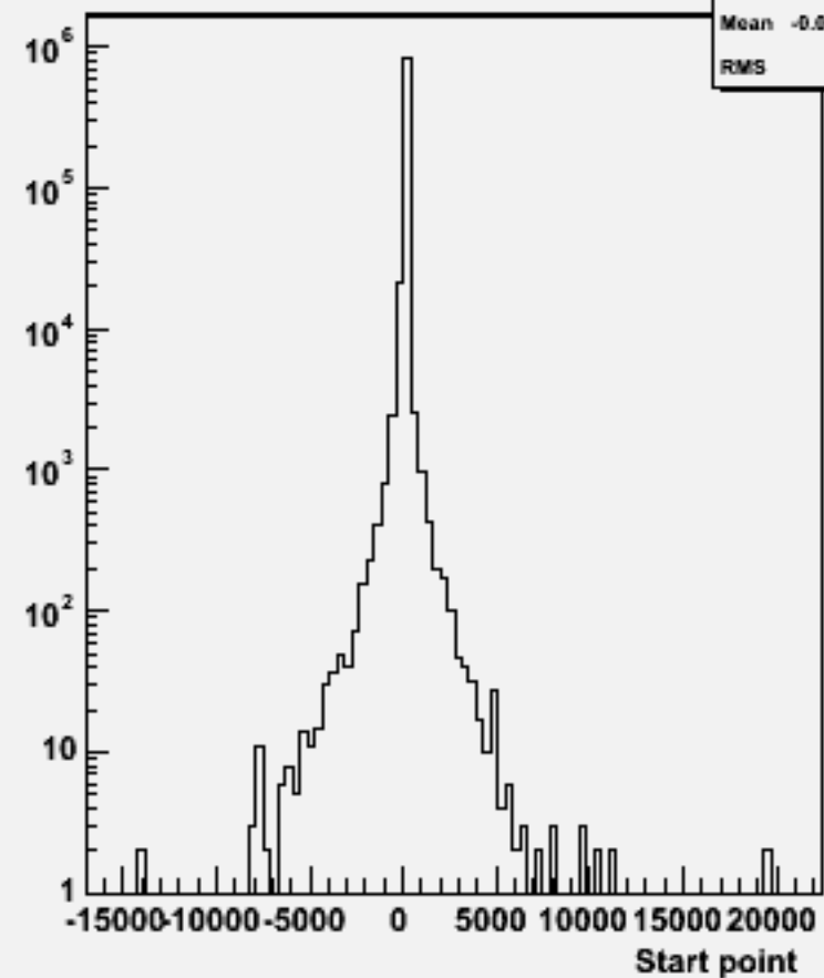
Start point Z : w100969 e3e3uddu_o
