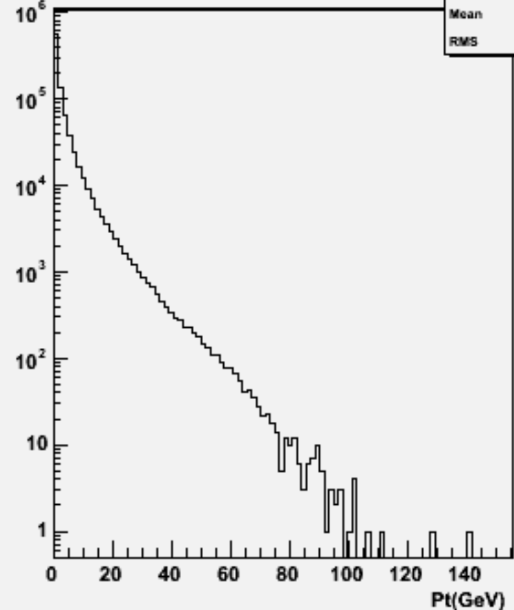
Particle Pt : w100969 e3e3uddu_o
