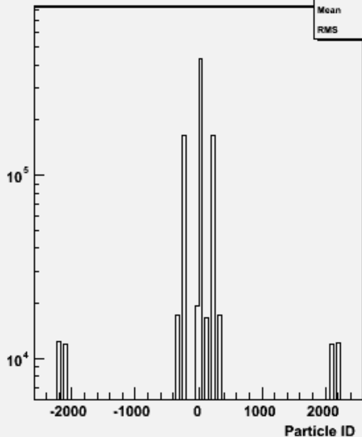
Particle ID : w100969 e3e3uddu_o
