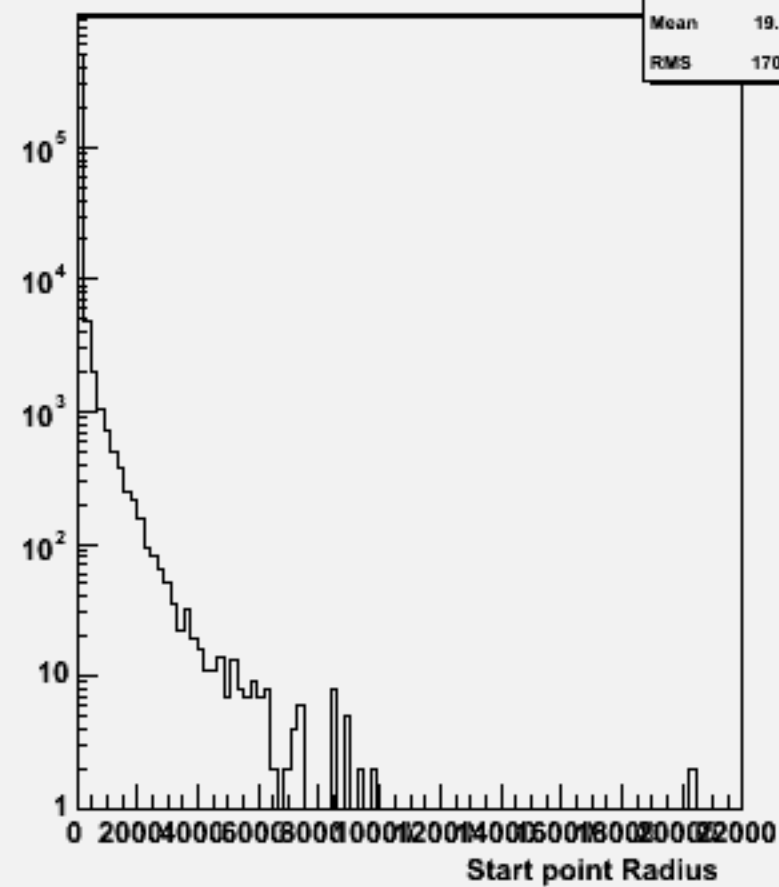
Start point R : w100957 e3e3ude1n1_o
