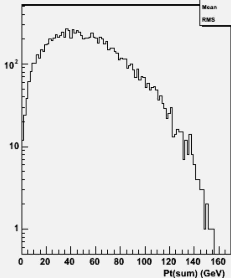
Pt Sum: w100957 e3e3ude1n1_o
