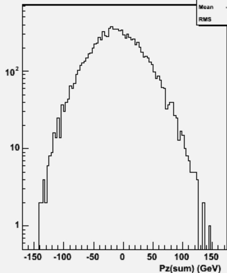
Pz Sum: w100957 e3e3ude1n1_o
