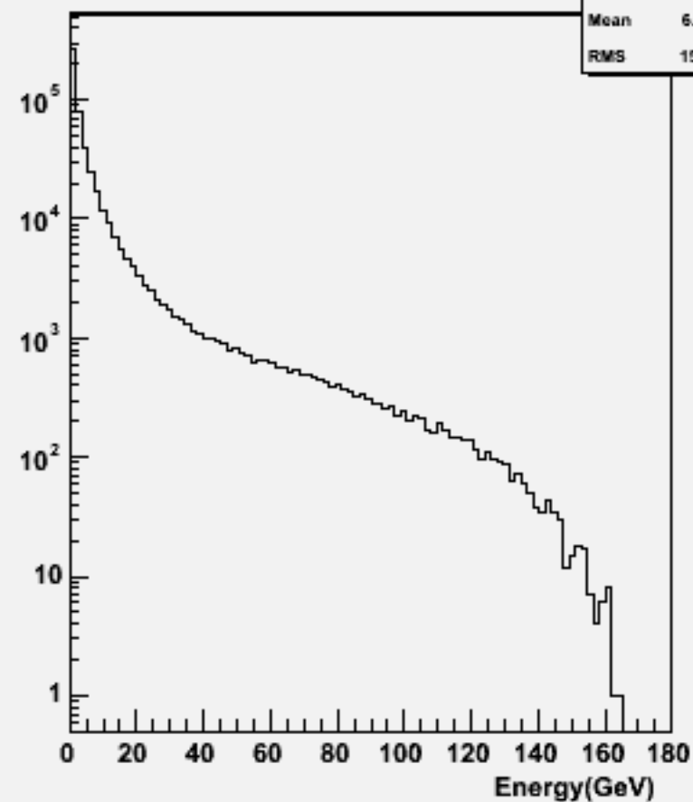
Start point R : w100957 e3e3ude1n1_o
