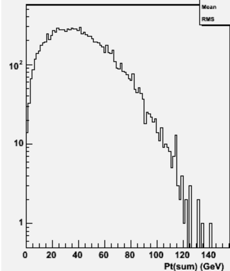
Pt Sum: w100956 e3e3ude1n1_o
