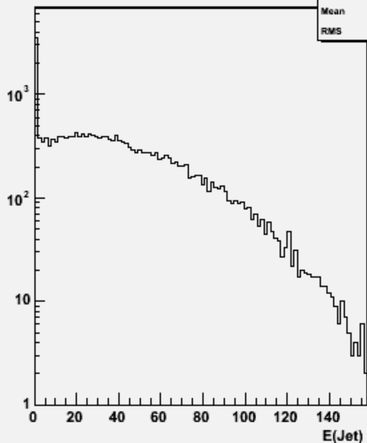
Jet energies(All jets)w100938 e3e3n3e3e1n1_o
