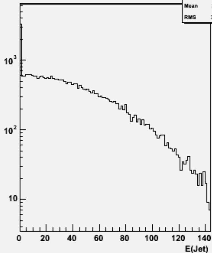
Jet energies(All jets)w100937 e3e3n3e3e1n1_o
