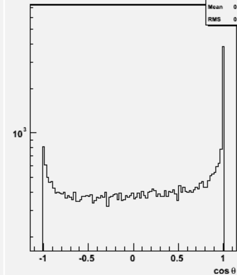
Jet cos \theta (All jets)w100933 e3e3n2e2sc_o
