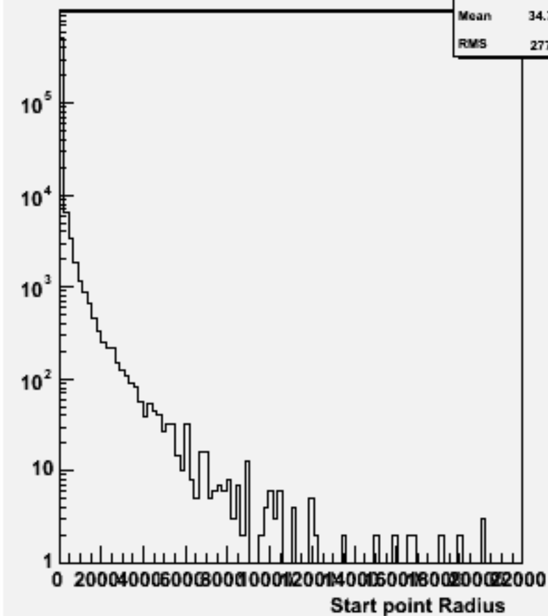
Start point R : w100933 e3e3n2e2sc_o
