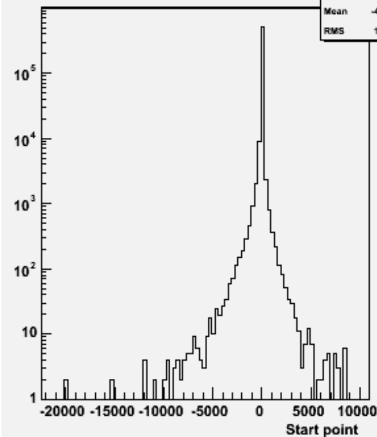
Start point Z : w100933 e3e3n2e2sc_o
