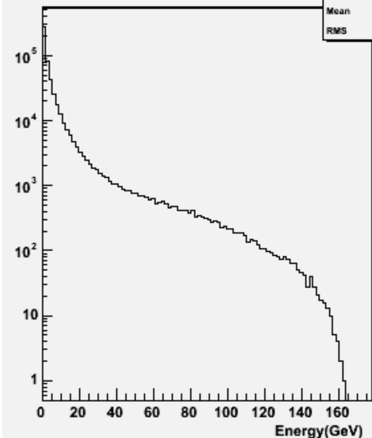
Start point R : w100933 e3e3n2e2sc_o
