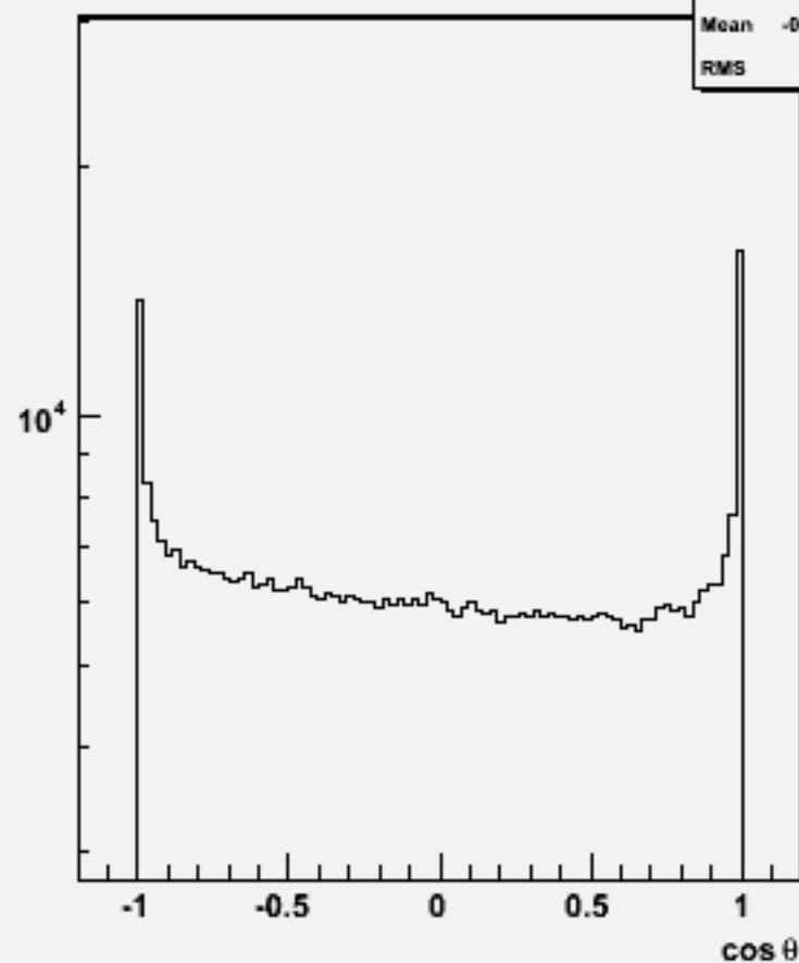
Particle cos \theta : w100933 e3e3n2e2sc_o
