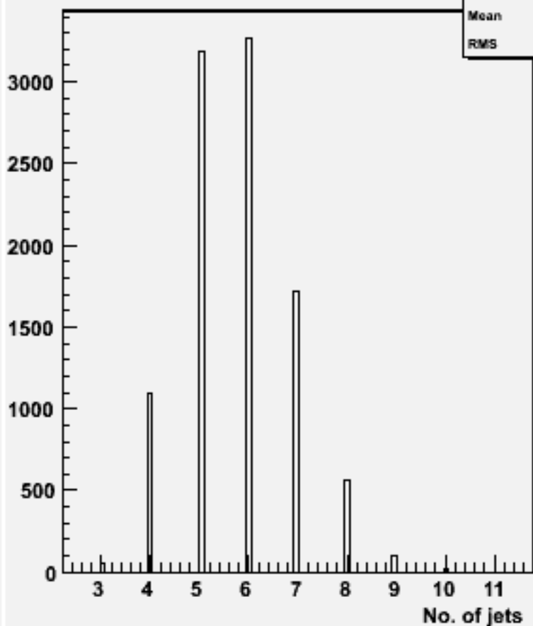
No. jets (ycut=0.001) : w100933 e3e3n2e2sc_o
