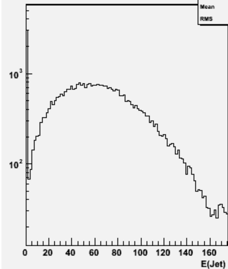
Jet energies(All jets)w100933 e3e3n2e2sc_o
