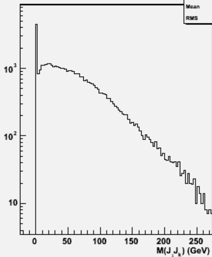
2jets mass(All comb)w100920 e3e3n2e2e2n2_o
