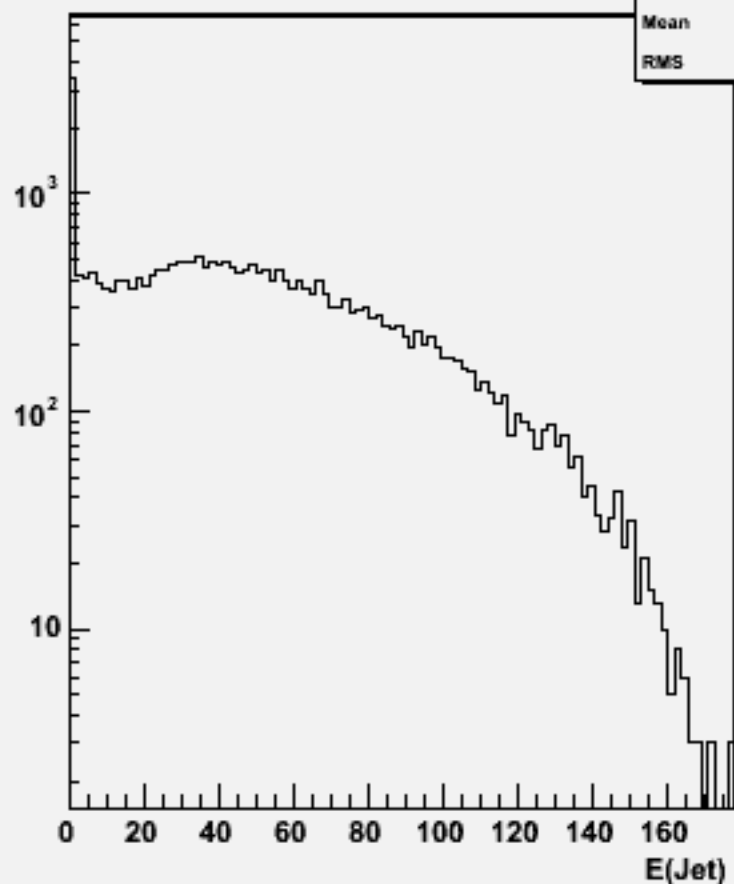
Jet energies(All jets)w100920 e3e3n2e2e2n2_o
