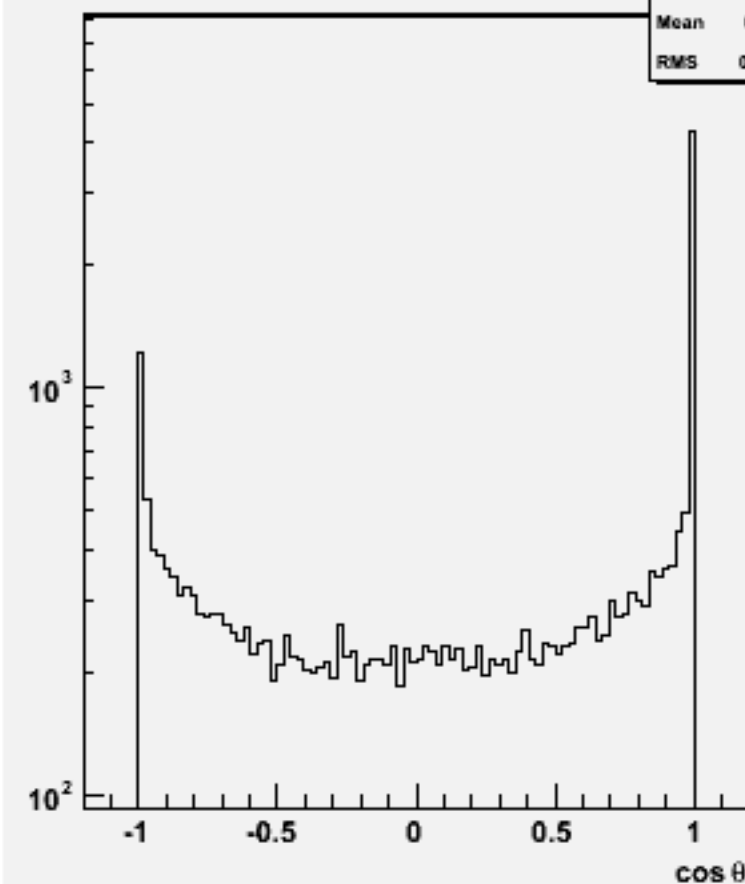
Jet cos \theta (All jets)w100920 e3e3n2e2e2n2_o
