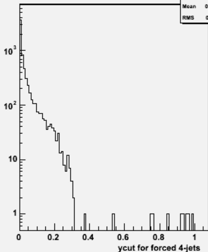
Ycut for 4-jets :w100920 e3e3n2e2e2n2_o
