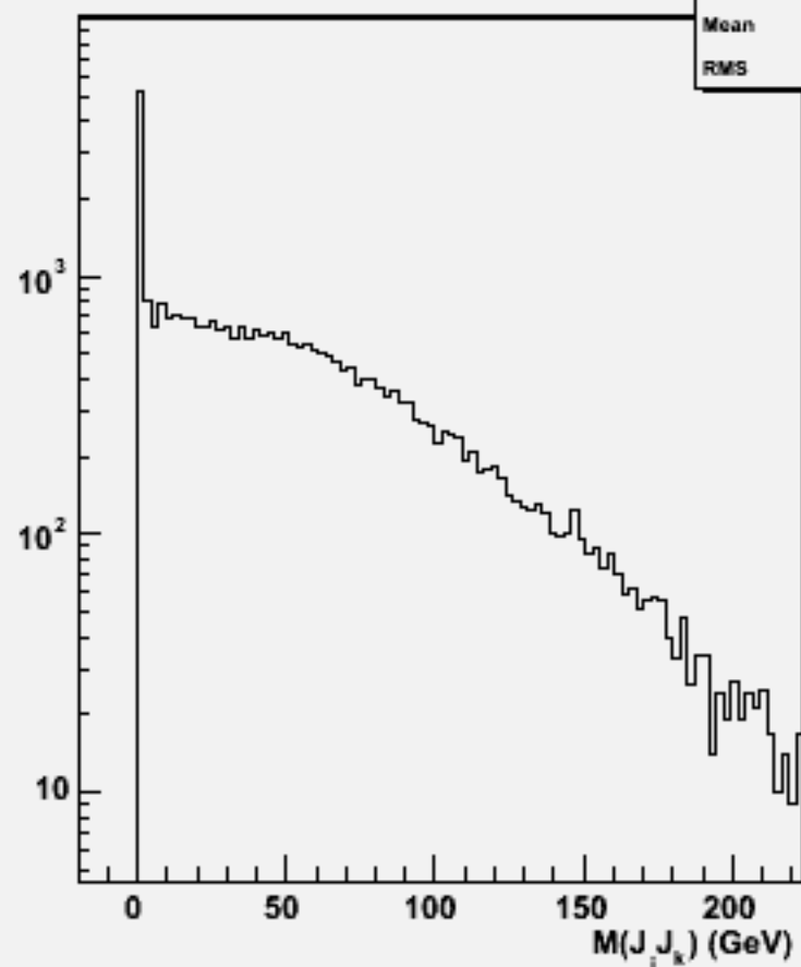
2jets mass(All comb)w100918 e3e3n2e2e1n1_o
