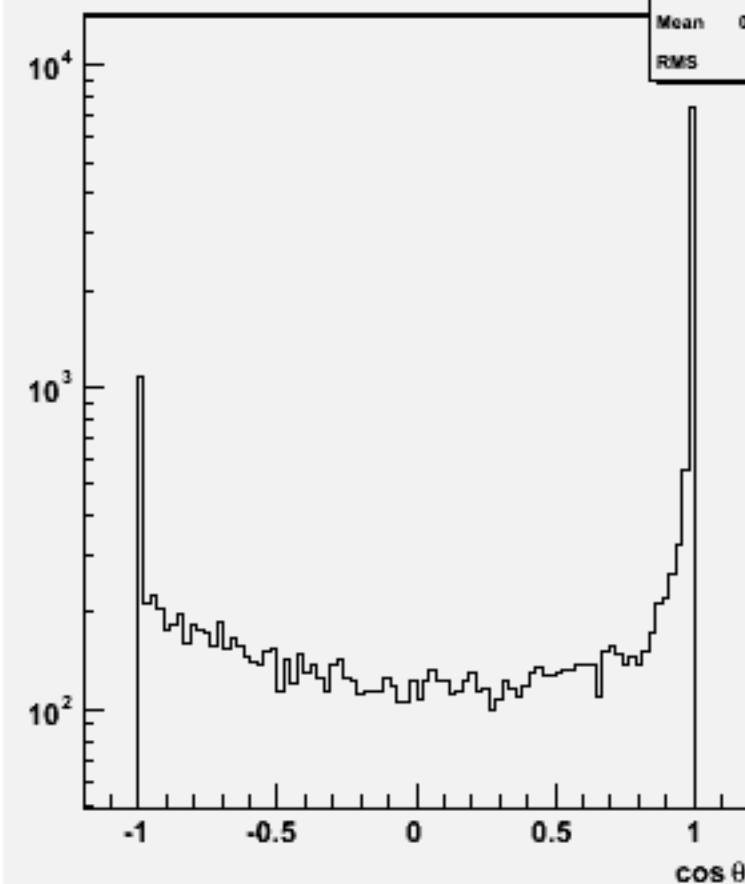
Jet cos \theta (All jets)w100918 e3e3n2e2e1n1_o
