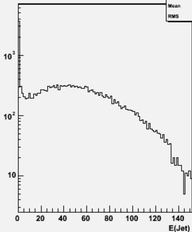
Jet energies(All jets)w100918 e3e3n2e2e1n1_o
