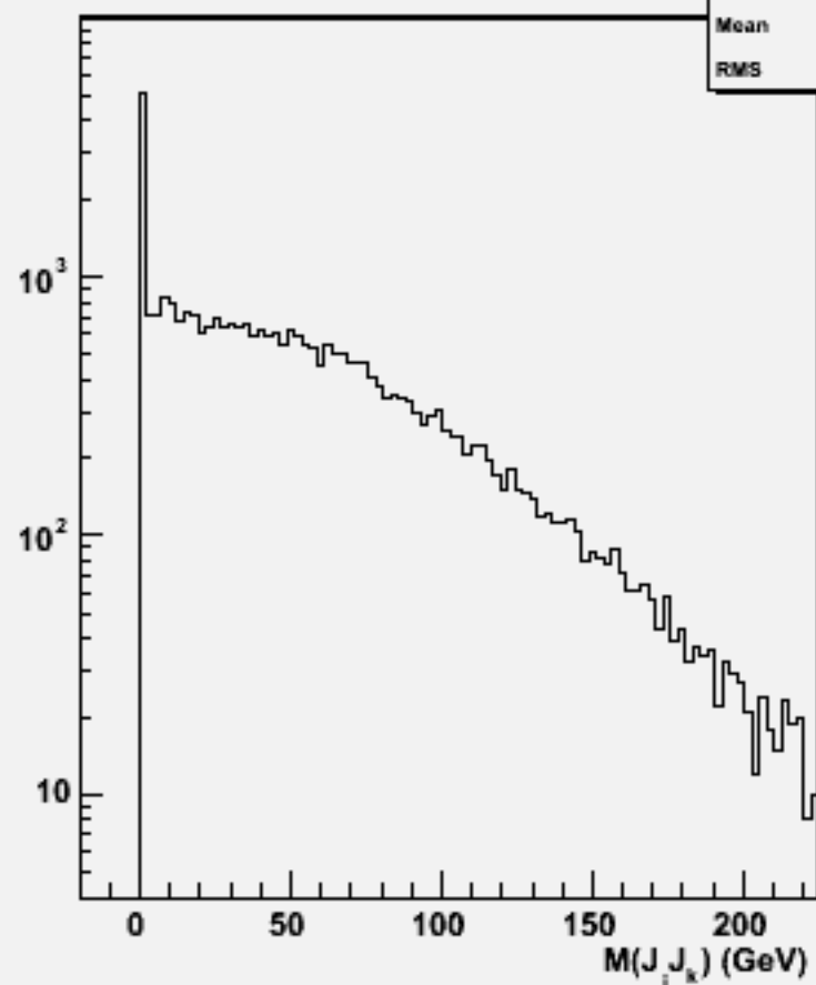
2jets mass(All comb)w100916 e3e3n2e2e1n1_o
