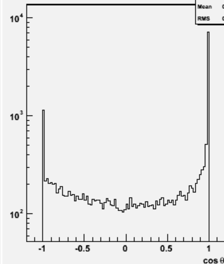
Jet cos \theta (All jets)w100916 e3e3n2e2e1n1_o
