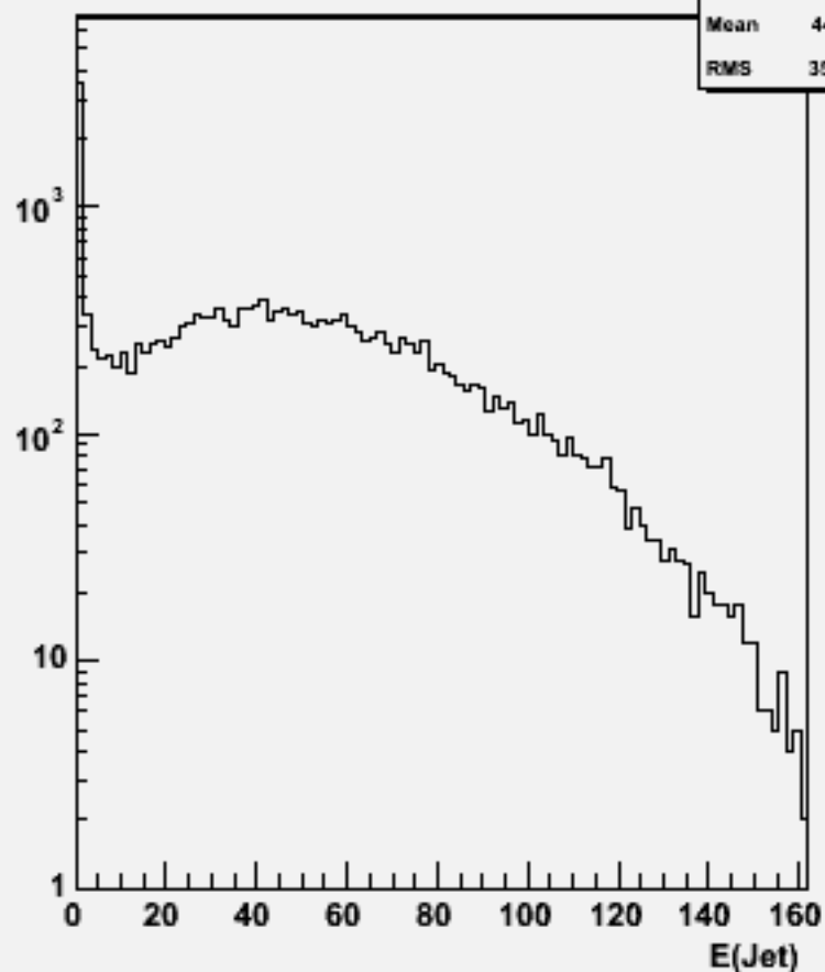
Jet energies(All jets)w100916 e3e3n2e2e1n1_o
