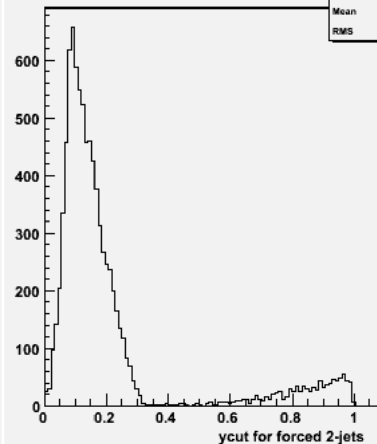
Ycut for 2-jets :w100913 e3e3n1e1sc_o
