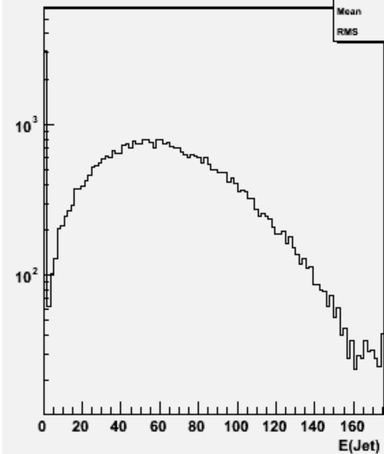
Jet energies(All jets)w100913 e3e3n1e1sc_o
