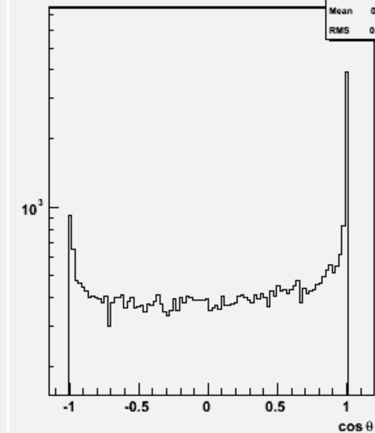
Jet cos \theta (All jets)w100913 e3e3n1e1sc_o
