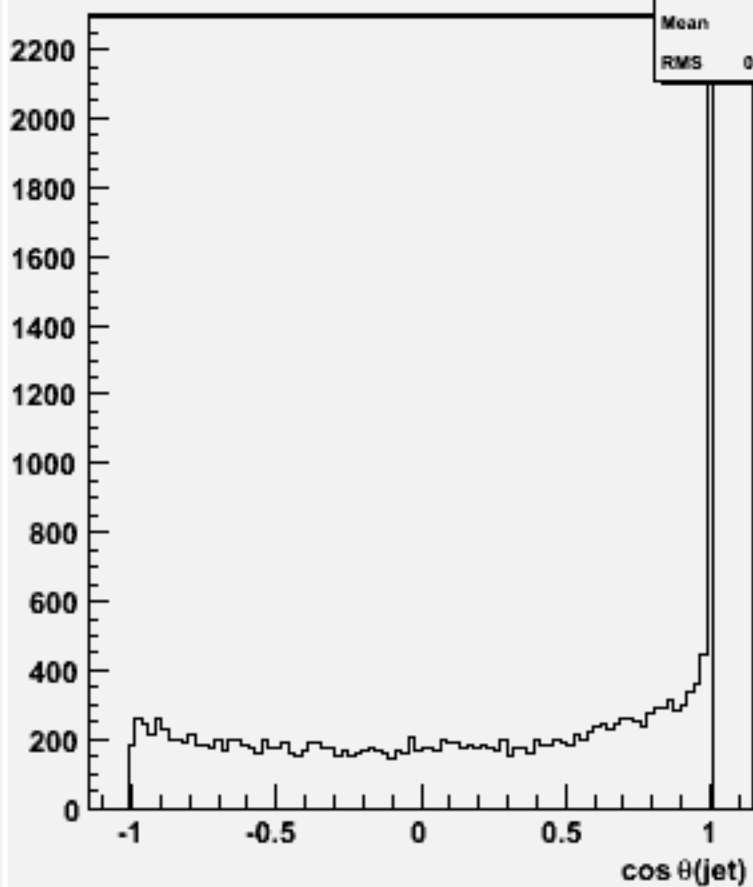
cos \theta for 2-jets :w100913 e3e3n1e1sc_o
