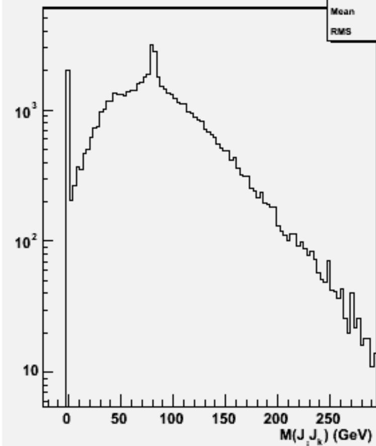
2jets mass(All comb)w100913 e3e3n1e1sc_o
