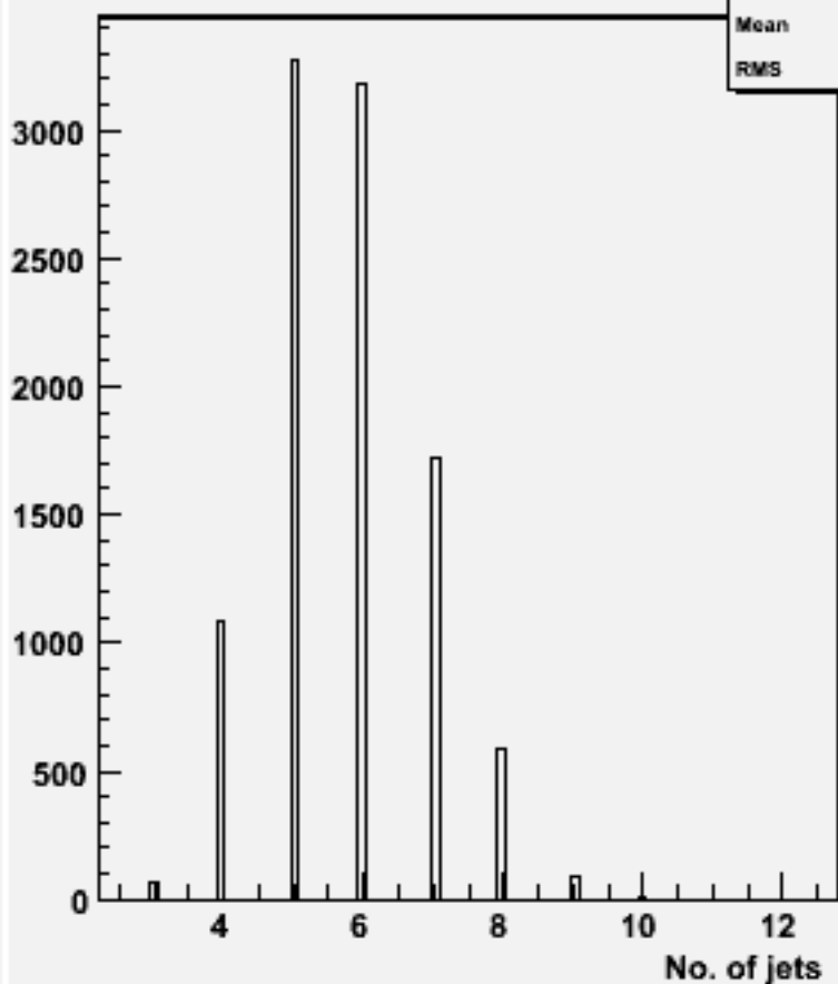
No. jets (ycut=0.001) : w100913 e3e3n1e1sc_o
