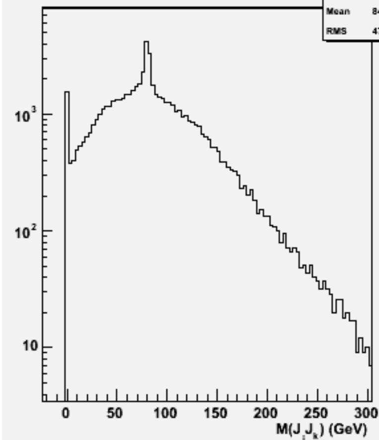
2jets mass(All comb)w100912 e3e3n1e1sc_o
