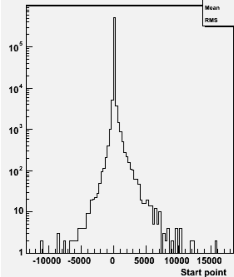
Start point Z : w100912 e3e3n1e1sc_o
