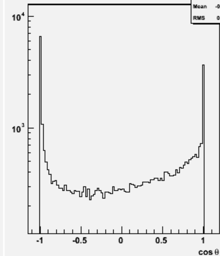
Jet cos \theta (All jets)w100912 e3e3n1e1sc_o
