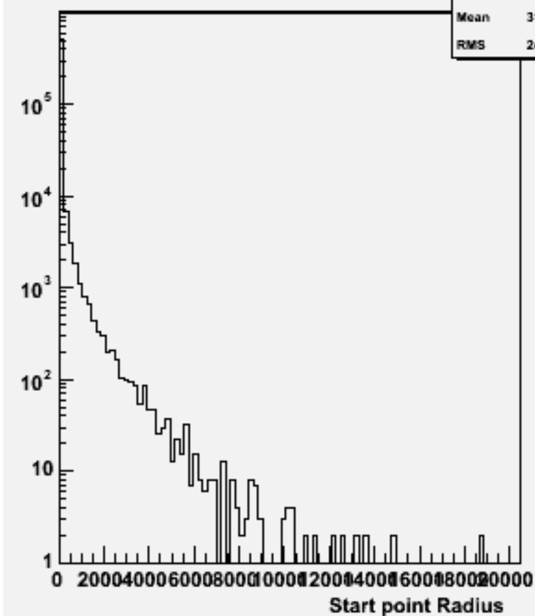
Start point R : w100912 e3e3n1e1sc_o
