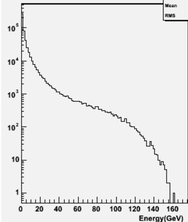
Particle Energy : w100912 e3e3n1e1sc_o
