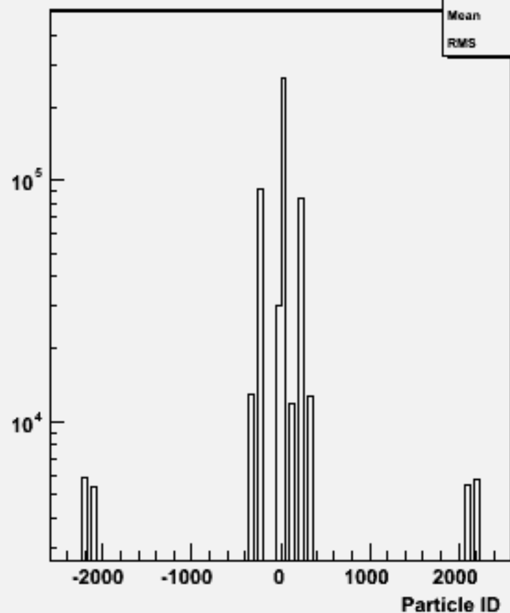
Particle ID : w100912 e3e3n1e1sc_o
