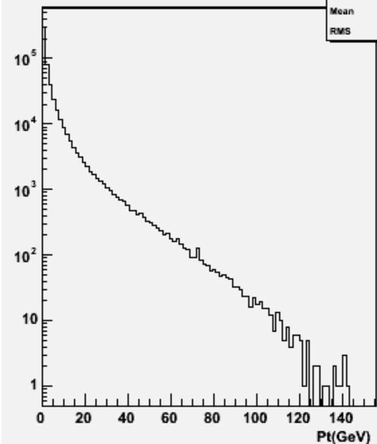
Particle Pt : w100912 e3e3n1e1sc_o
