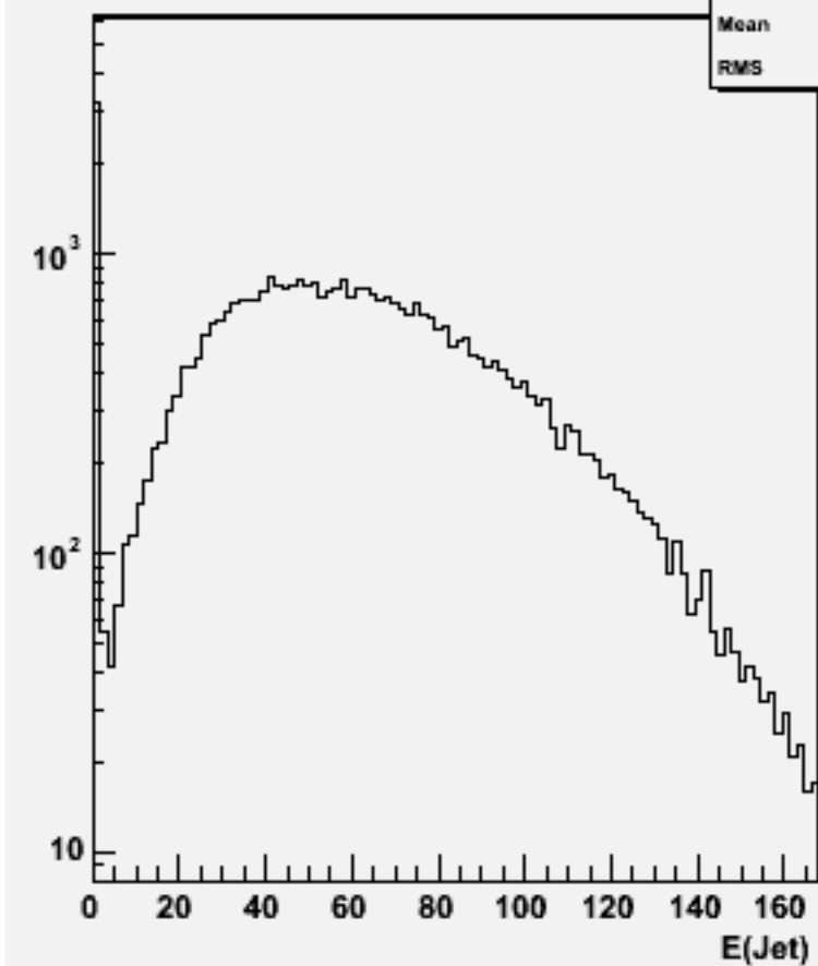
Jet energies(All jets)w100912 e3e3n1e1sc_o
