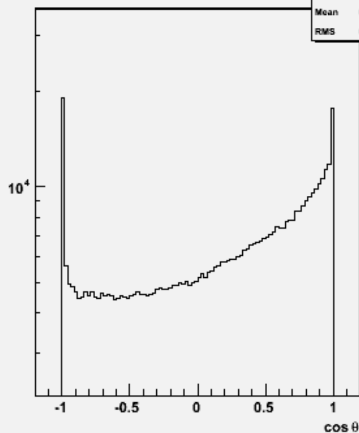
Particle cosθ : w100912 e3e3n1e1sc_o
