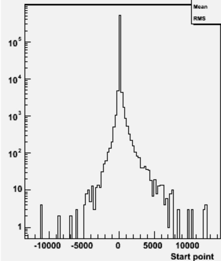
Start point Z : w100911 e3e3n1e1sc_o
