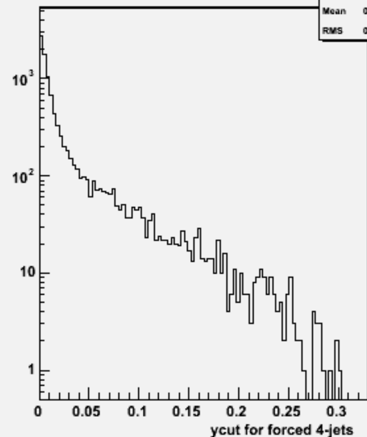
Ycut for 4-jets :w100911 e3e3n1e1sc_o
