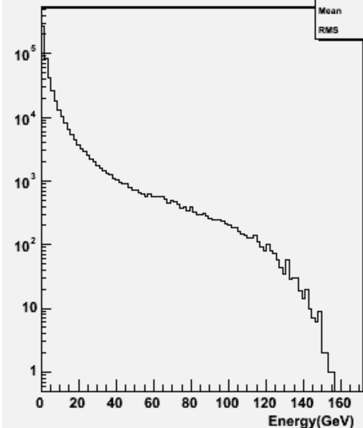
Particle Energy : w100911 e3e3n1e1sc_o
