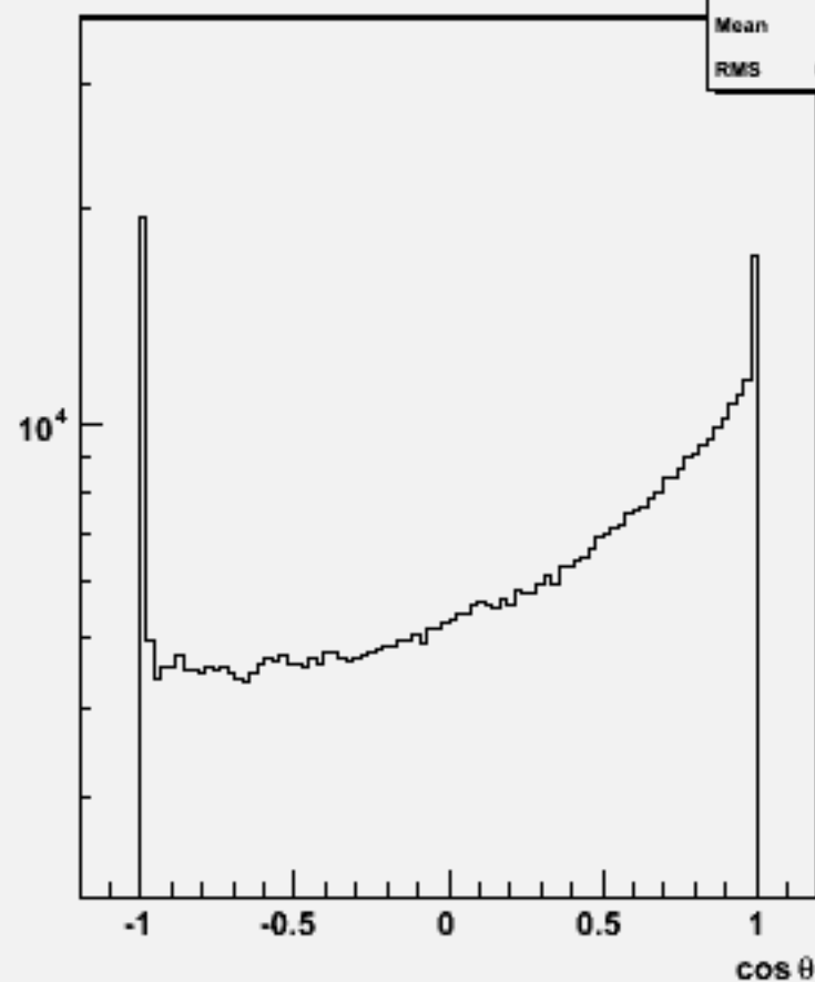
Particle cosθ : w100911 e3e3n1e1sc_o
