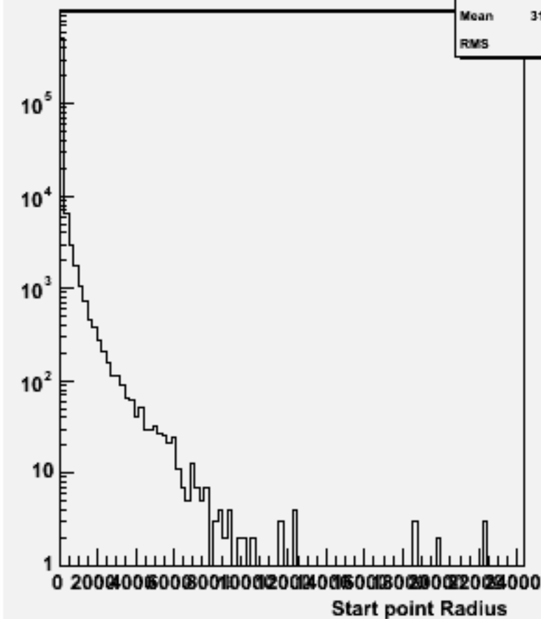
Start point R : w100911 e3e3n1e1sc_o
