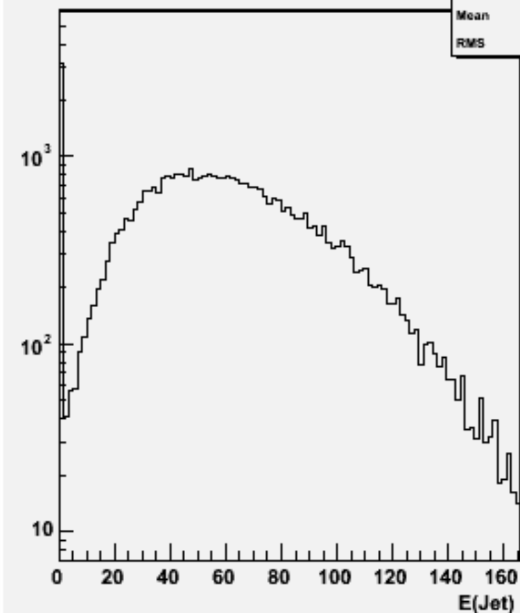
Jet energies(All jets)w100911 e3e3n1e1sc_o
