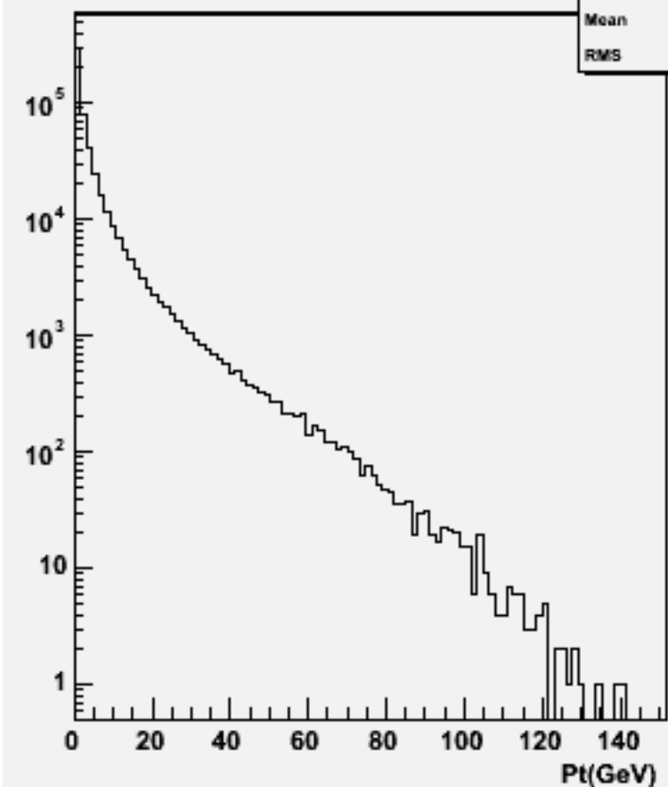
Particle Pt : w100911 e3e3n1e1sc_o
