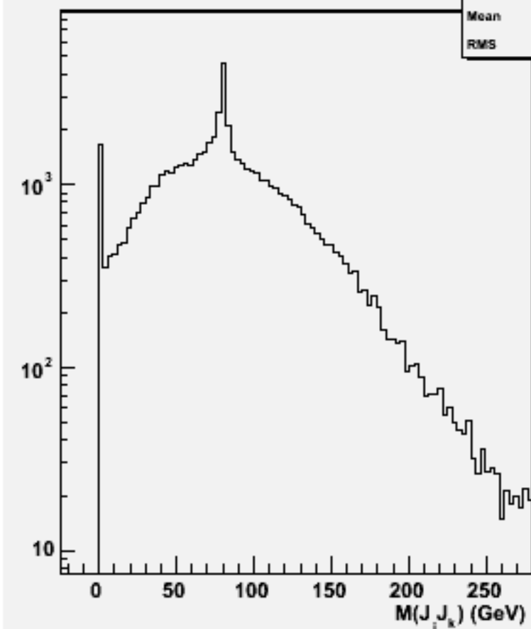
2jets mass(All comb)w100911 e3e3n1e1sc_o
