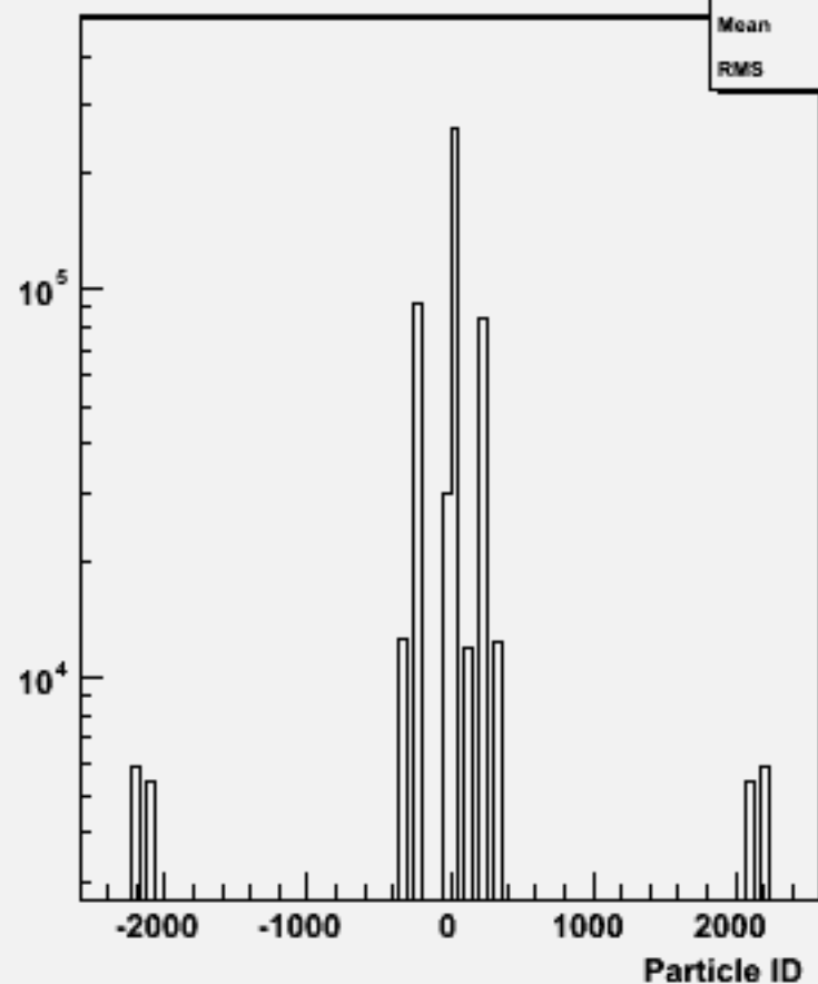
Particle ID : w100911 e3e3n1e1sc_o
