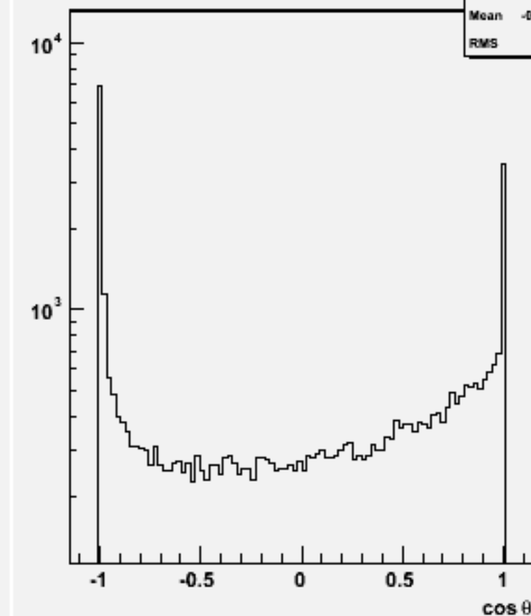
Jet cos \theta (All jets)w100911 e3e3n1e1sc_o
