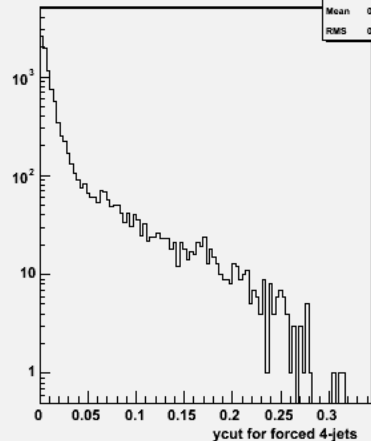
Ycut for 4-jets :w100909 e3e3n1e1du_o
