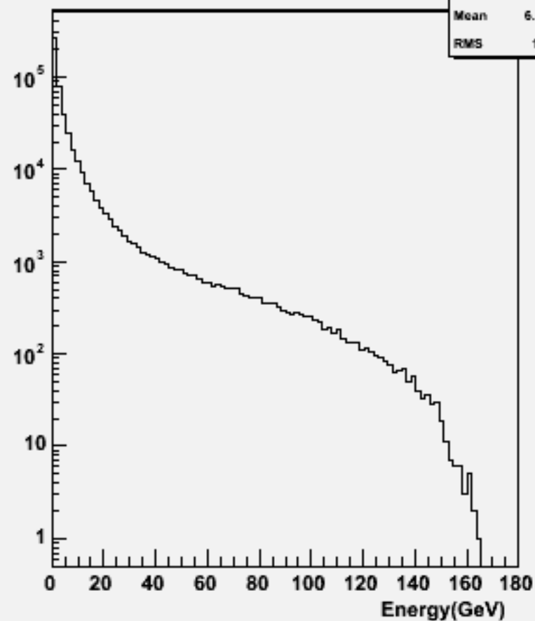
Start point R : w100909 e3e3n1e1du_o
