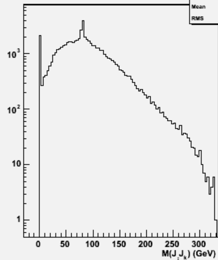
2jets mass(All comb)w100909 e3e3n1e1du_o
