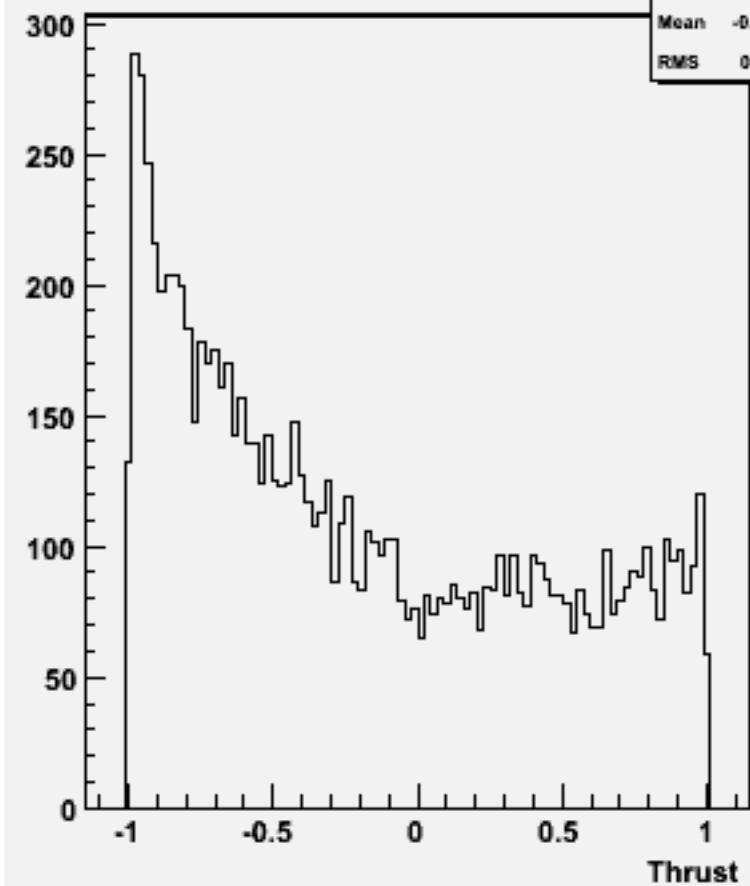
cos \Theta (thrust) w100909 e3e3n1e1du_o
