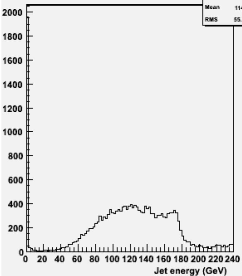
energy for 2-jets :w100909 e3e3n1e1du_o
