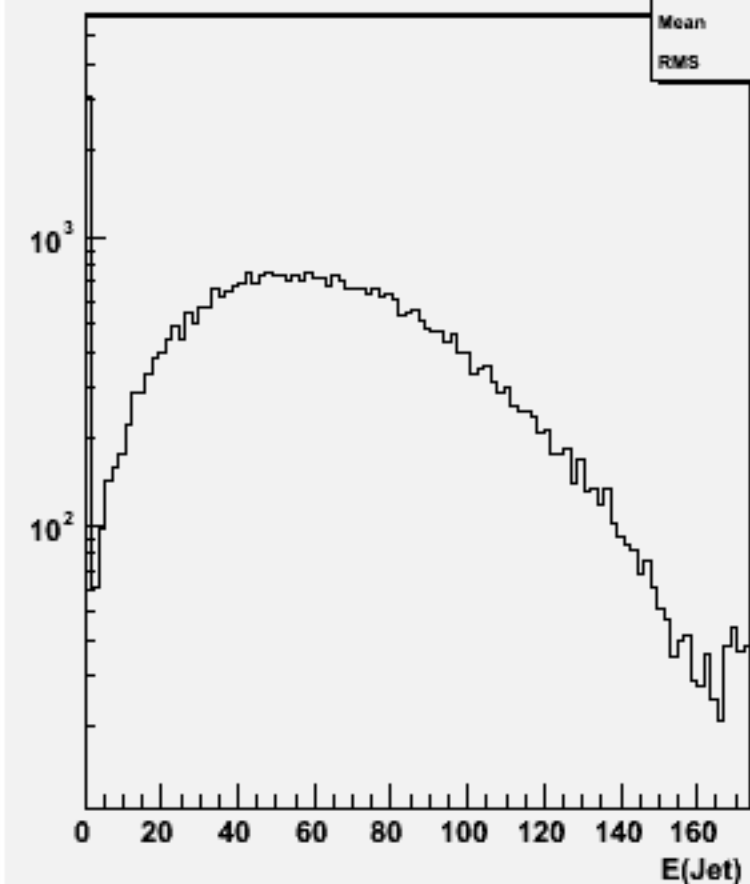
Jet energies(All jets)w100909 e3e3n1e1du_o
