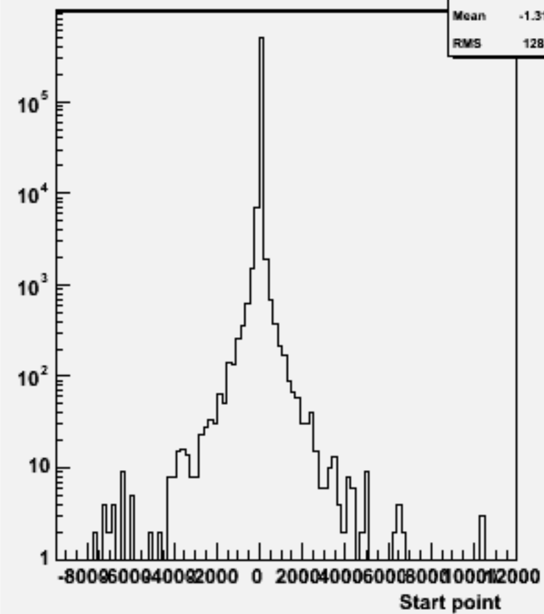
Start point Z : w100909 e3e3n1e1du_o
