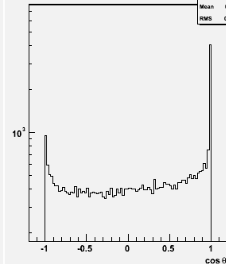
Jet cos \theta (All jets)w100909 e3e3n1e1du_o
