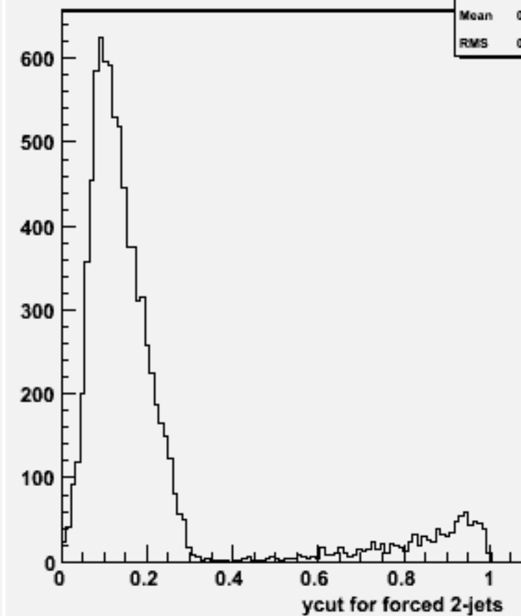
Ycut for 2-jets :w100909 e3e3n1e1du_o
