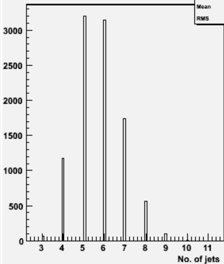
No. jets (ycut=0.001) : w100909 e3e3n1e1du_o
