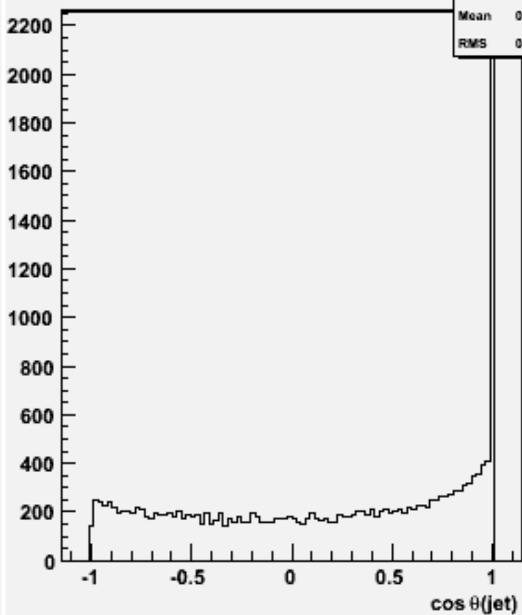
cos \theta for 2-jets :w100909 e3e3n1e1du_o
