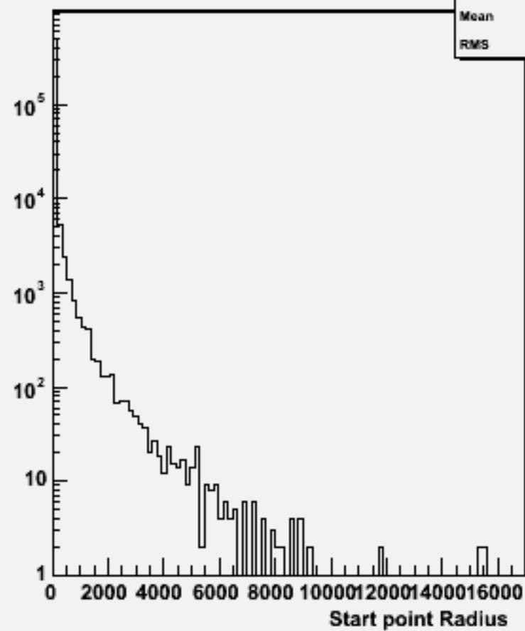
Start point R : w100909 e3e3n1e1du_o
