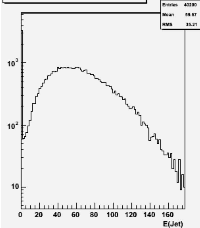
Jet energies(All jets)w100908 e3e3n1e1du_o
