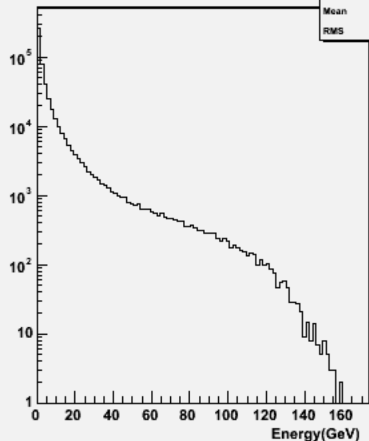
Particle Energy : w100908 e3e3n1e1du_o
