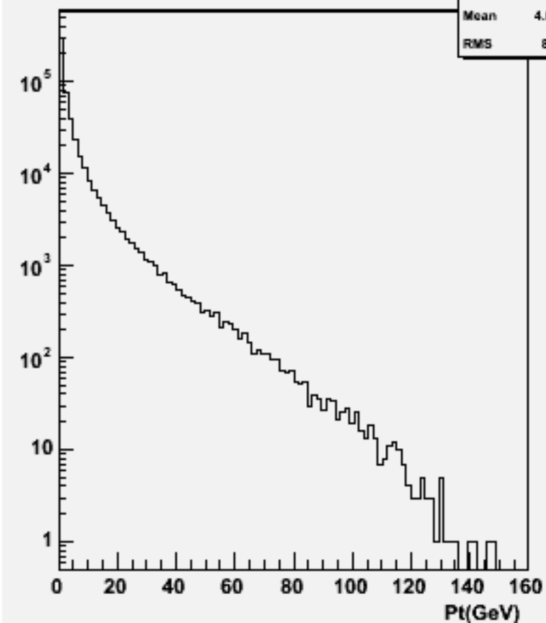
Particle Pt : w100908 e3e3n1e1du_o
