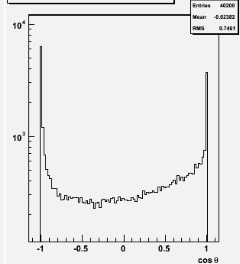
Jet cos \theta (All jets)w100908 e3e3n1e1du_o
