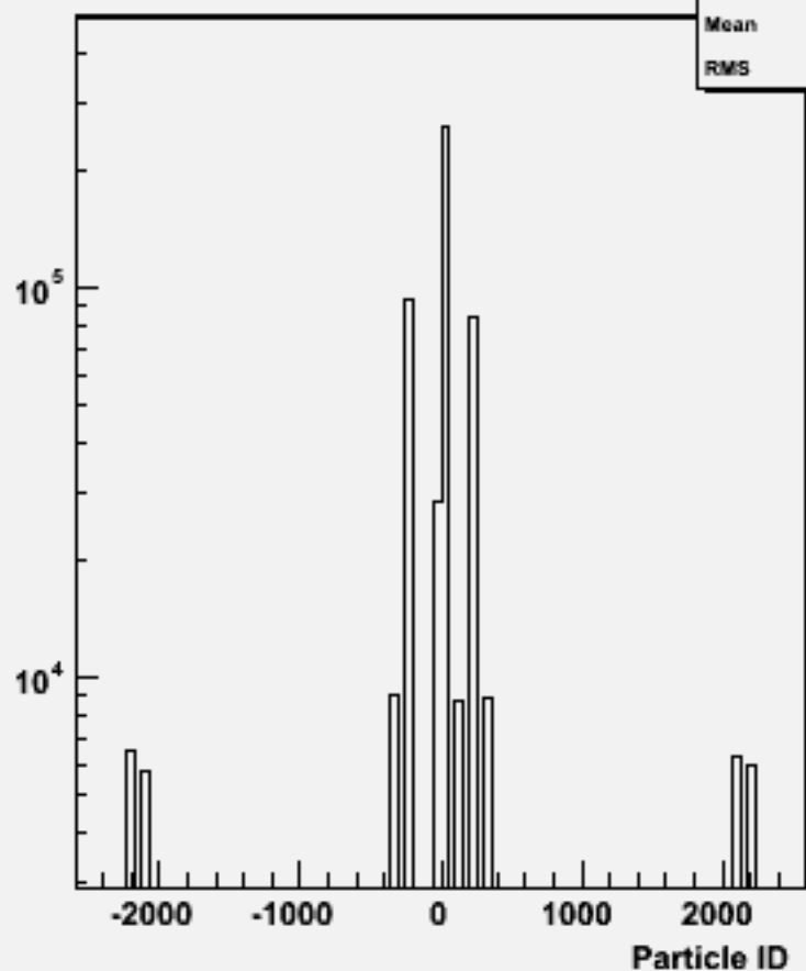
Particle ID : w100908 e3e3n1e1du_o
