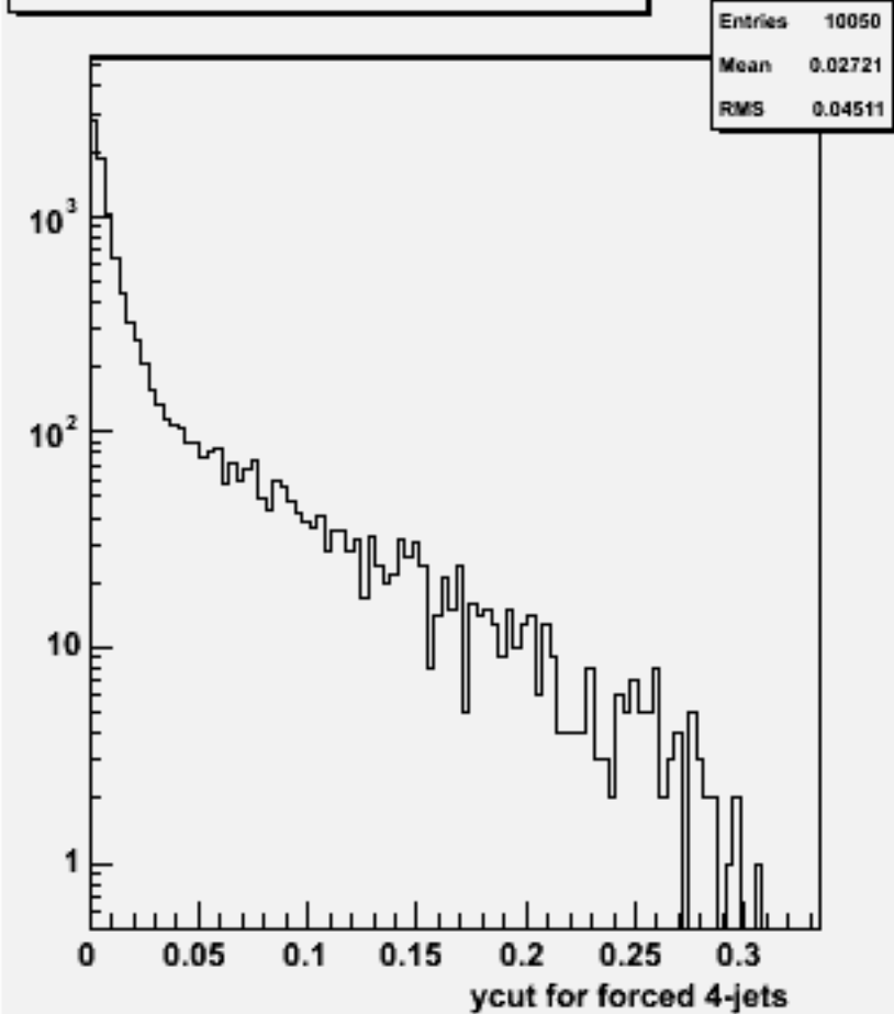
Ycut for 4-jets :w100908 e3e3n1e1du_o
