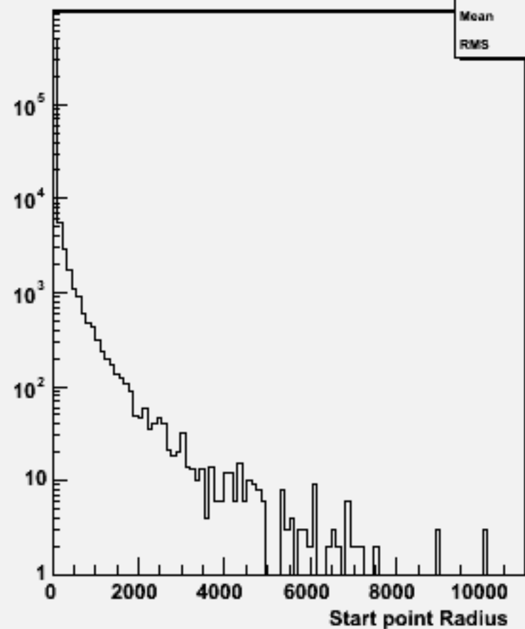
Start point R : w100908 e3e3n1e1du_o
