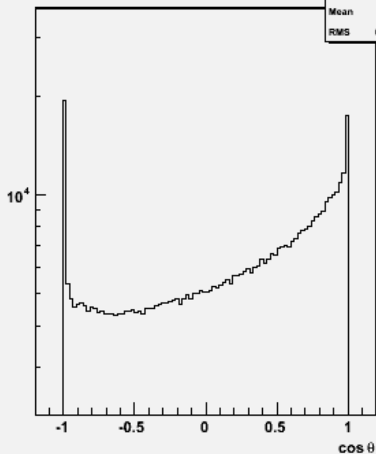
Particle \cos\theta : w100908 e3e3n1e1du_o
