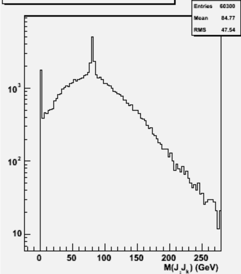
2jets mass(All comb)w100908 e3e3n1e1du_o
