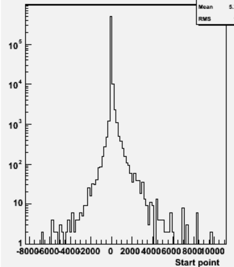
Start point Z : w100908 e3e3n1e1du_o
