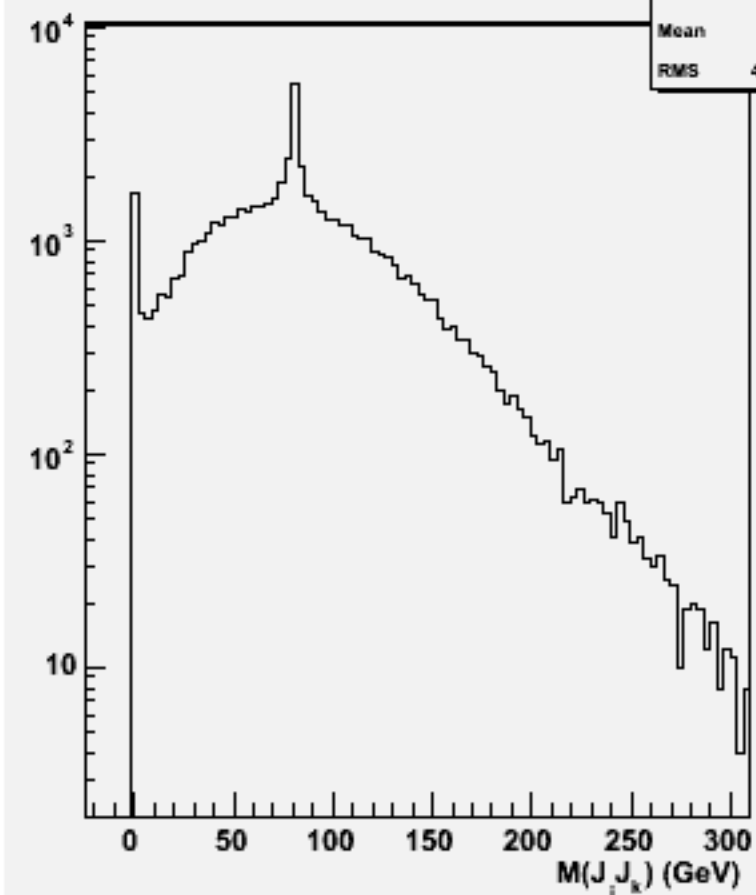
2jets mass(All comb)w100907 e3e3n1e1du_o
