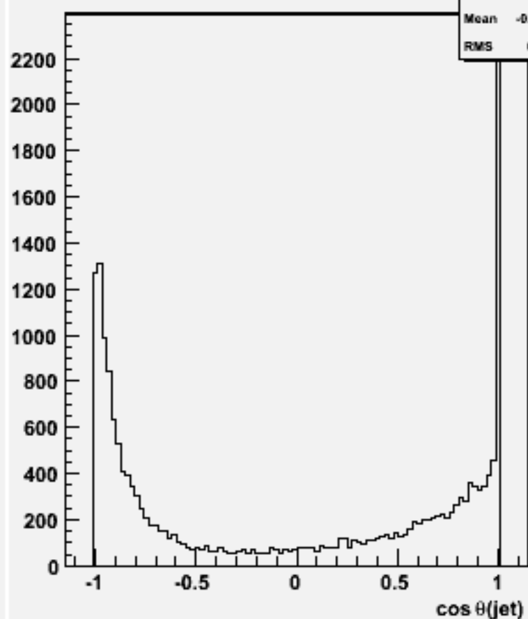
cos \theta for 2-jets :w100907 e3e3n1e1du_o
