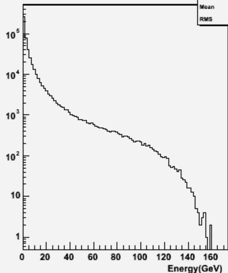
Particle Energy : w100907 e3e3n1e1du_o
