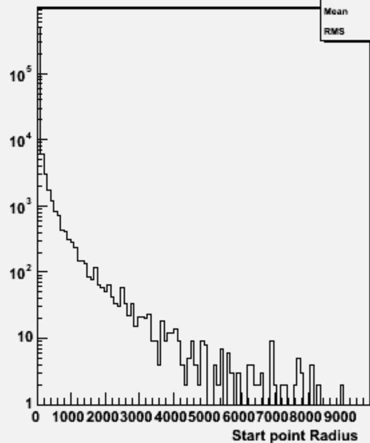
Start point R : w100907 e3e3n1e1du_o
