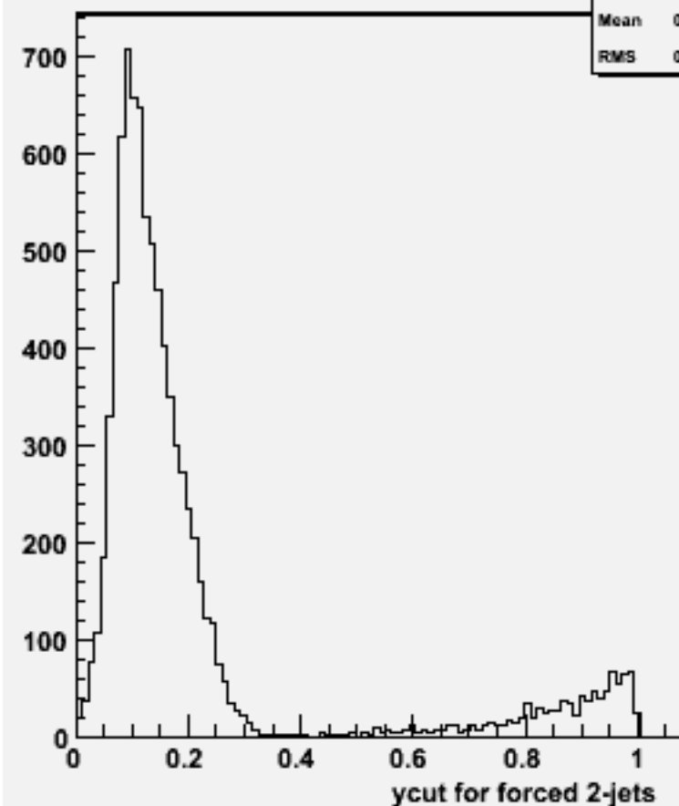
Ycut for 2-jets :w100907 e3e3n1e1du_o
