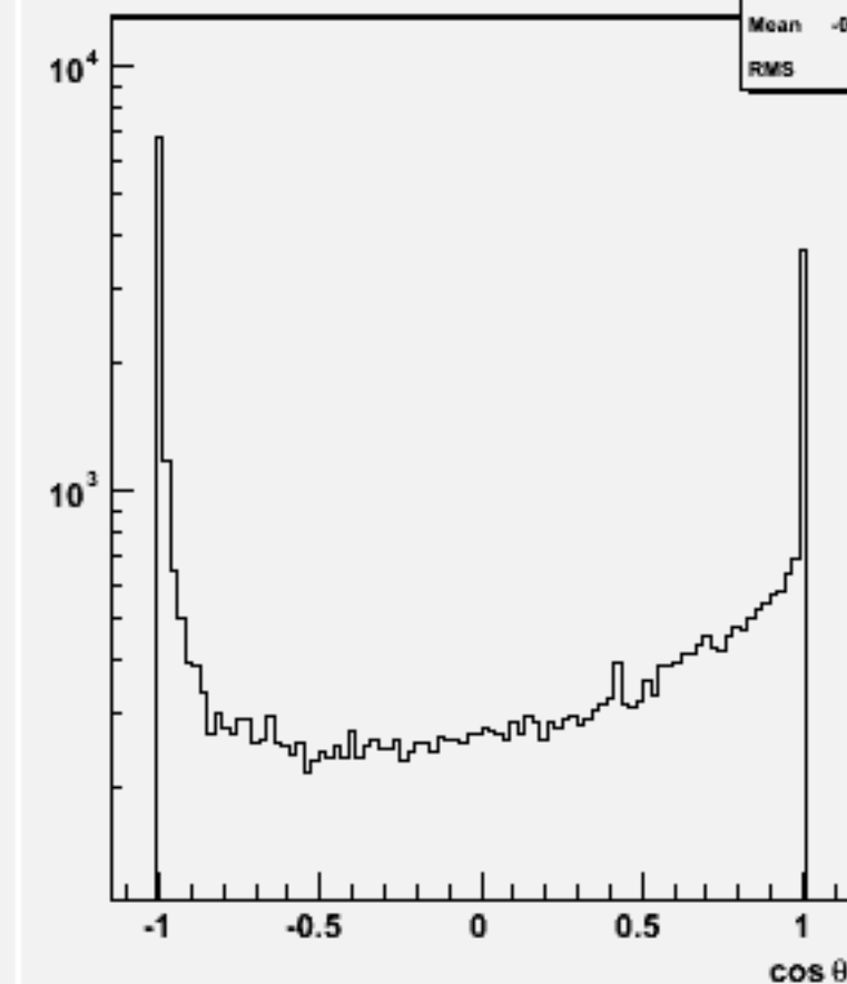
Jet cos \theta (All jets)w100907 e3e3n1e1du_o
