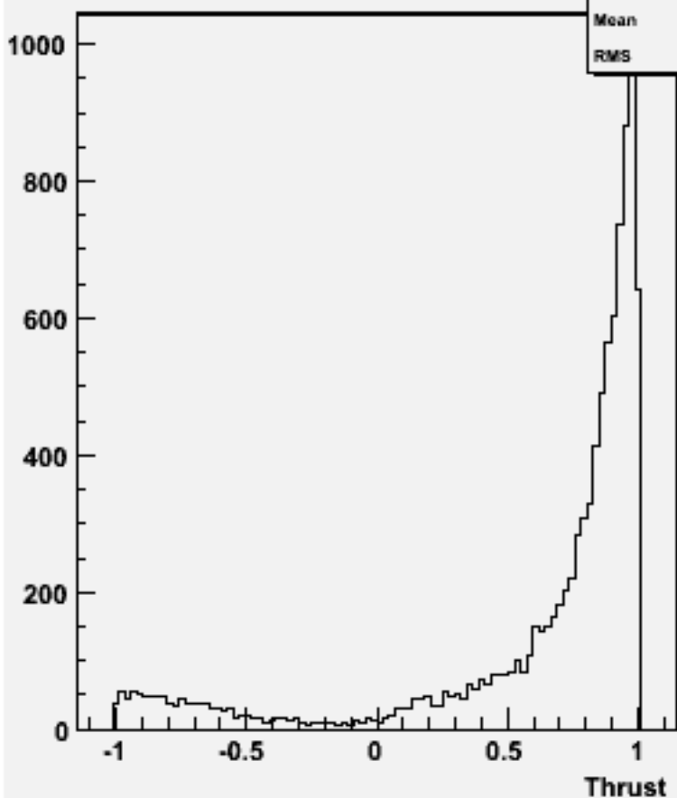
cos \Theta (thrust) w100907 e3e3n1e1du_o
