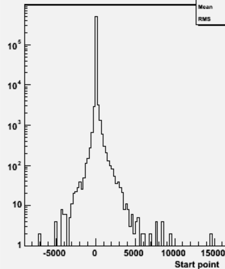
Start point Z : w100907 e3e3n1e1du_o
