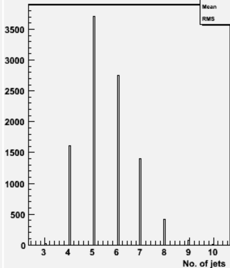
No. jets (ycut=0.001) : w100907 e3e3n1e1du_o
