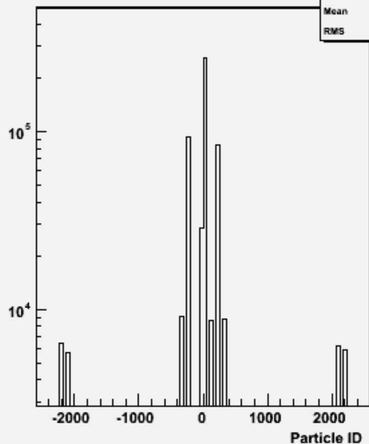
Particle ID : w100907 e3e3n1e1du_o
