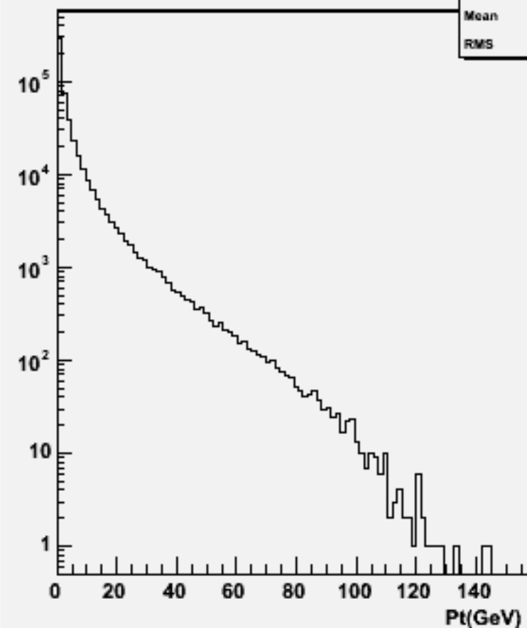
Particle Pt : w100907 e3e3n1e1du_o
