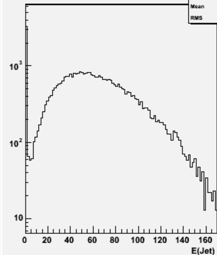
Jet energies(All jets)w100907 e3e3n1e1du_o
