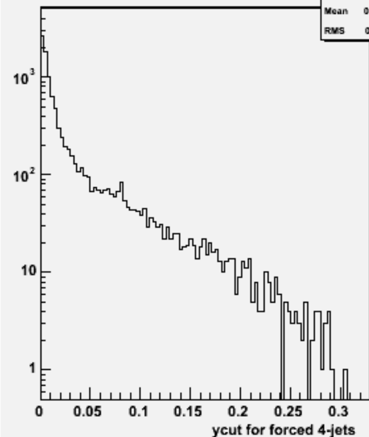
Ycut for 4-jets :w100907 e3e3n1e1du_o
