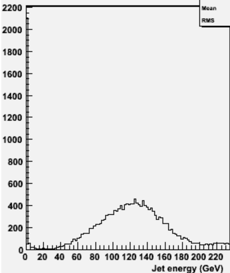
energy for 2-jets :w100907 e3e3n1e1du_o
