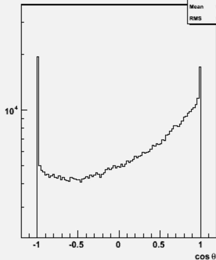
Particle cos \theta : w100907 e3e3n1e1du_o
