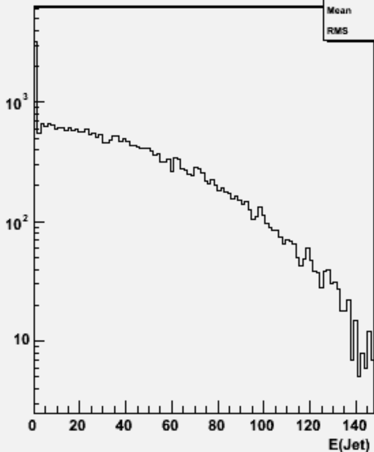
Jet energies(All jets)w100905 e3e3n1e1e3n3_o
