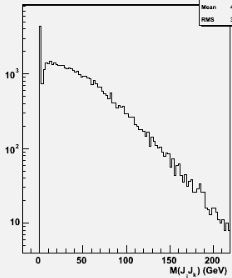
2jets mass(All comb)w100905 e3e3n1e1e3n3_o
