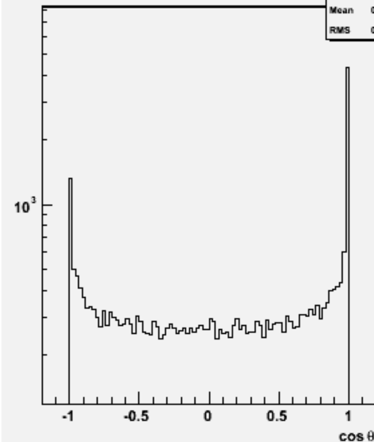
Jet cos \theta (All jets)w100905 e3e3n1e1e3n3_o
