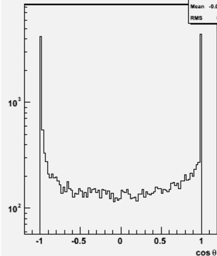
Jet cos \theta (All jets)w100904 e3e3n1e1e3n3_o
