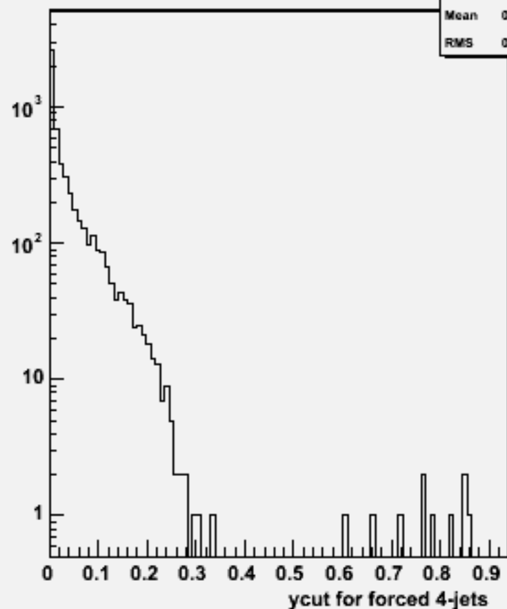
Ycut for 4-jets :w100904 e3e3n1e1e3n3_o
