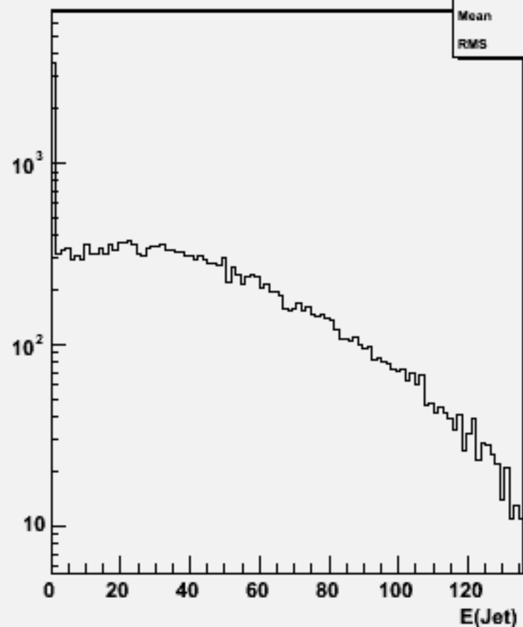
Jet energies(All jets)w100904 e3e3n1e1e3n3_o
