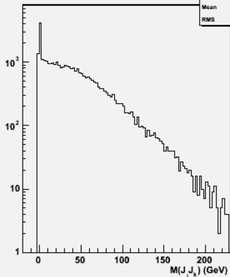
2jets mass(All comb)w100904 e3e3n1e1e3n3_o
