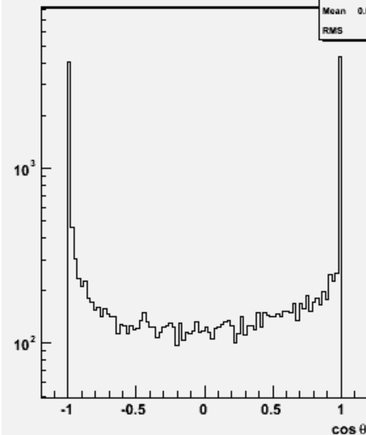
Jet cos \theta (All jets)w100899 e3e3n1e1e2n2_o
