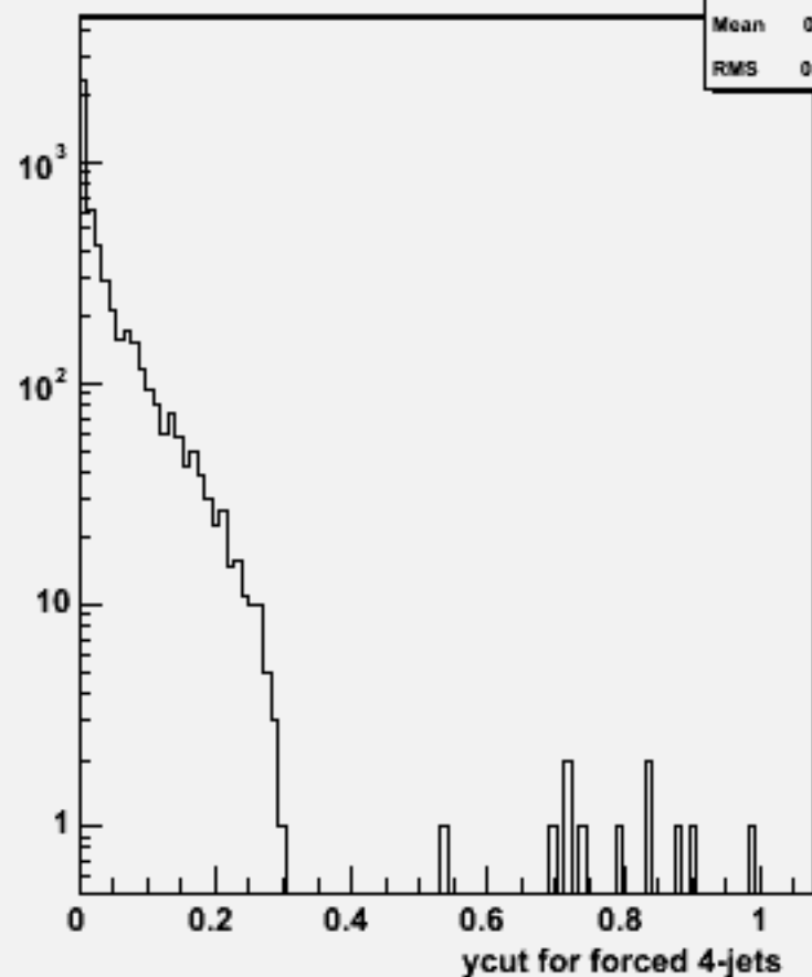
Ycut for 4-jets :w100899 e3e3n1e1e2n2_o
