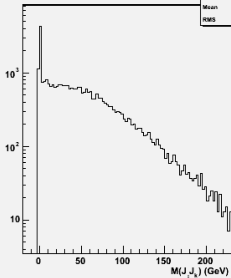
2jets mass(All comb)w100899 e3e3n1e1e2n2_o
