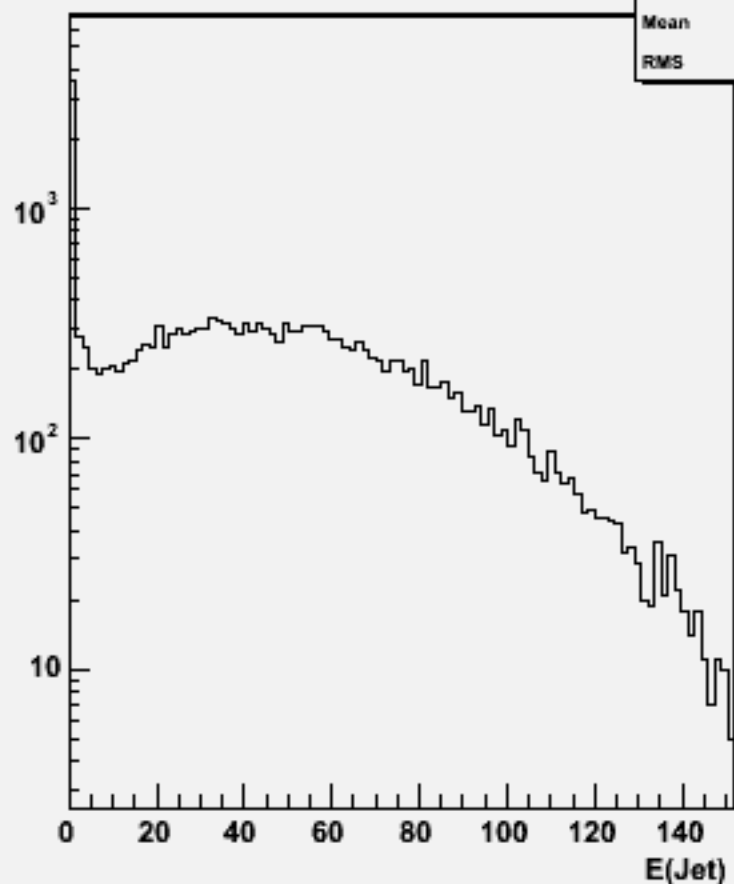
Jet energies(All jets)w100899 e3e3n1e1e2n2_o
