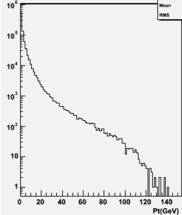
Particle Pt : w100893 e2e2cssc_o
