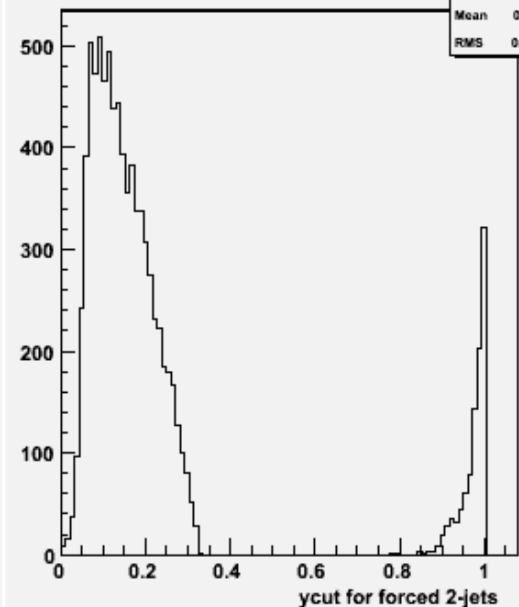
Ycut for 2-jets :w100893 e2e2cssc_o
