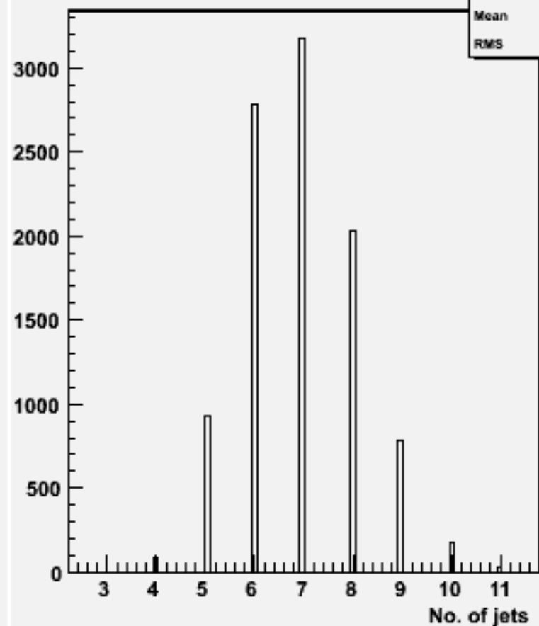
No. jets (ycut=0.001) : w100893 e2e2cssc_o
