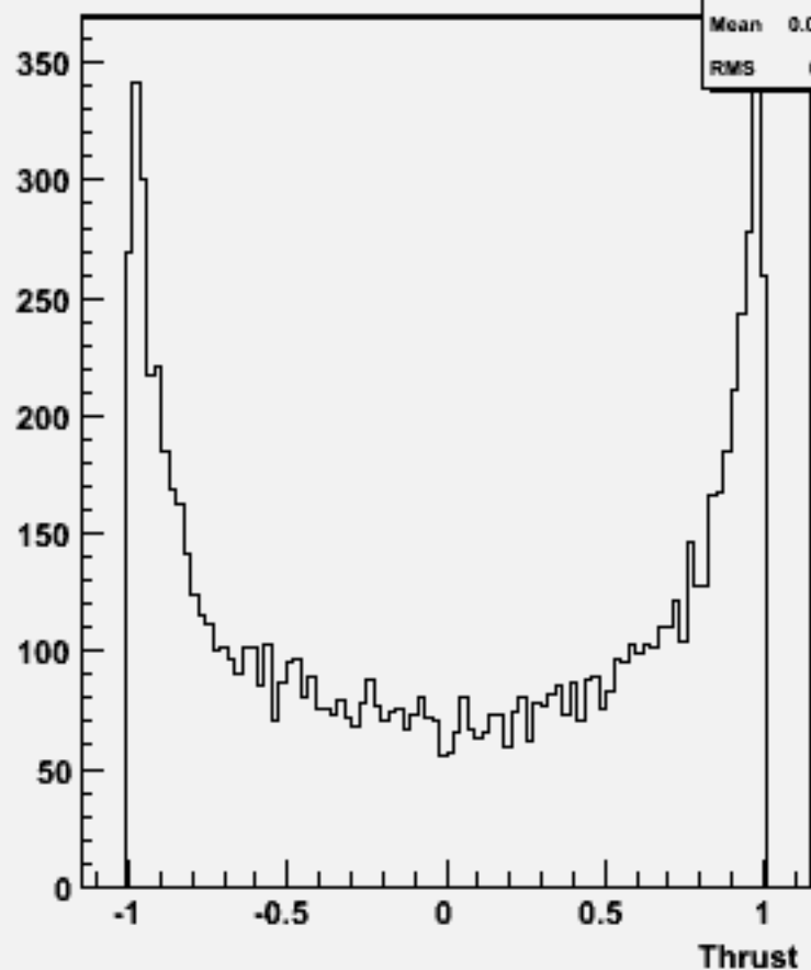
cos \Theta (thrust) w100893 e2e2cssc_o
