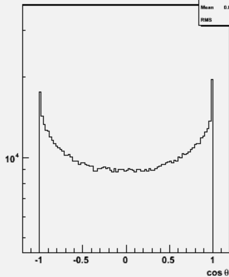
Particle cosθ : w100893 e2e2cssc_o
