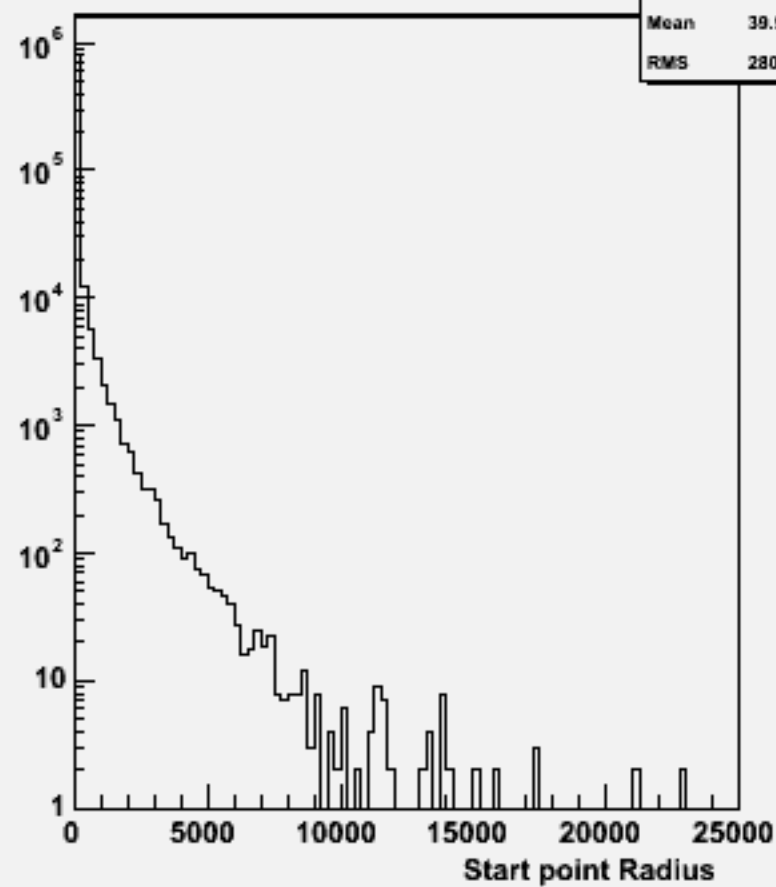
Start point R : w100893 e2e2cssc_o
