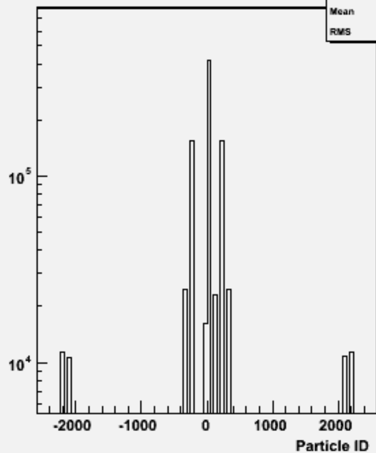
Particle ID : w100893 e2e2cssc_o
