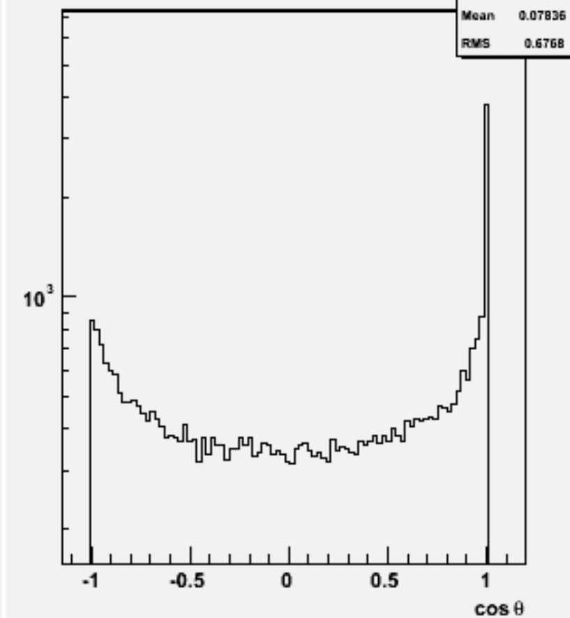
Jet cosθ (All jets)w100893 e2e2cssc_o
