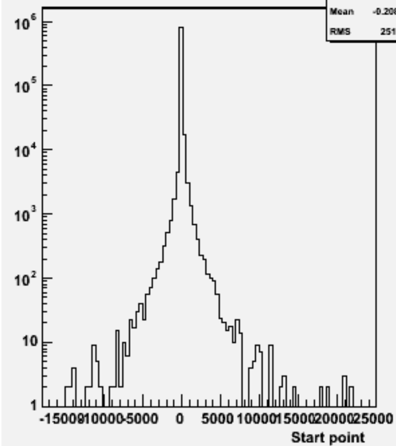
Start point Z : w100893 e2e2cssc_o
