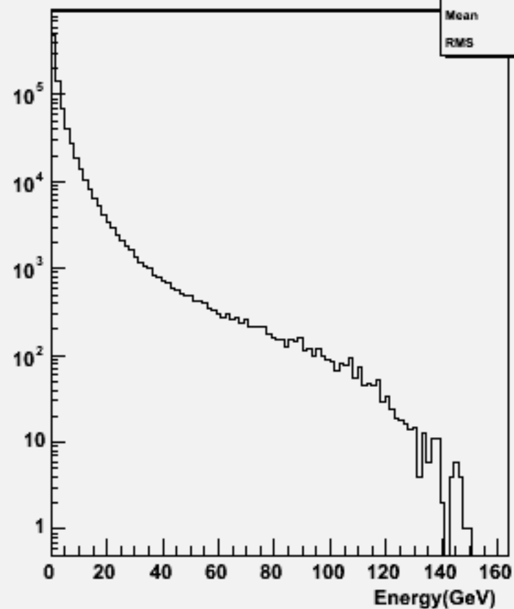
Particle Energy : w100893 e2e2cssc_o
