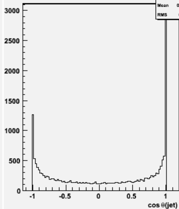
cos \theta for 2-jets :w100893 e2e2cssc_o
