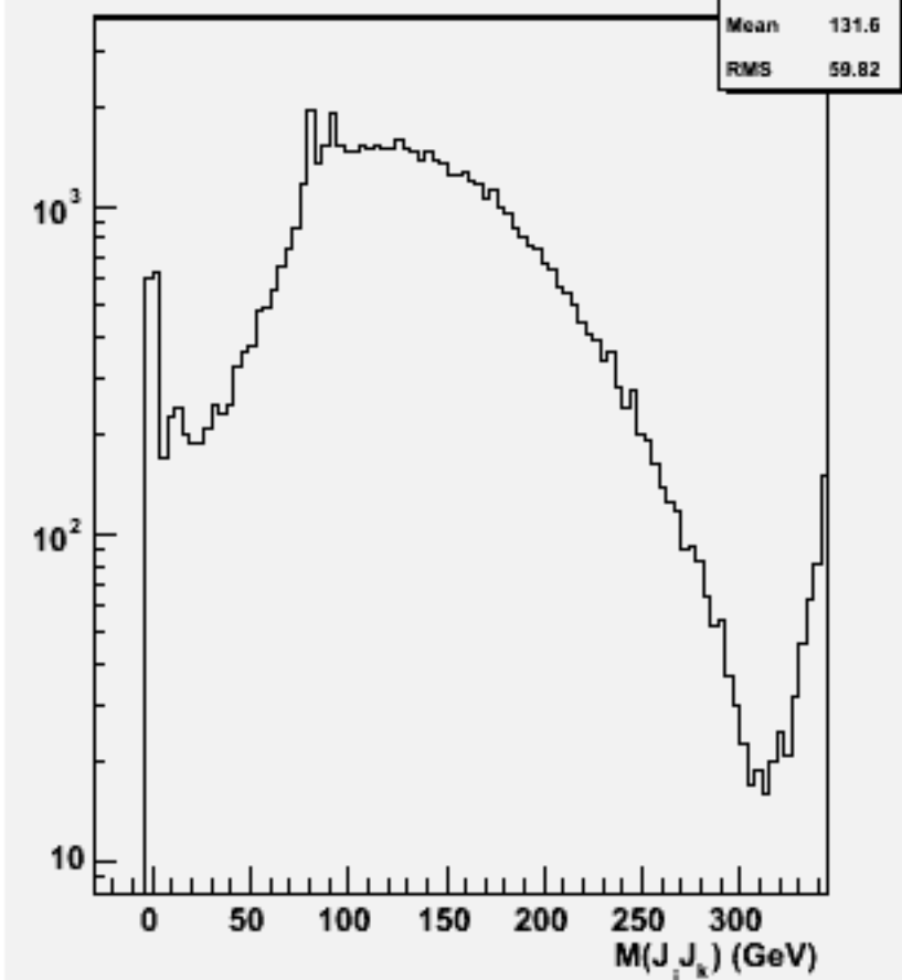
2jets mass(All comb)w100893 e2e2cssc_o
