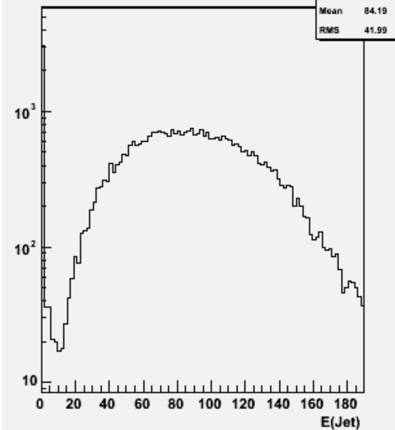
Jet energies(All jets)w100893 e2e2cssc_o
