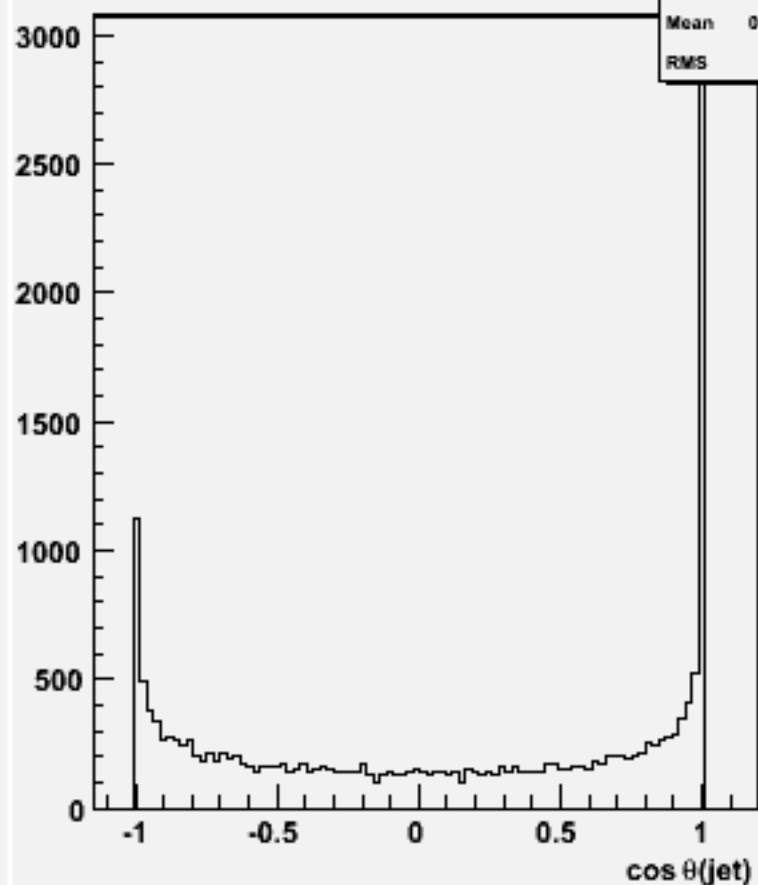
cos \theta for 2-jets :w100892 e2e2cssc_o
