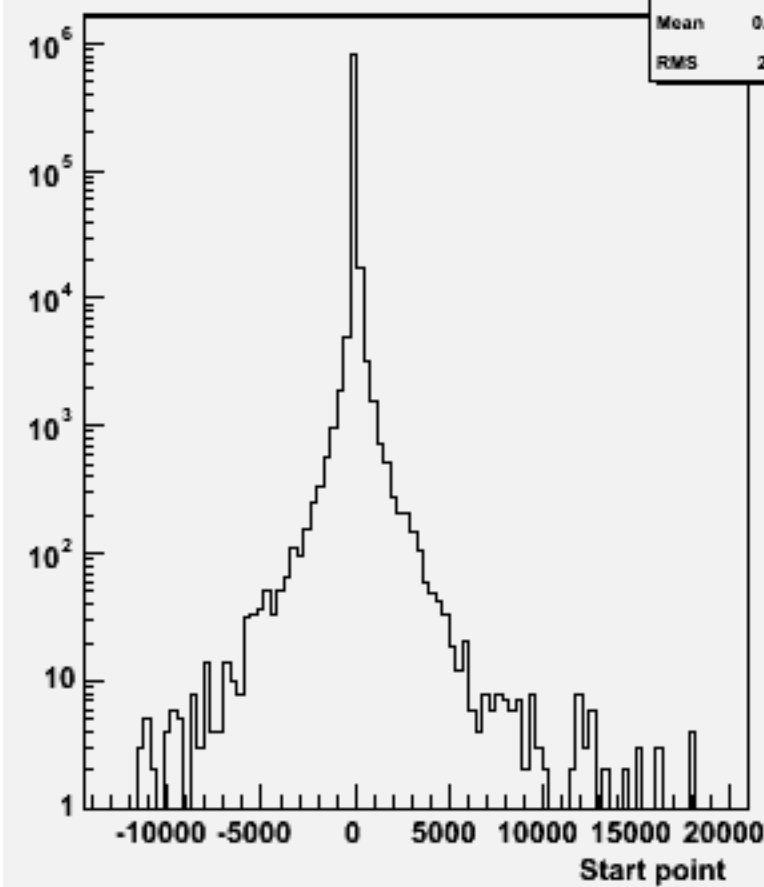
Start point Z : w100892 e2e2cssc_o
