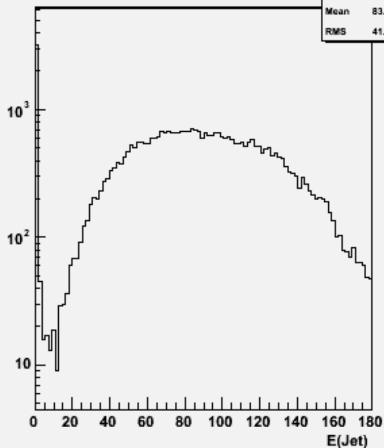
Jet energies(All jets)w100892 e2e2cssc_o
