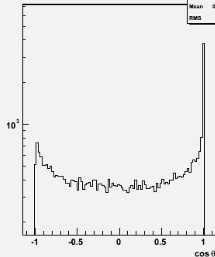
Jet cosθ (All jets)w100892 e2e2cssc_o
