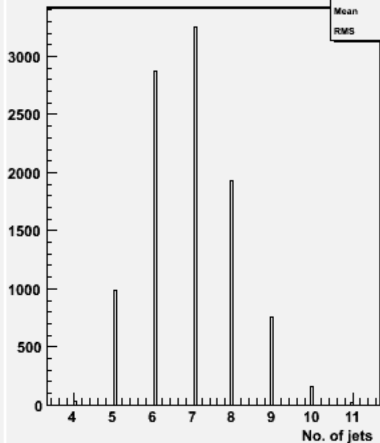
No. jets (ycut=0.001) : w100892 e2e2cssc_o
