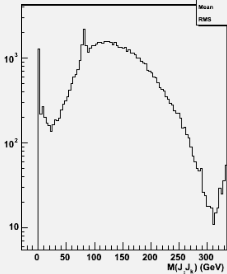
2jets mass(All comb)w100892 e2e2cssc_o
