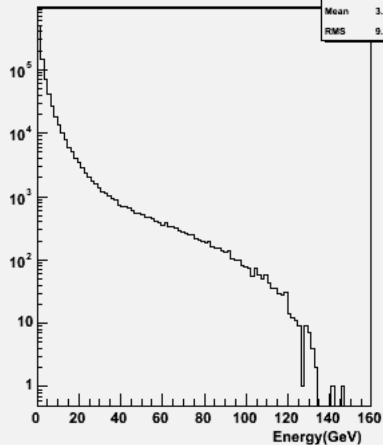
Start point R : w100892 e2e2cssc_o
