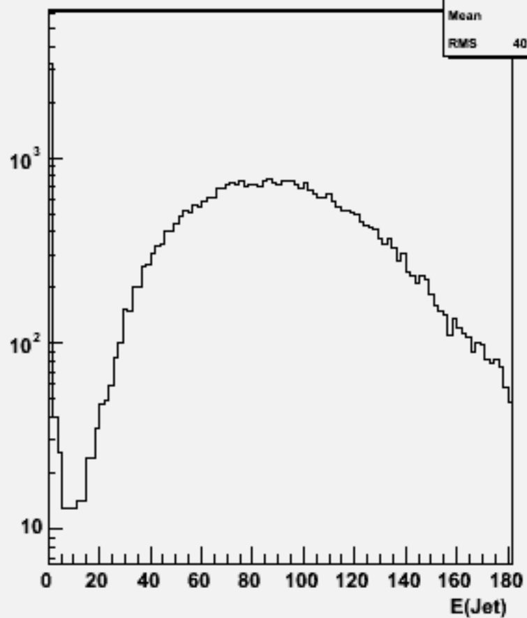
Jet energies(All jets)w100889 e2e2csdu_o
