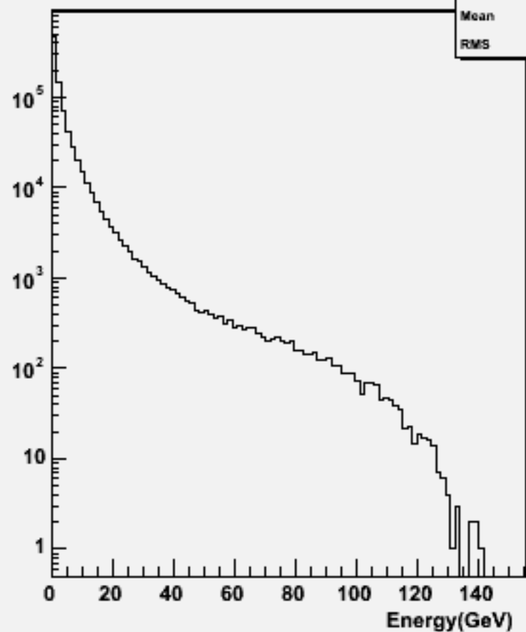
Particle Energy : w100889 e2e2csdu_o
