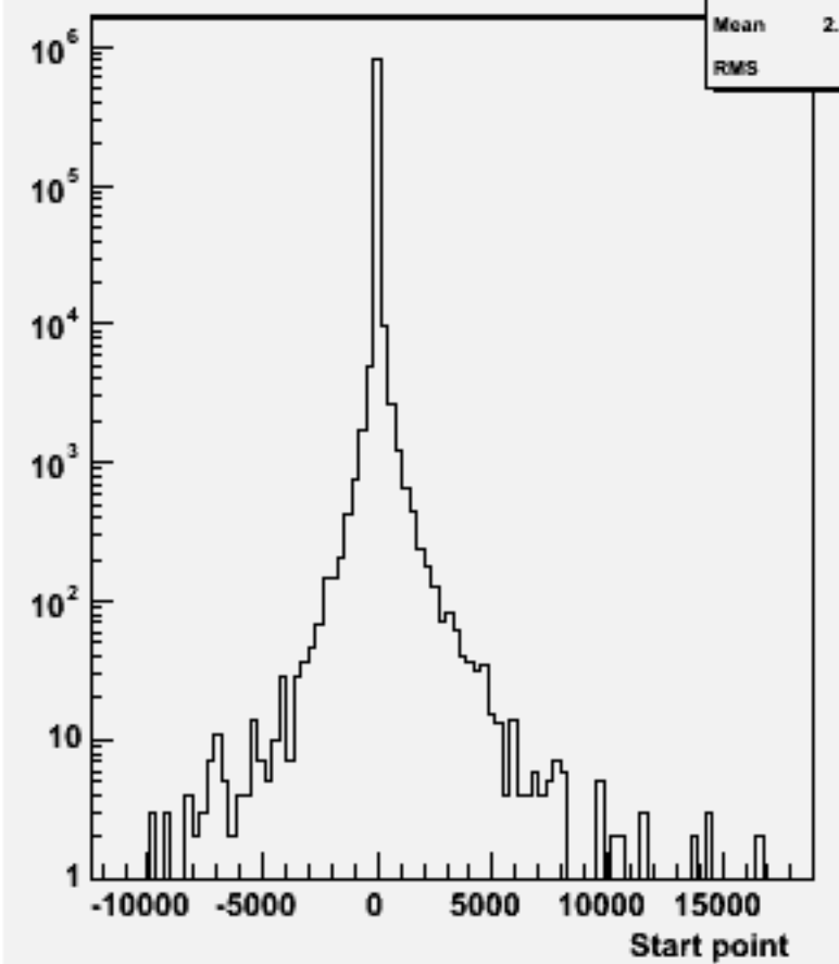
Start point Z : w100889 e2e2csdu_o
