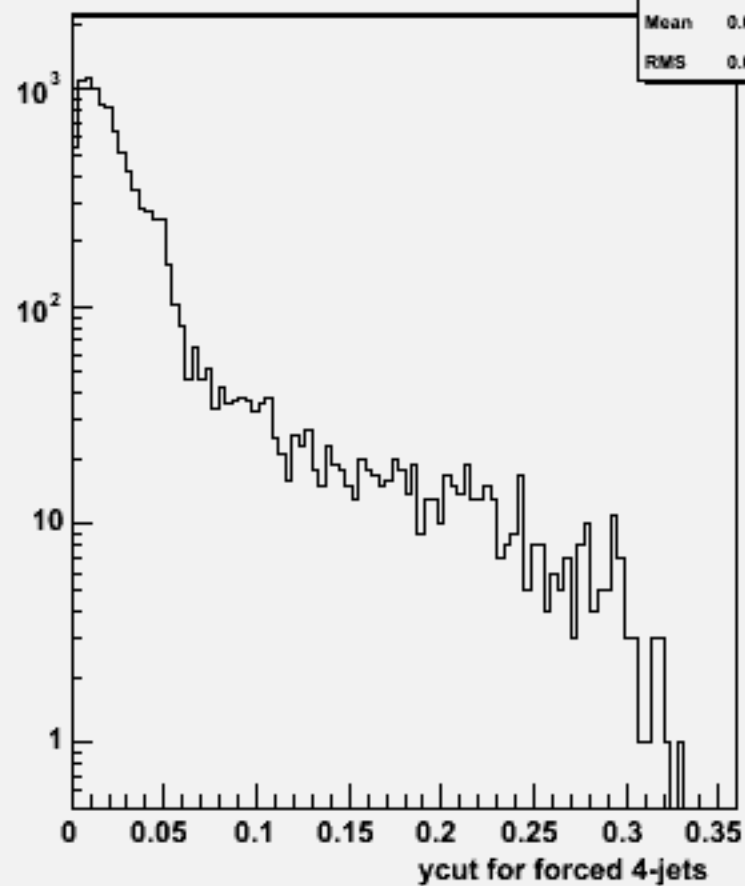
Ycut for 4-jets :w100889 e2e2csdu_o
