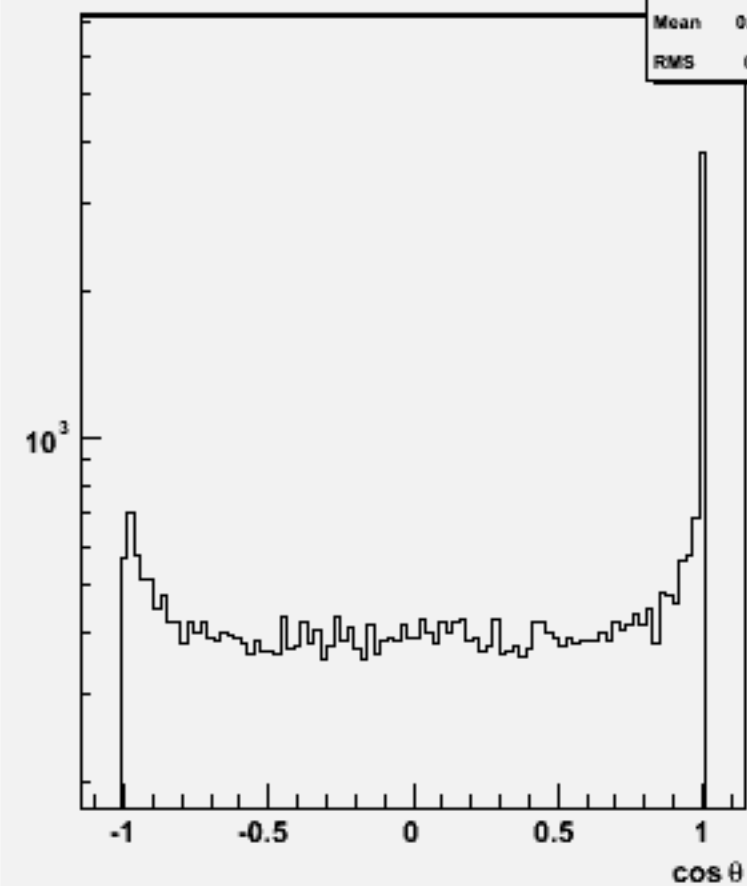
Jet cosθ (All jets)w100889 e2e2csdu_o
