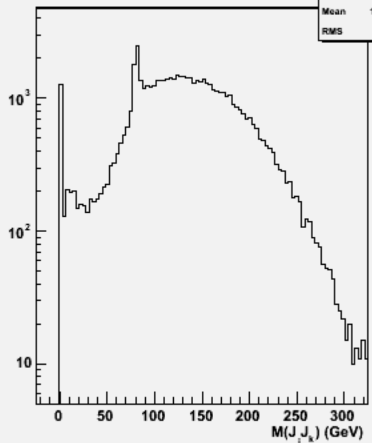
2jets mass(All comb)w100889 e2e2csdu_o
