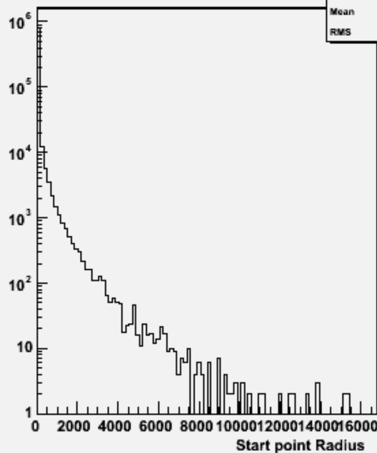
Start point R : w100888 e2e2csdu_o
