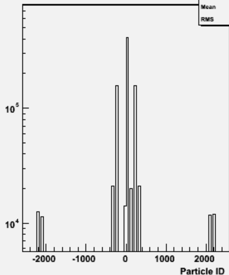
Particle ID : w100888 e2e2csdu_o
