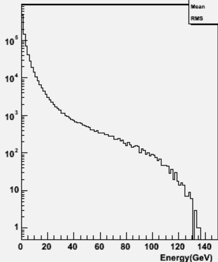
Particle Energy : w100888 e2e2csdu_o
