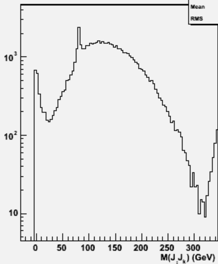
2jets mass(All comb)w100888 e2e2csdu_o
