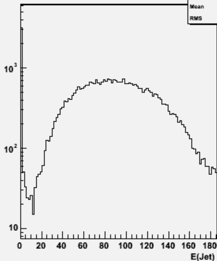
Jet energies(All jets)w100888 e2e2csdu_o
