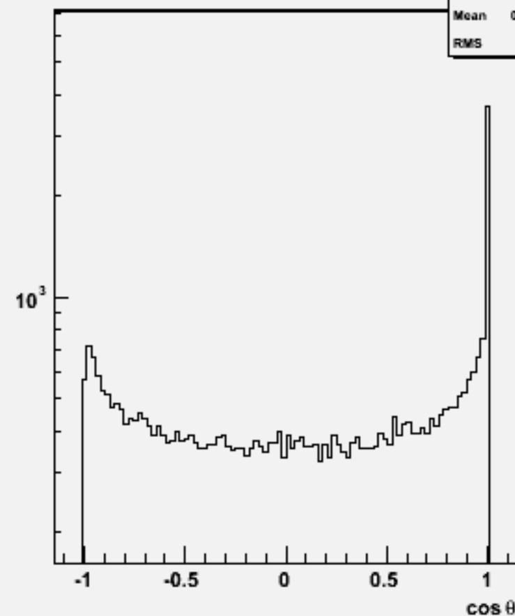
Jet cosθ (All jets)w100888 e2e2csdu_o
