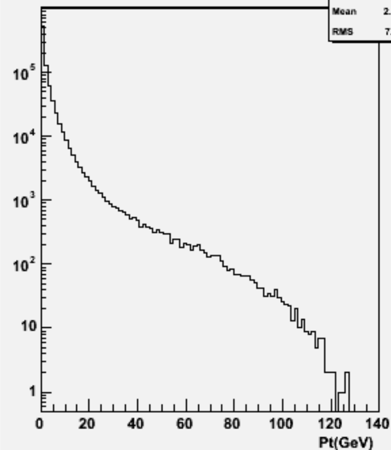
Particle Pt : w100888 e2e2csdu_o
