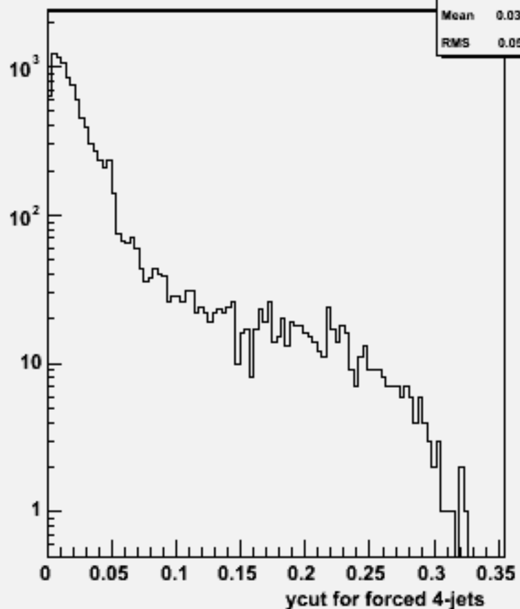
Ycut for 4-jets :w100888 e2e2csdu_o
