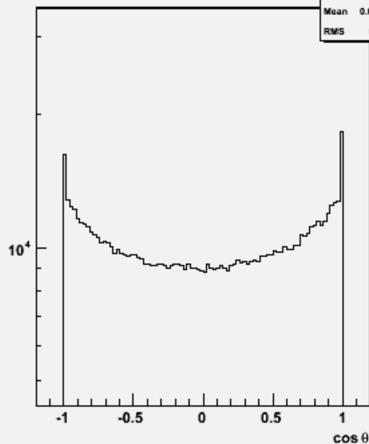
Particle cos \theta : w100888 e2e2csdu_o
