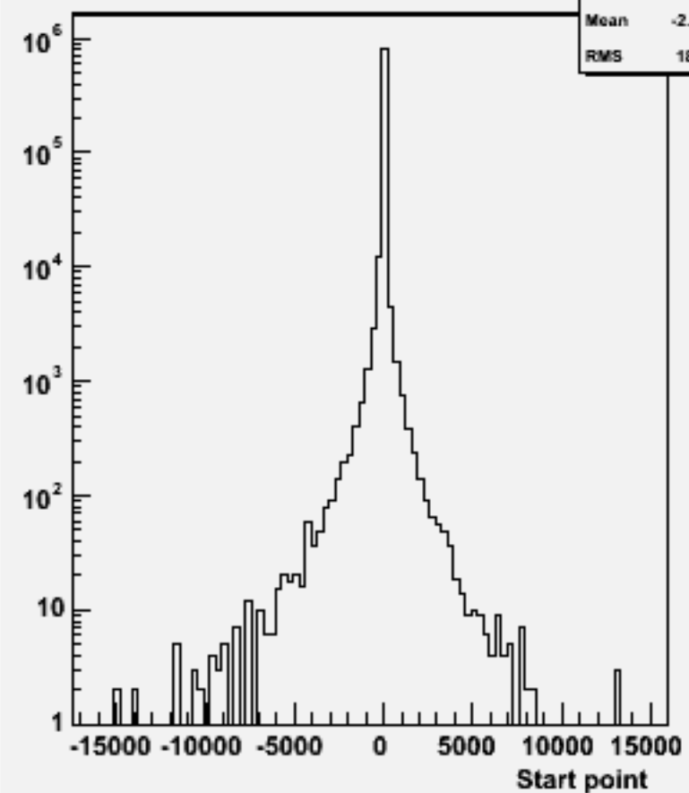
Start point Z : w100888 e2e2csdu_o
