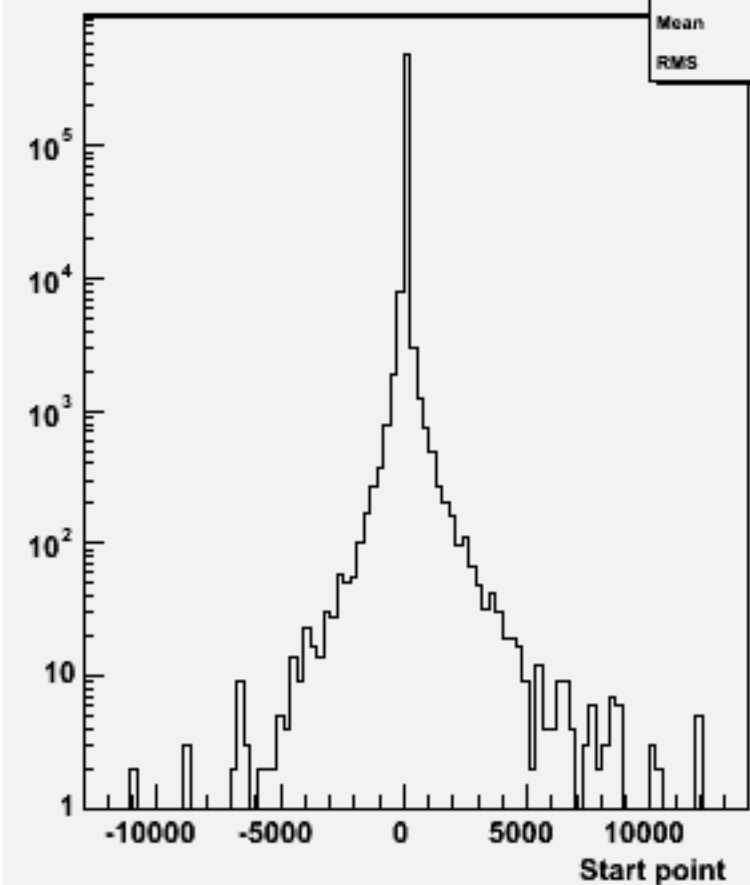
Start point Z : w100885 e2e2cse3n3_o
