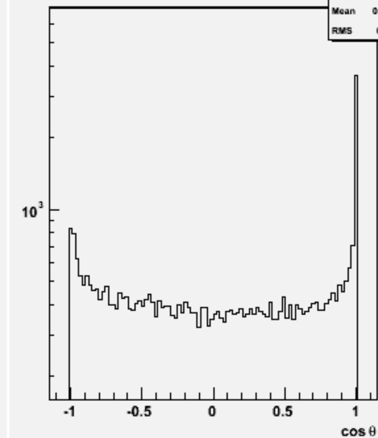
Jet cos \theta (All jets)w100885 e2e2cse3n3_o
