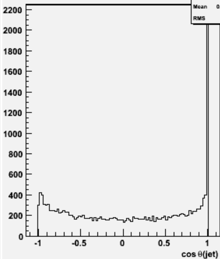
cos \theta for 2-jets :w100885 e2e2cse3n3_o
