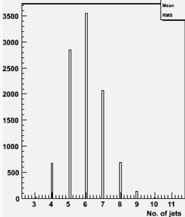
No. jets (ycut=0.001) : w100885 e2e2cse3n3_o
