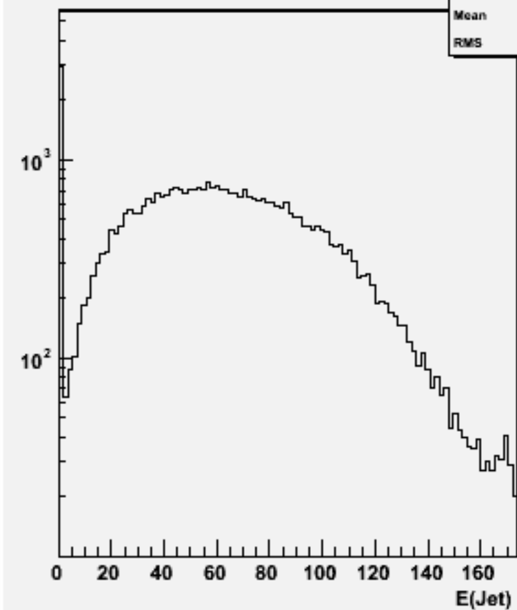
Jet energies(All jets)w100885 e2e2cse3n3_o
