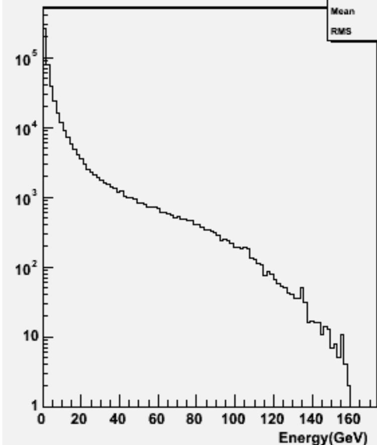
Particle Energy : w100885 e2e2cse3n3_o
