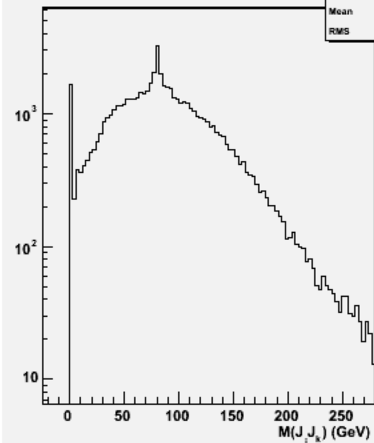
2jets mass(All comb)w100885 e2e2cse3n3_o
