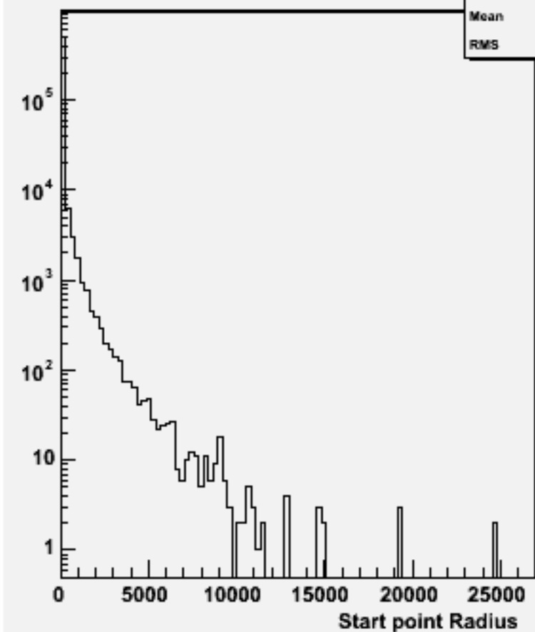
Start point R : w100885 e2e2cse3n3_o
