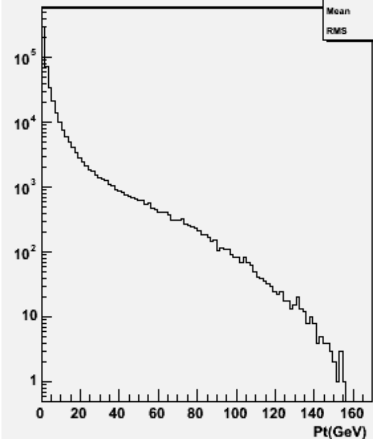
Particle Pt : w100885 e2e2cse3n3_o
