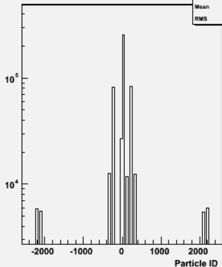
Particle ID : w100885 e2e2cse3n3_o
