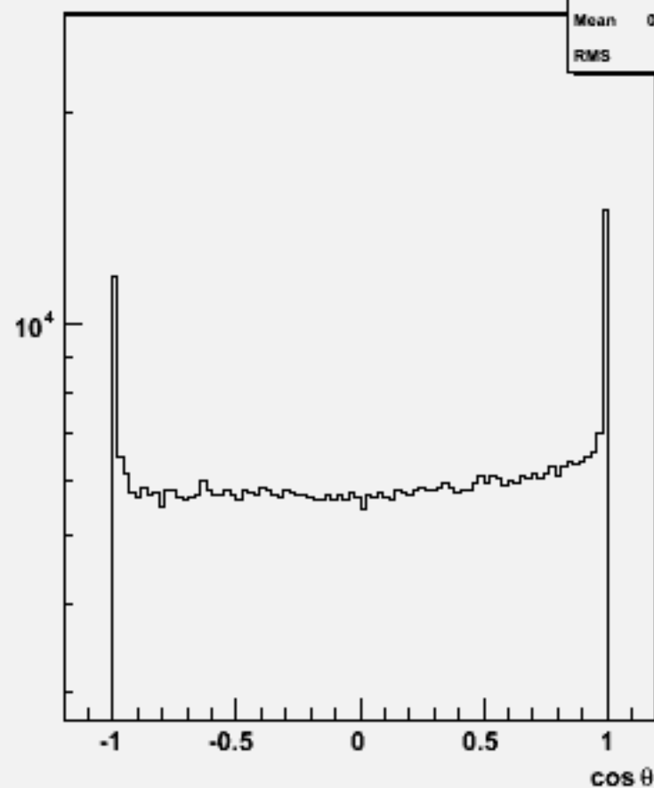
Particle cosθ : w100885 e2e2cse3n3_o
