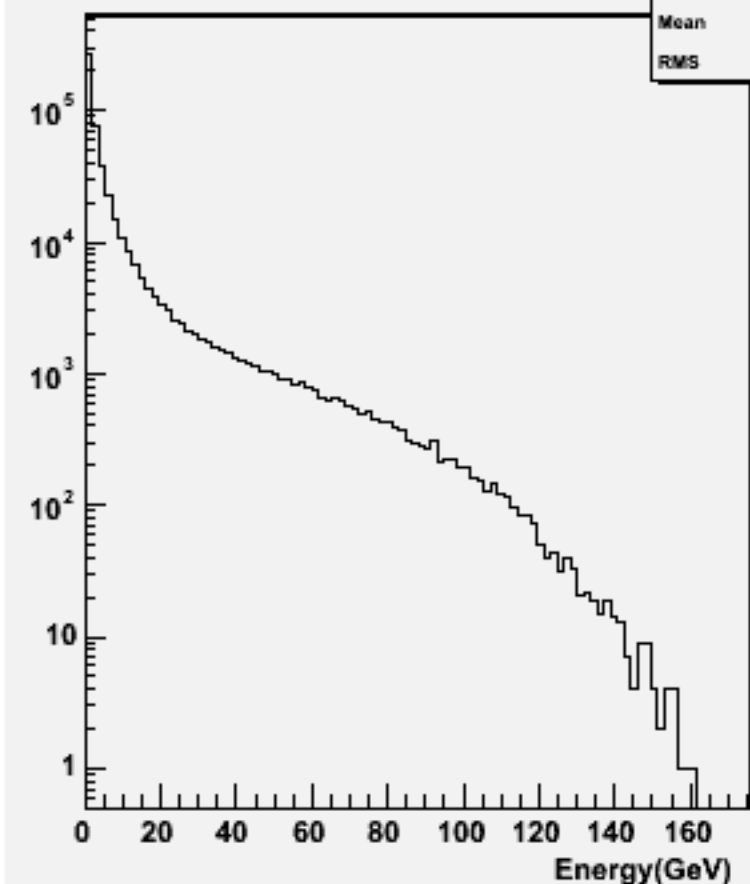
Particle Energy : w100884 e2e2cse3n3_o
