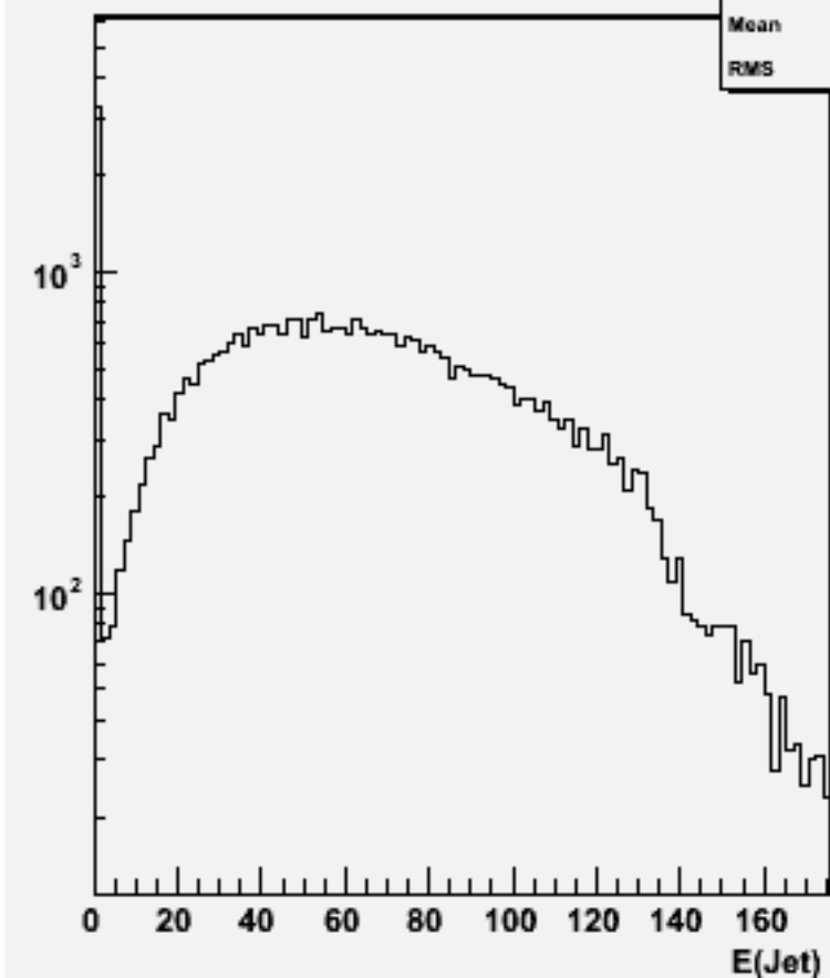
Jet energies(All jets)w100884 e2e2cse3n3_o
