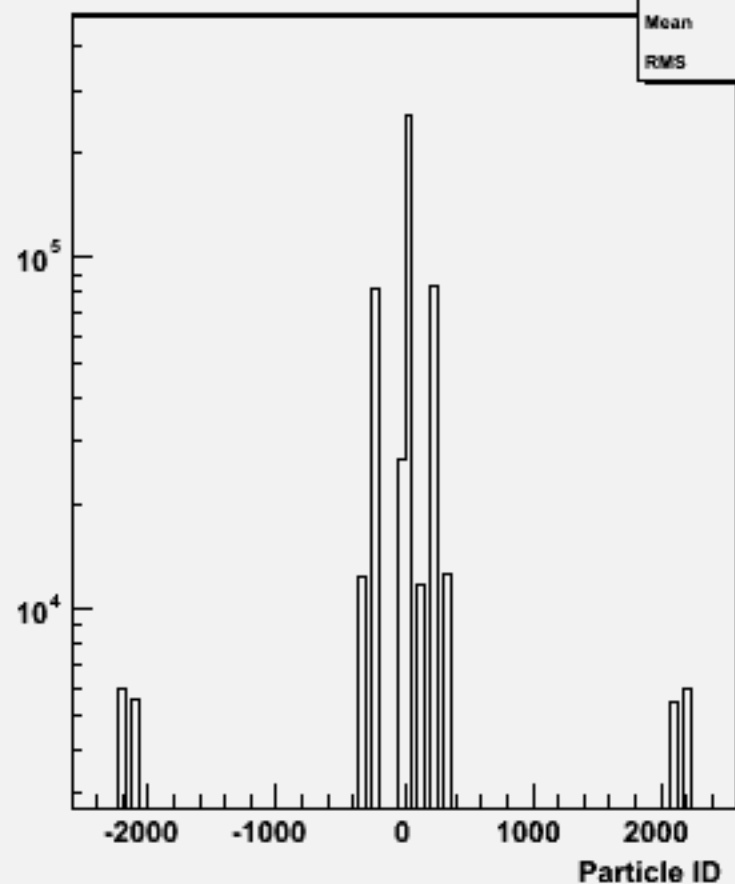
Particle ID : w100884 e2e2cse3n3_o
