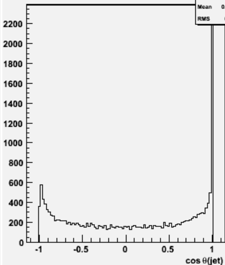
cos \theta for 2-jets :w100884 e2e2cse3n3_o
