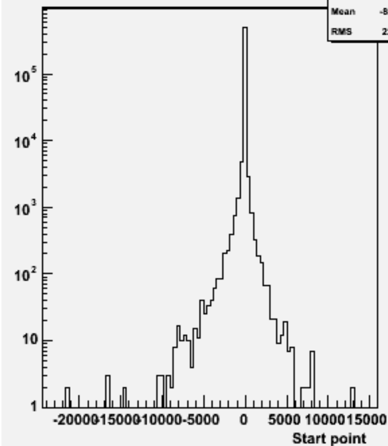
Start point Z : w100884 e2e2cse3n3_o
