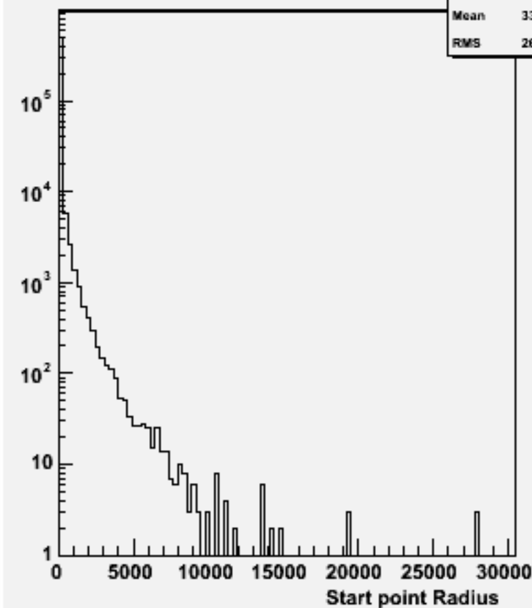
Start point R : w100884 e2e2cse3n3_o
