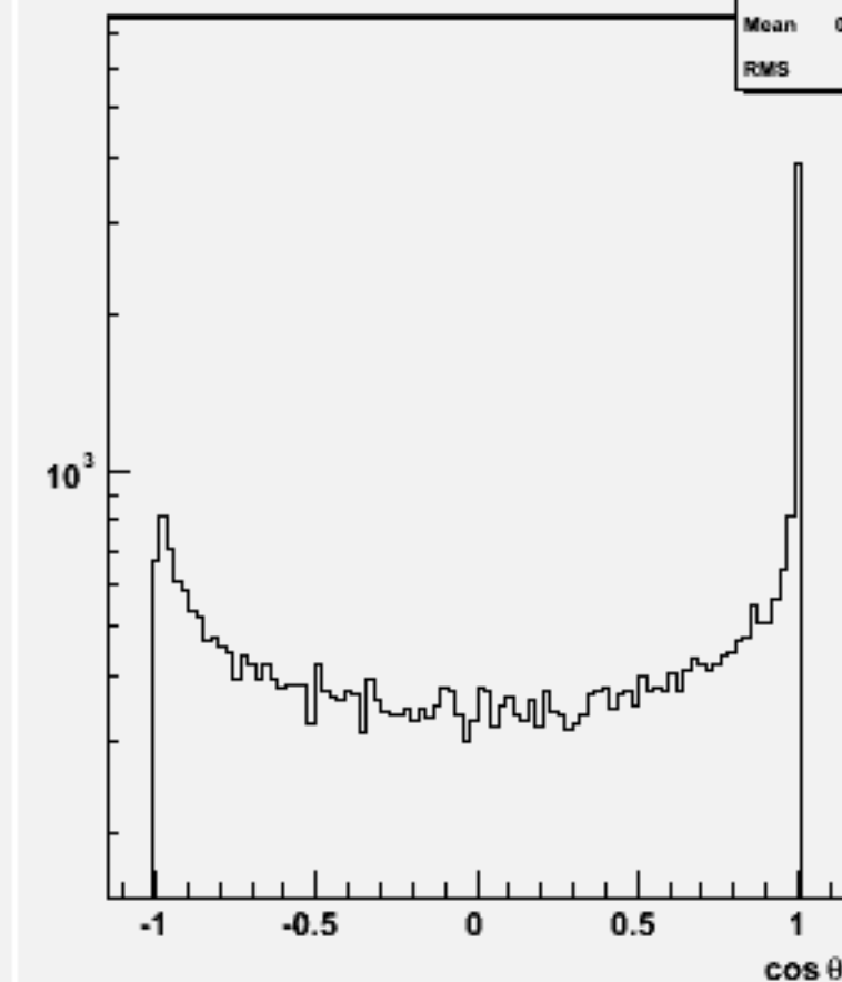
Jet cos \theta (All jets)w100884 e2e2cse3n3_o
