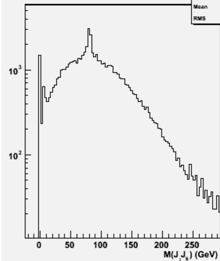
2jets mass(All comb)w100884 e2e2cse3n3_o
