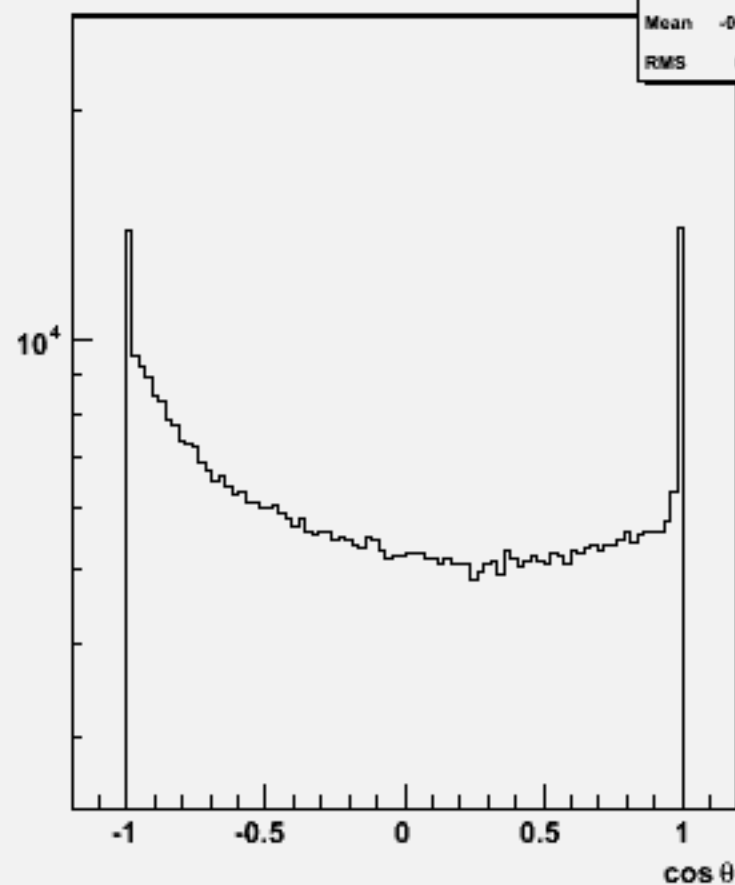
Particle cos \theta : w100884 e2e2cse3n3_o
