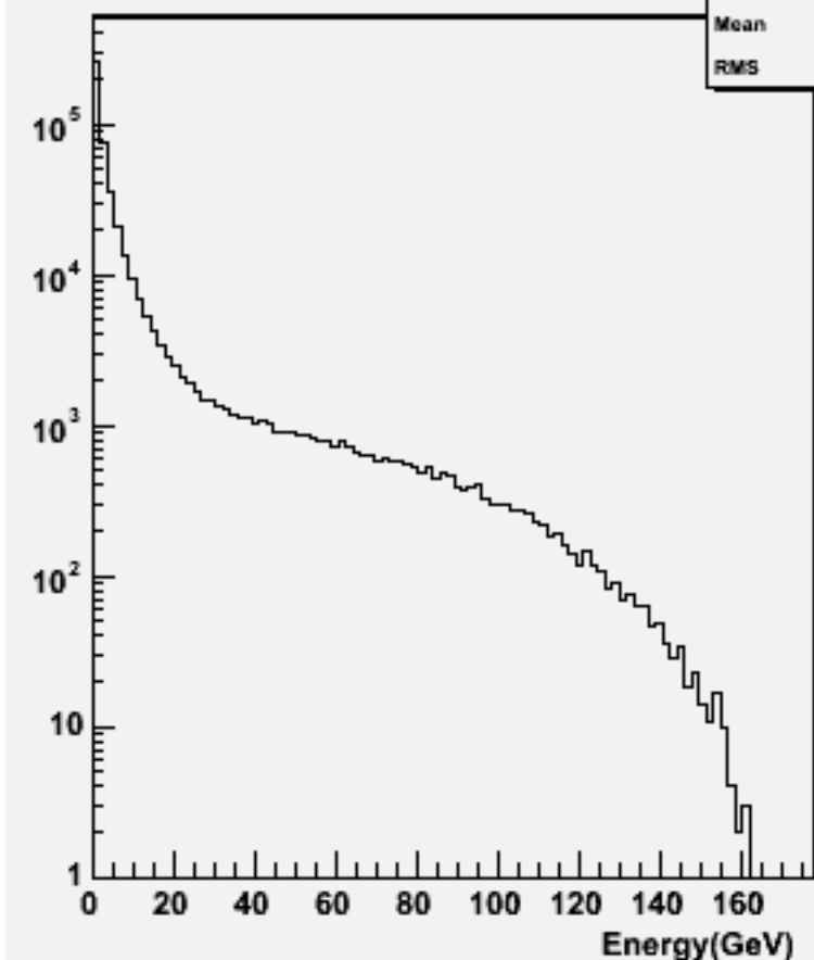
Start point R : w100881 e2e2cse2n2_o
