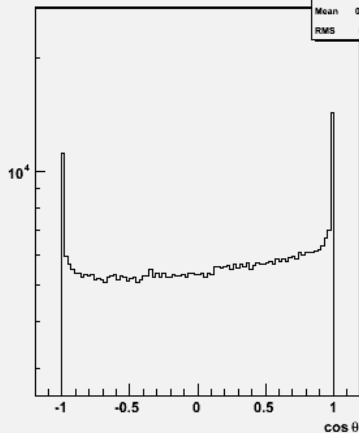
Particle cos \theta : w100881 e2e2cse2n2_o
