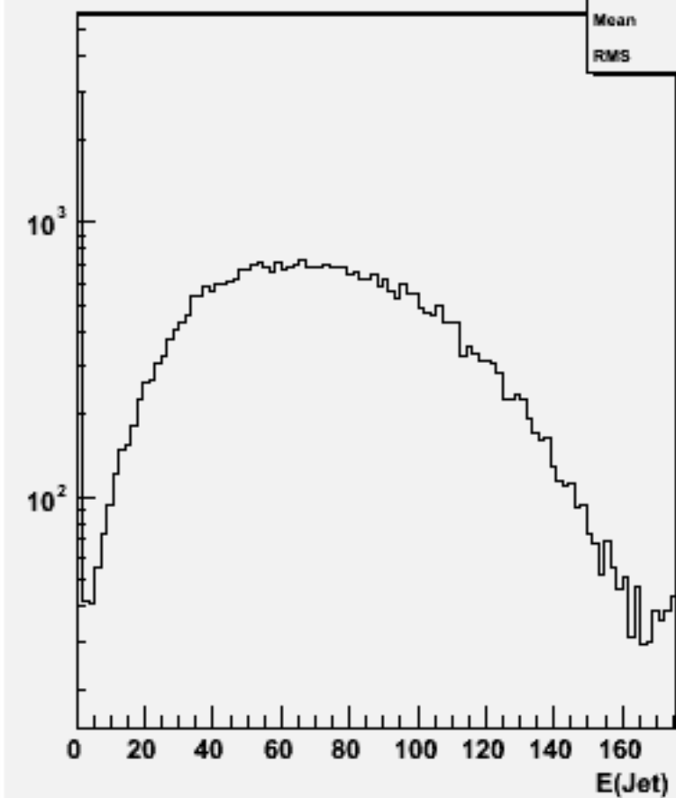
Jet energies(All jets)w100881 e2e2cse2n2_o
