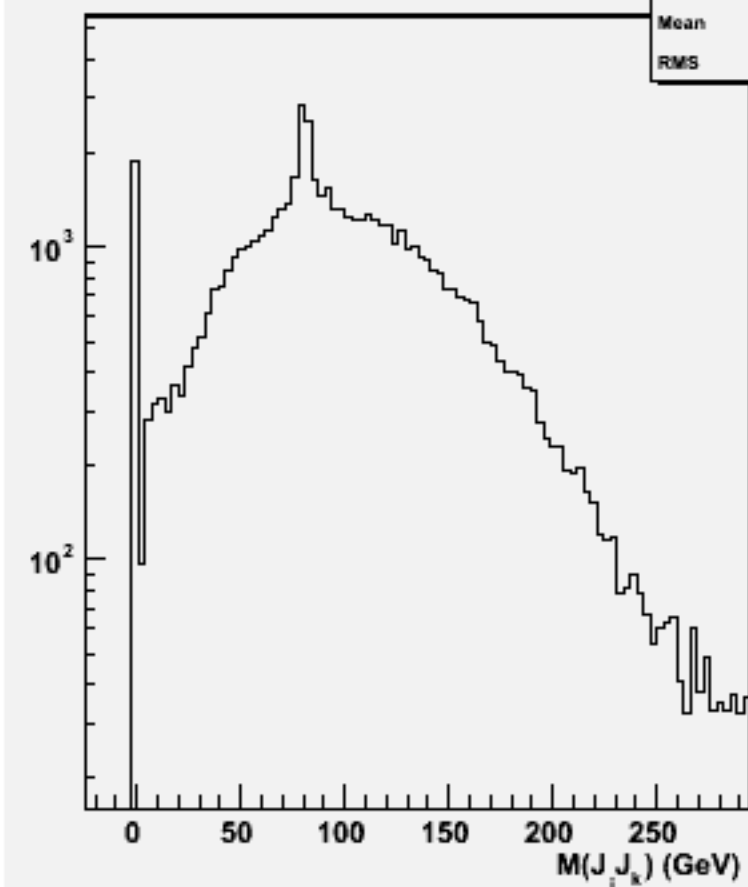
2jets mass(All comb)w100881 e2e2cse2n2_o
