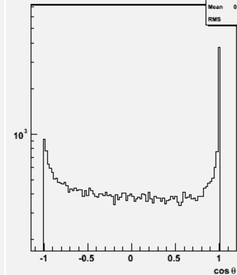
Jet cos \theta (All jets)w100881 e2e2cse2n2_o
