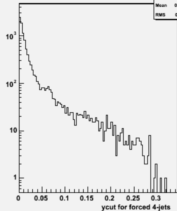
Ycut for 4-jets :w100881 e2e2cse2n2_o
