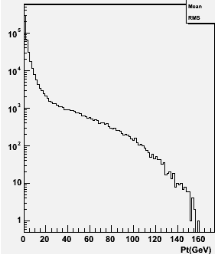
Start point Z : w100881 e2e2cse2n2_o
