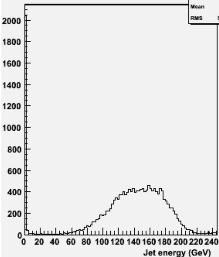
energy for 2-jets :w100880 e2e2cse2n2_o
