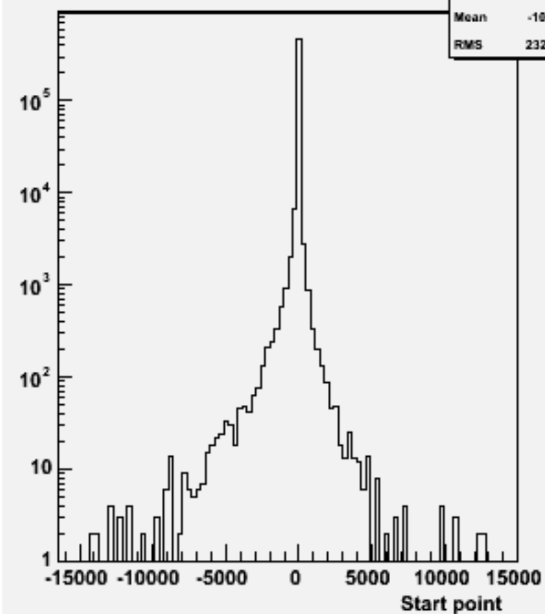
Start point Z : w100880 e2e2cse2n2_o
