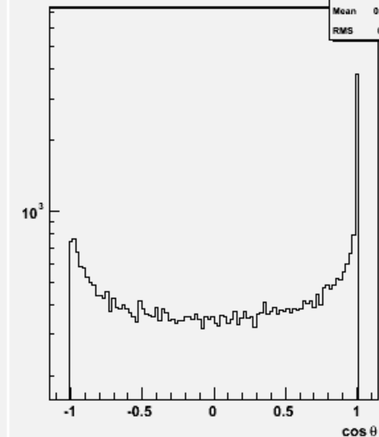
Jet cos \theta (All jets)w100880 e2e2cse2n2_o
