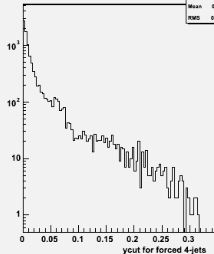
Ycut for 4-jets :w100880 e2e2cse2n2_o
