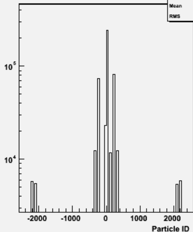
Particle ID : w100880 e2e2cse2n2_o
