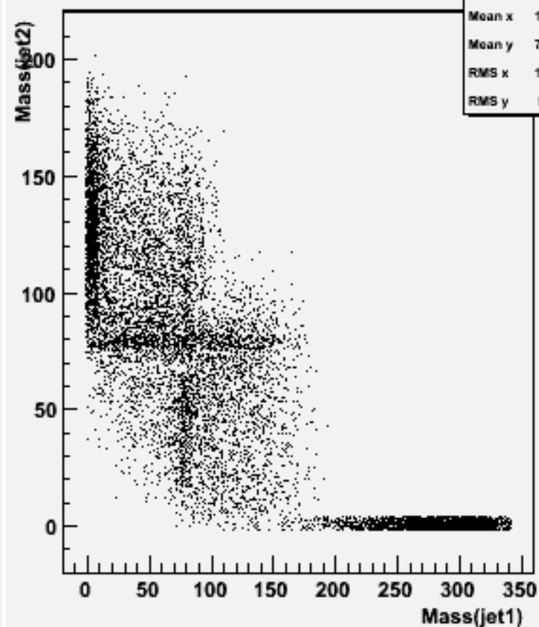
Jet mass for forced 2-jets : w100880 e2e2cse2n2_o
