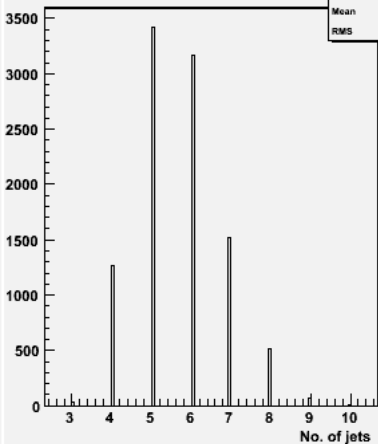
No. jets (ycut=0.001) : w100880 e2e2cse2n2_o
