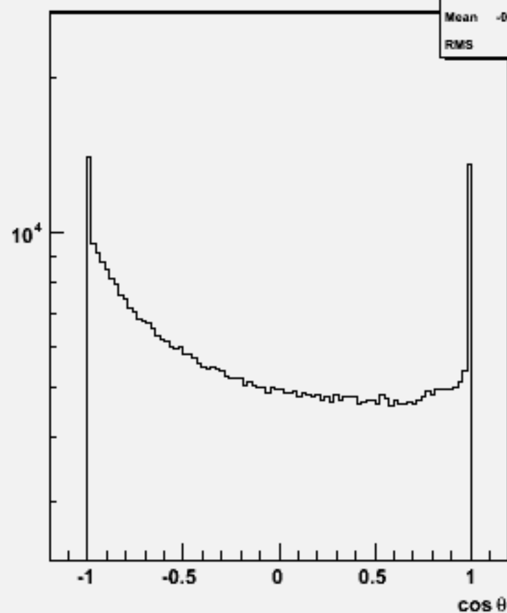
Particle \cos\theta : w100880 e2e2cse2n2_o
