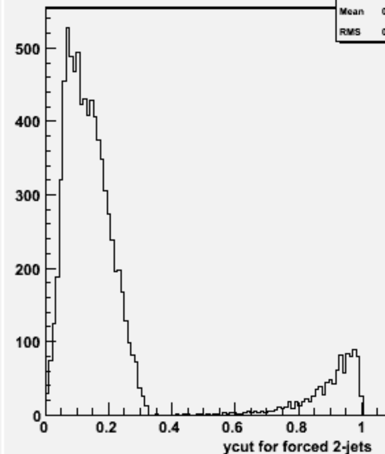
Ycut for 2-jets :w100880 e2e2cse2n2_o
