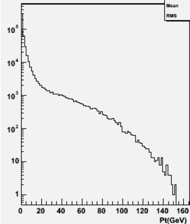
Particle Pt : w100880 e2e2cse2n2_o
