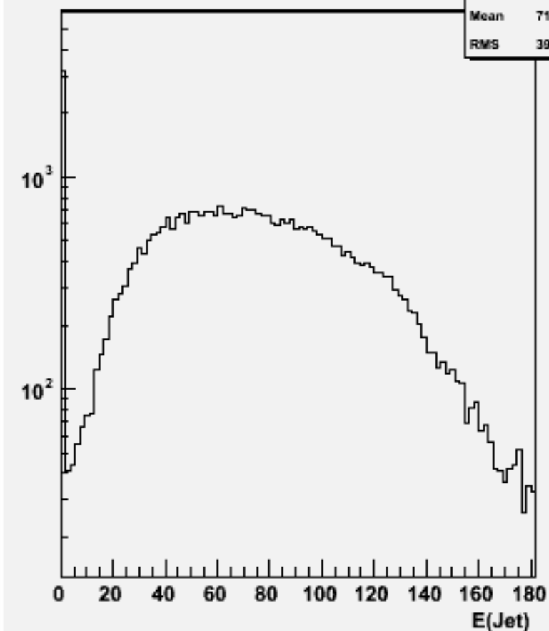
Jet energies(All jets)w100880 e2e2cse2n2_o
