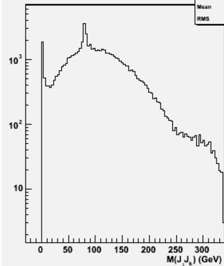
2jets mass(All comb)w100880 e2e2cse2n2_o
