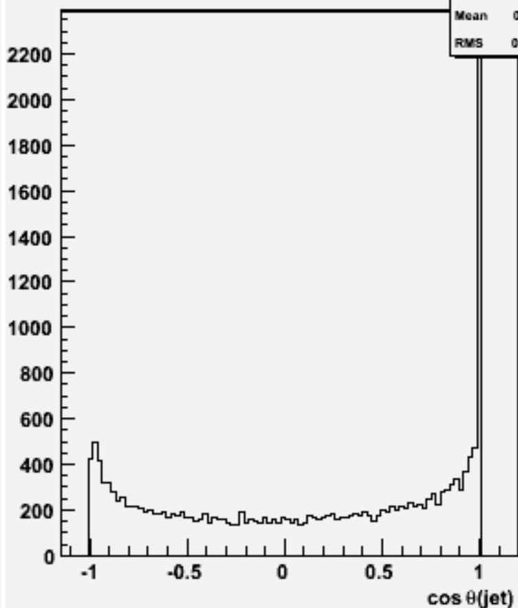
cos \theta for 2-jets :w100880 e2e2cse2n2_o
