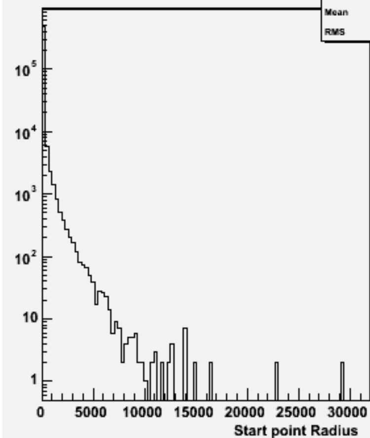
Start point R : w100880 e2e2cse2n2_o
