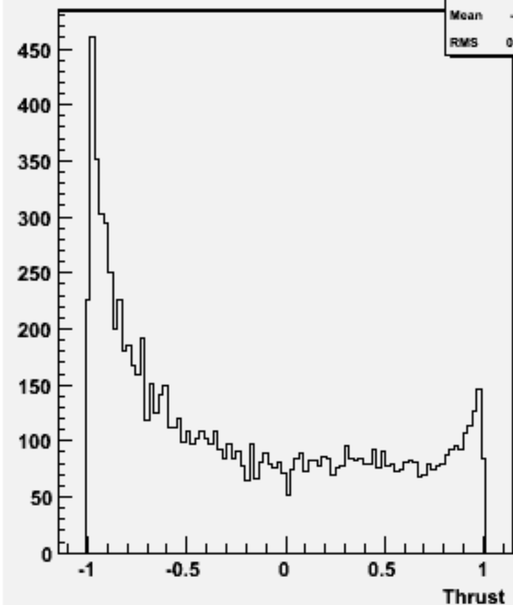
cos \Theta (thrust) w100880 e2e2cse2n2_o
