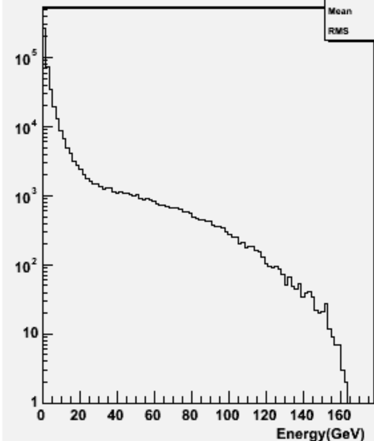
Particle Energy : w100880 e2e2cse2n2_o
