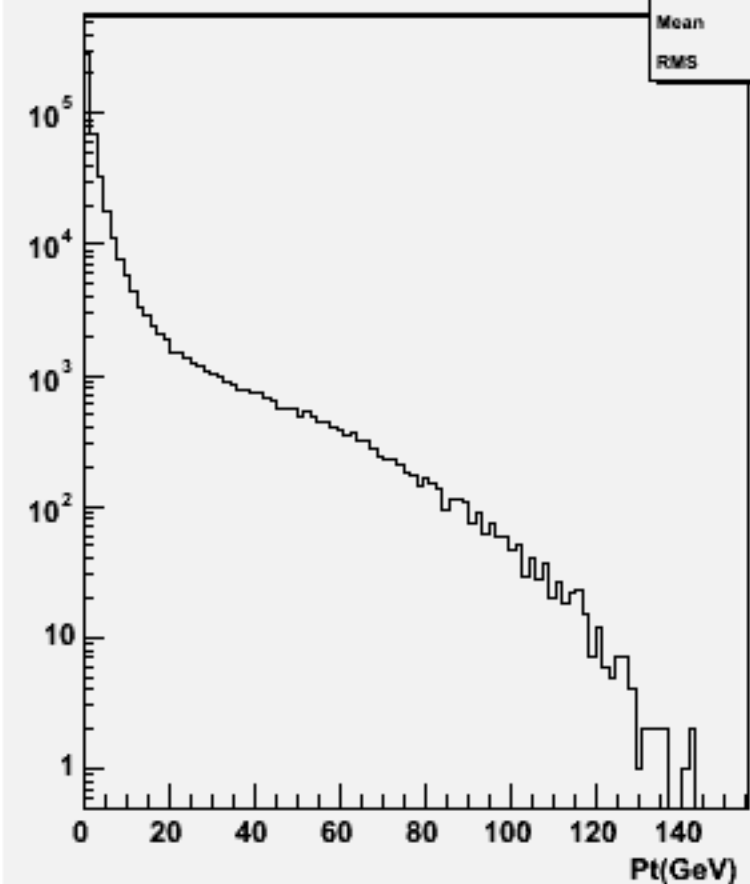
Particle Pt : w100876 e2e2cse1n1_o
