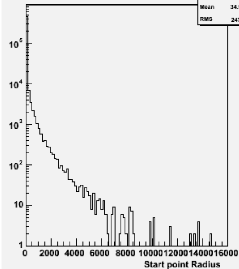
Start point R : w100876 e2e2cse1n1_o
