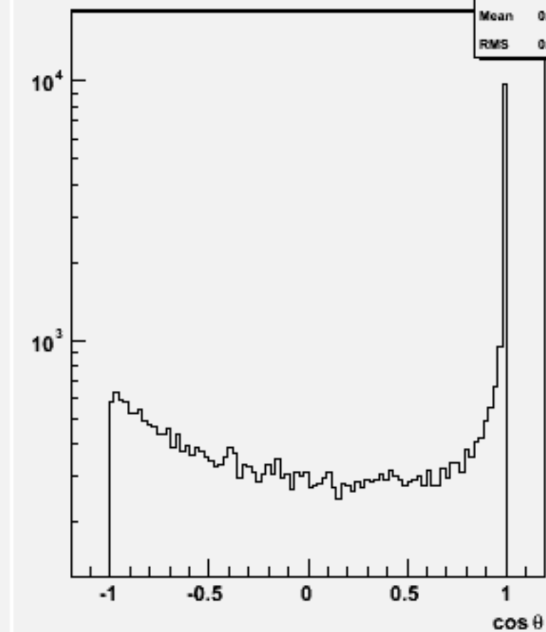
Jet cos \theta (All jets)w100876 e2e2cse1n1_o
