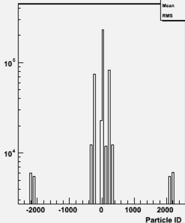
Particle ID : w100876 e2e2cse1n1_o
