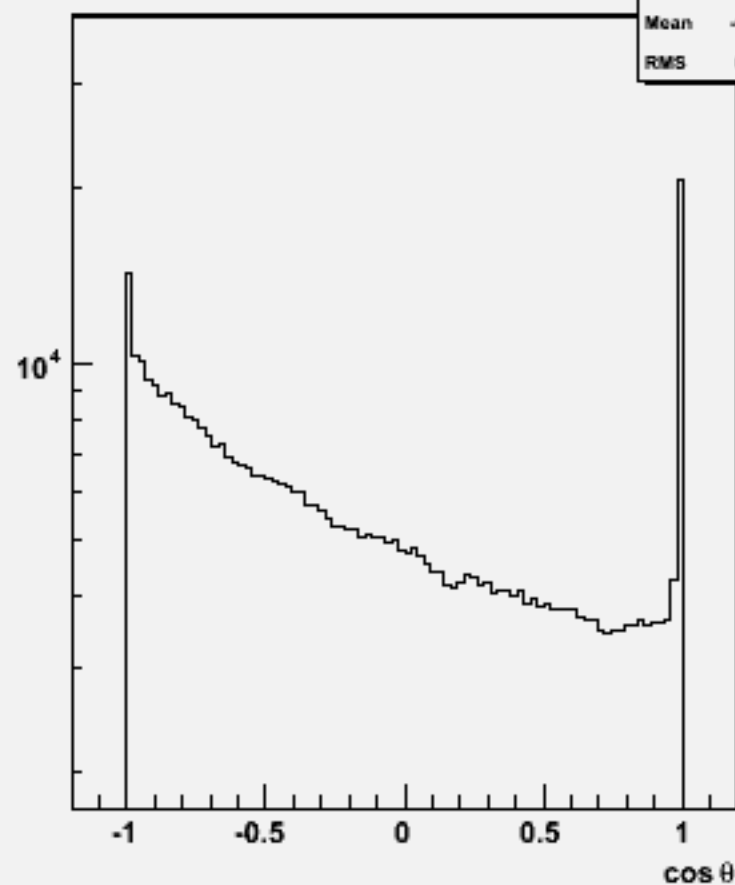
Particle cos \theta : w100876 e2e2cse1n1_o
