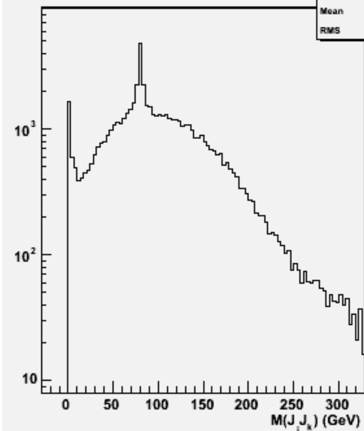
2jets mass(All comb)w100876 e2e2cse1n1_o
