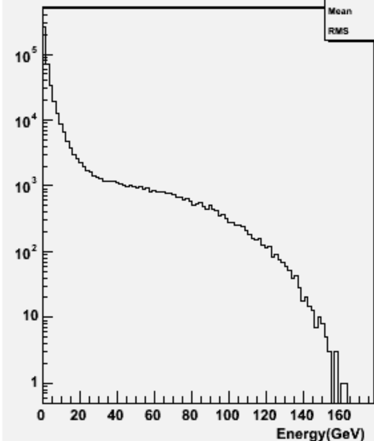
Particle Energy : w100876 e2e2cse1n1_o
