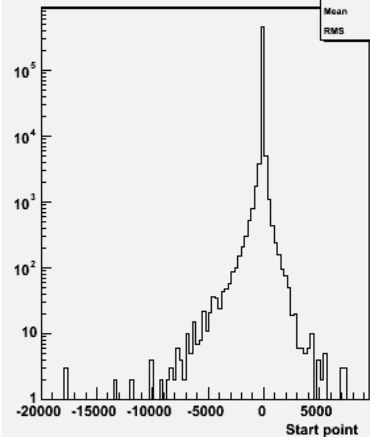
Start point Z : w100876 e2e2cse1n1_o
