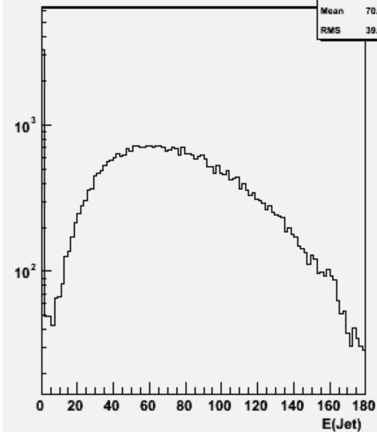
Jet energies(All jets)w100876 e2e2cse1n1_o
