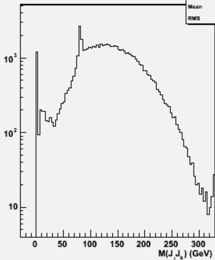
2jets mass(All comb)w100873 e2e2udsc_o
