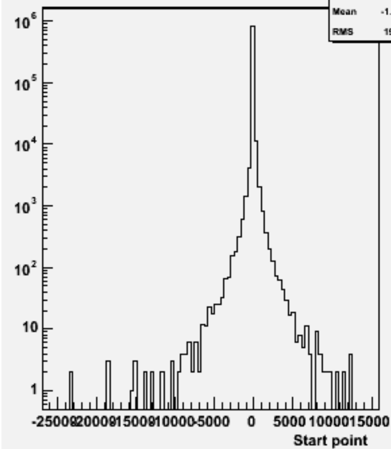
Start point Z : w100873 e2e2udsc_o
