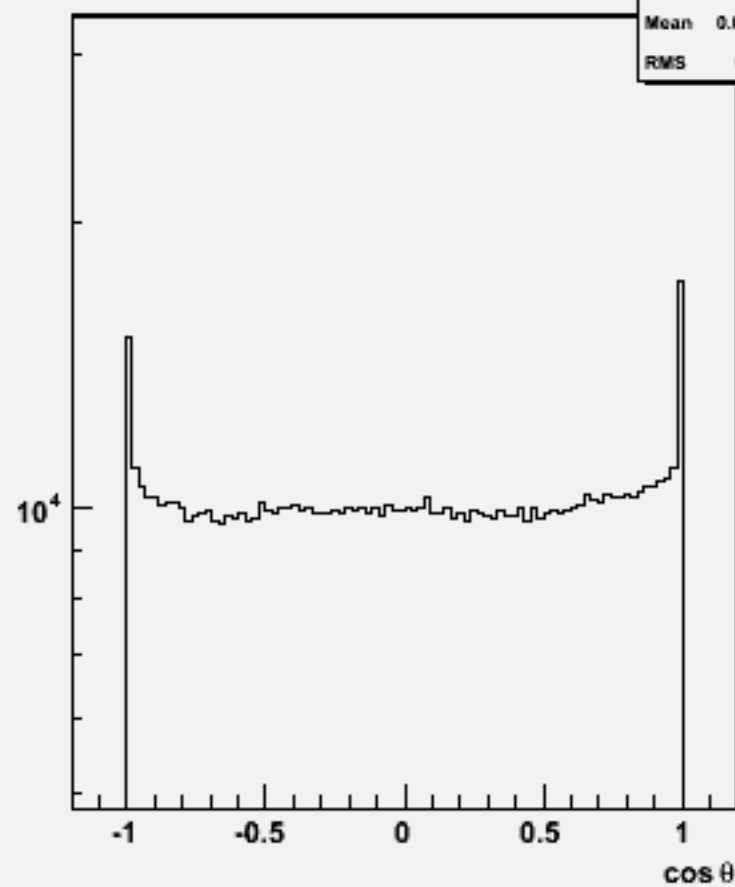
Particle cos \theta : w100873 e2e2udsc_o
