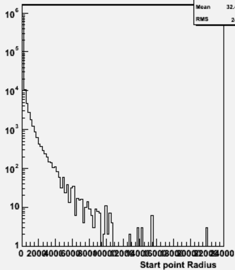
Start point R : w100873 e2e2udsc_o
