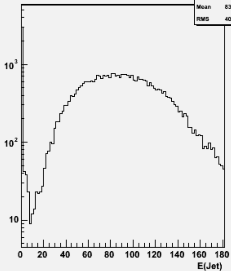
Jet energies(All jets)w100873 e2e2udsc_o
