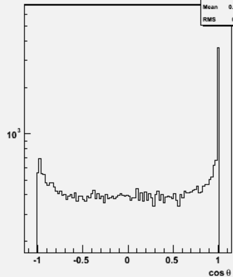
Jet cosθ (All jets)w100873 e2e2udsc_o
