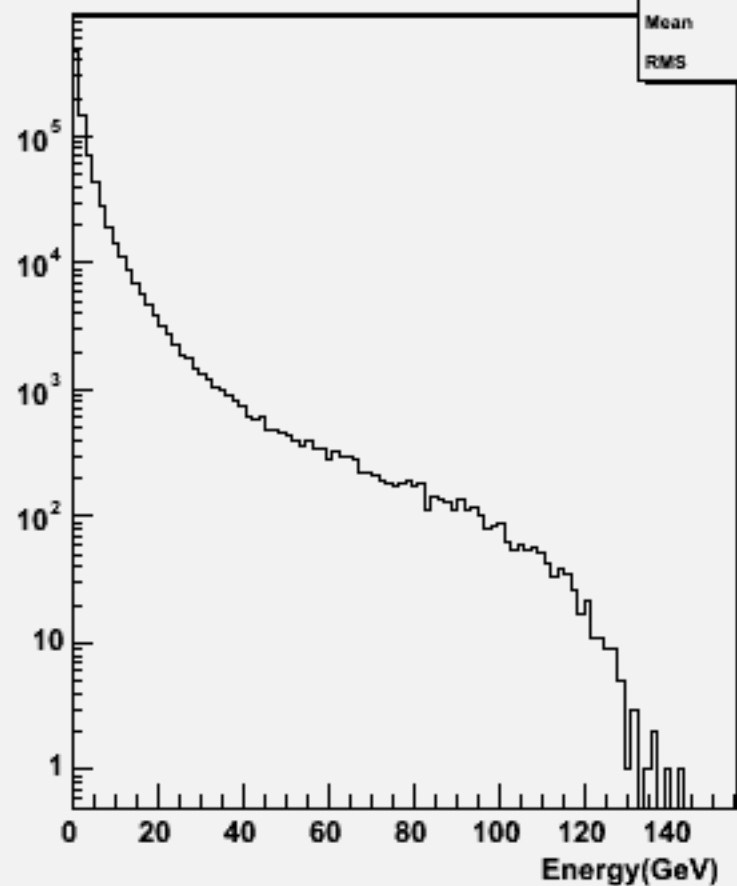
Particle Energy : w100873 e2e2udsc_o
