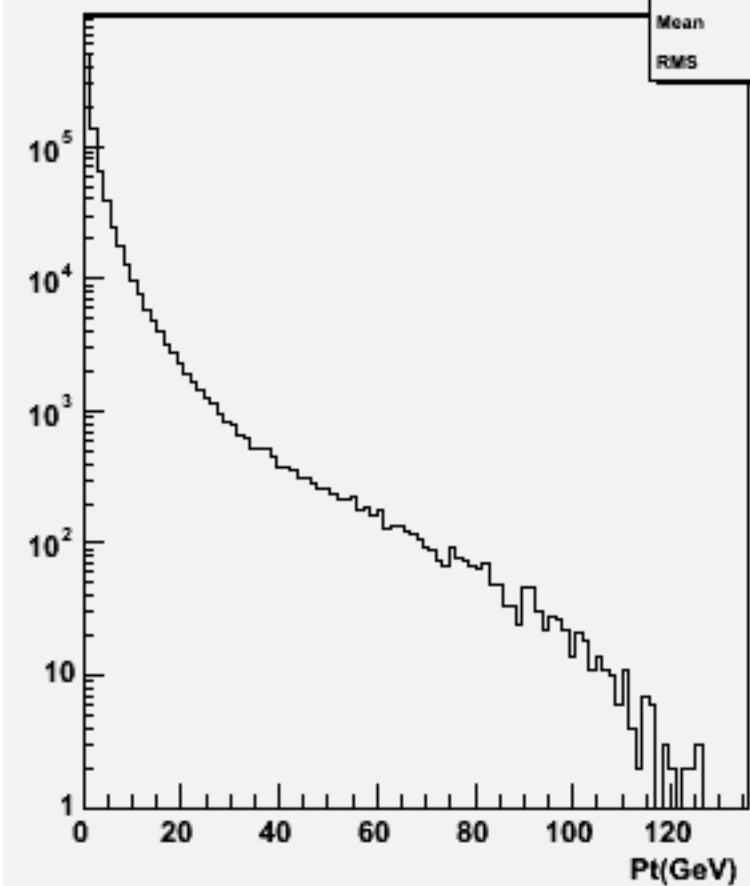
Particle Pt : w100873 e2e2udsc_o
