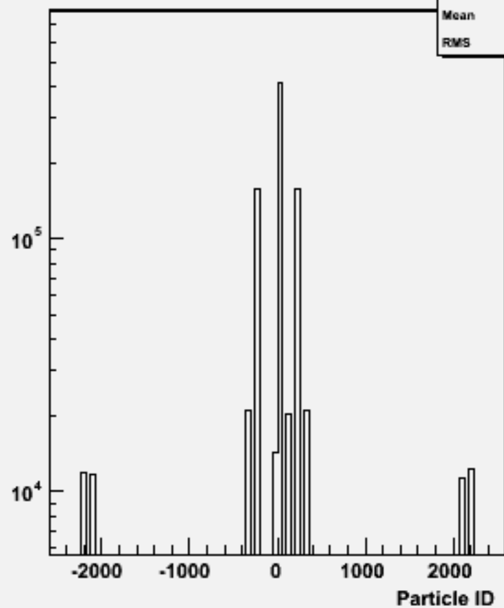
Particle ID : w100873 e2e2udsc_o
