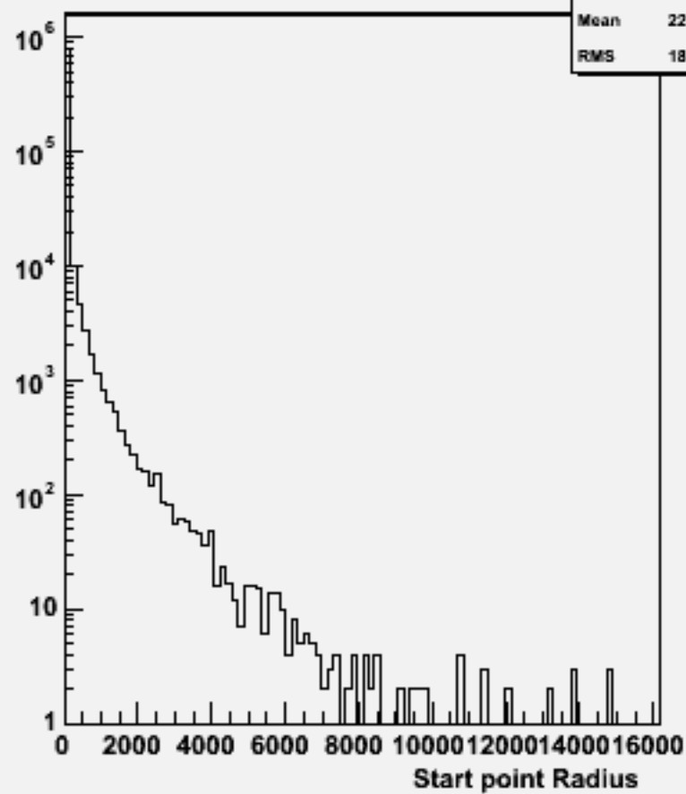
Start point R : w100869 e2e2uddu_o
