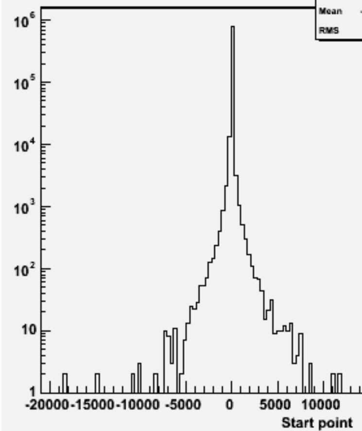
Start point Z : w100869 e2e2uddu_o
