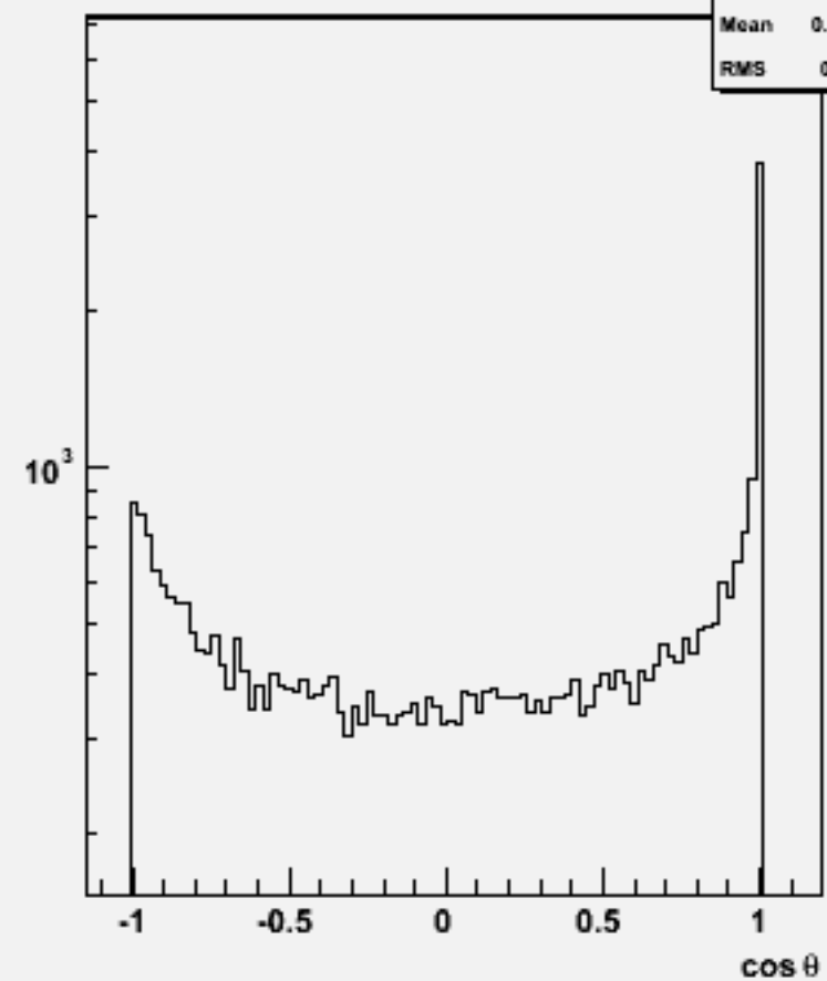
Jet cosθ (All jets)w100869 e2e2uddu_o
