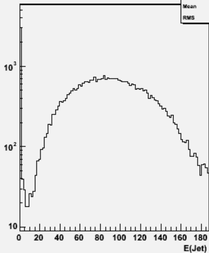
Jet energies(All jets)w100869 e2e2uddu_o
