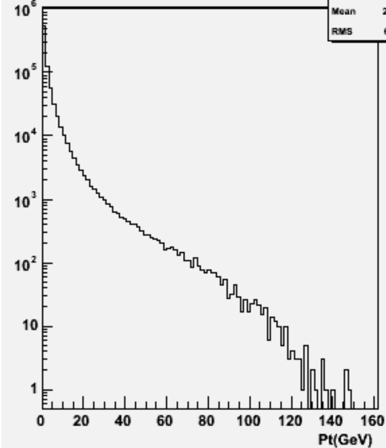
Particle Pt : w100869 e2e2uddu_o
