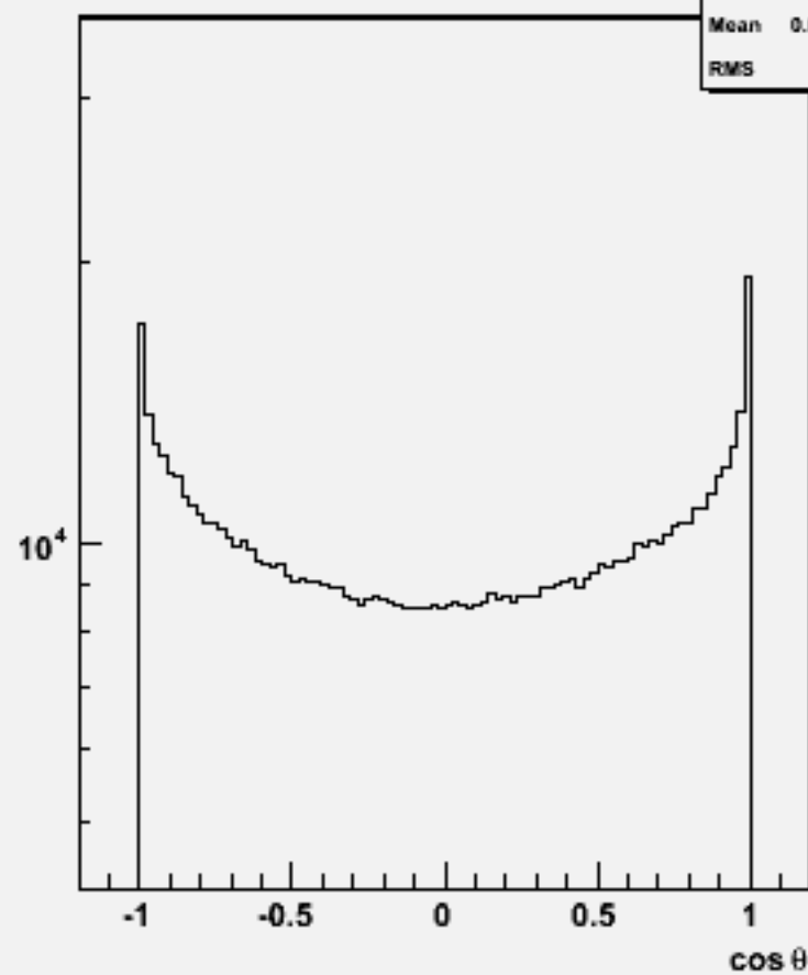
Particle cos \theta : w100869 e2e2uddu_o
