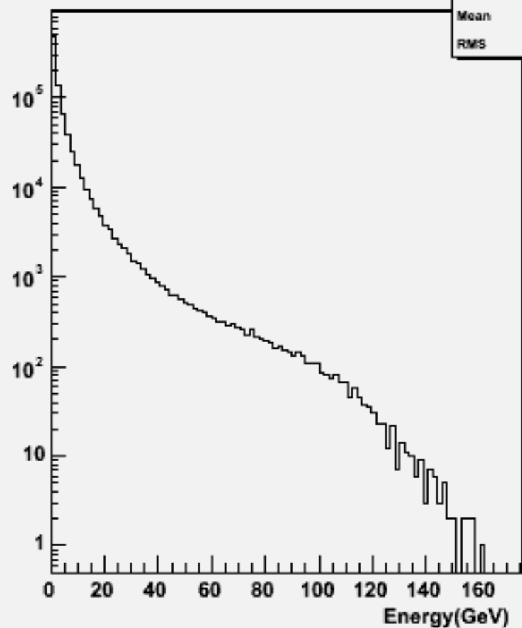
Particle Energy : w100869 e2e2uddu_o
