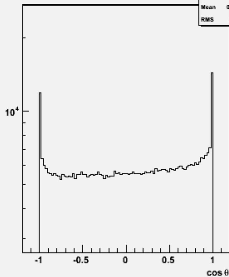
Particle cosθ : w100865 e2e2ude3n3_o
