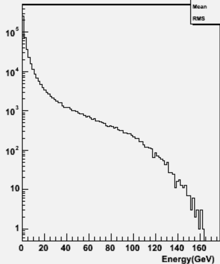
Start point R : w100865 e2e2ude3n3_o
