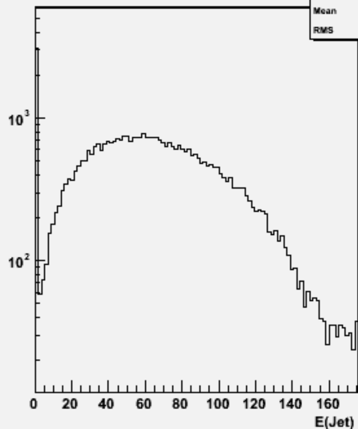
Jet energies(All jets)w100865 e2e2ude3n3_o
