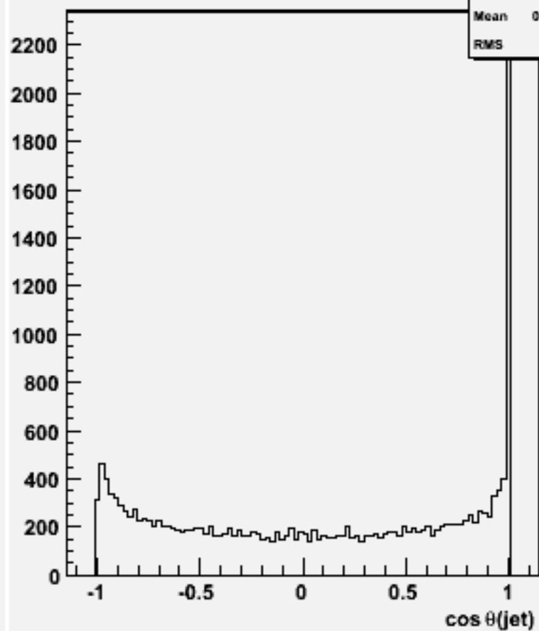
cos \theta for 2-jets :w100865 e2e2ude3n3_o
