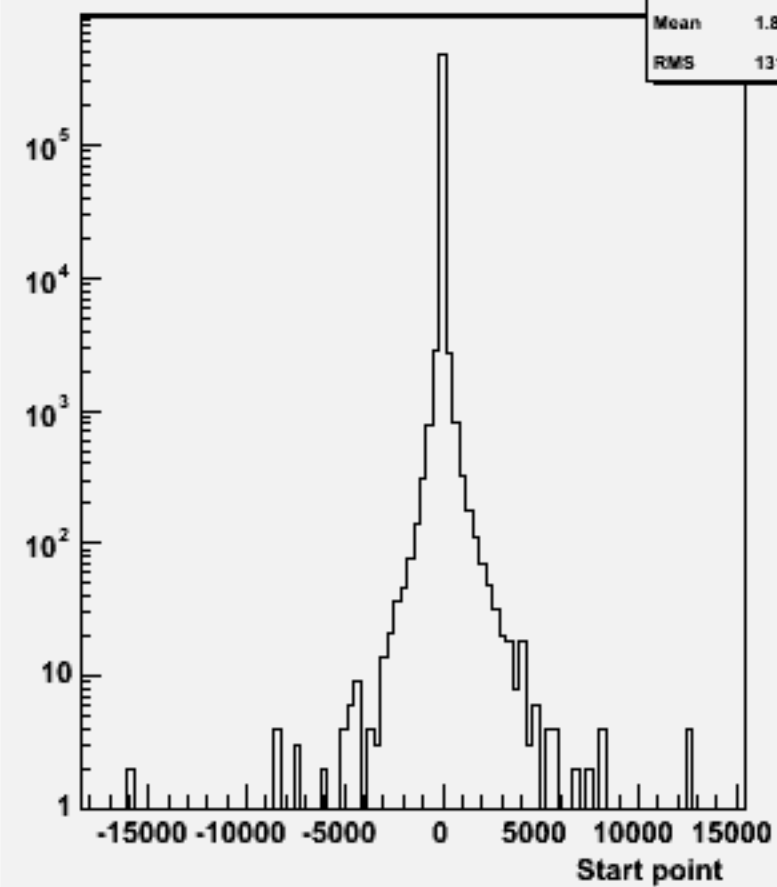
Start point Z : w100865 e2e2ude3n3_o
