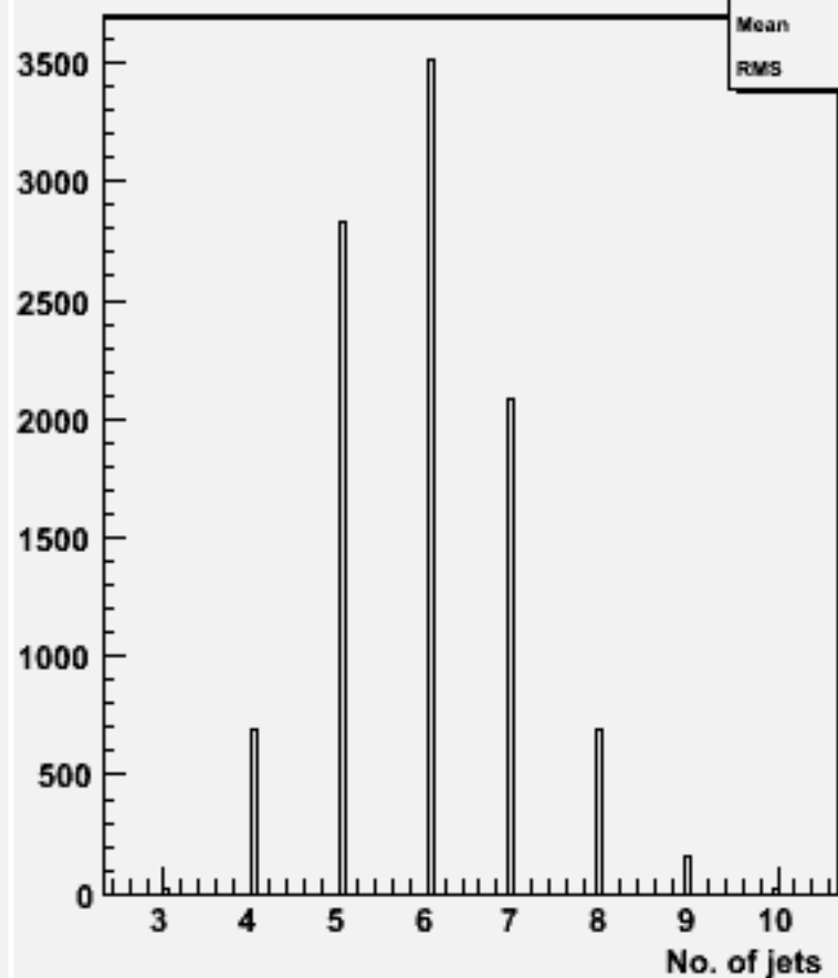
No. jets (ycut=0.001) : w100865 e2e2ude3n3_o
