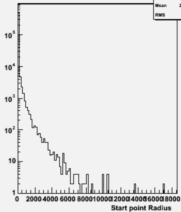
Start point R : w100865 e2e2ude3n3_o
