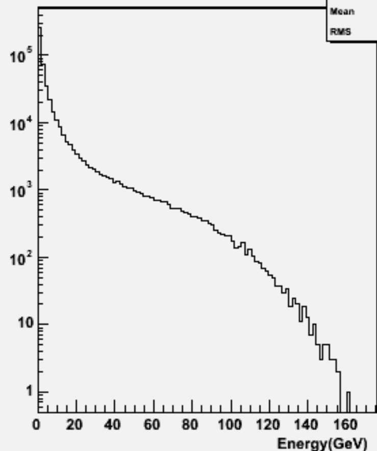
Start point R : w100864 e2e2ude3n3_o
