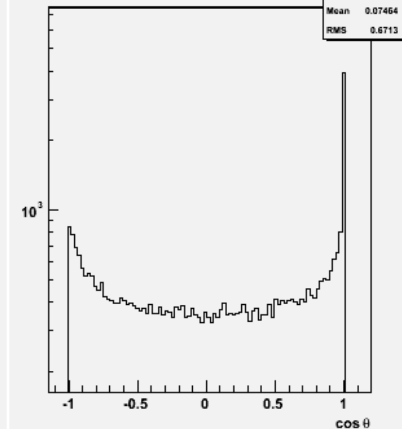
Jet cos \theta (All jets)w100864 e2e2ude3n3_o
