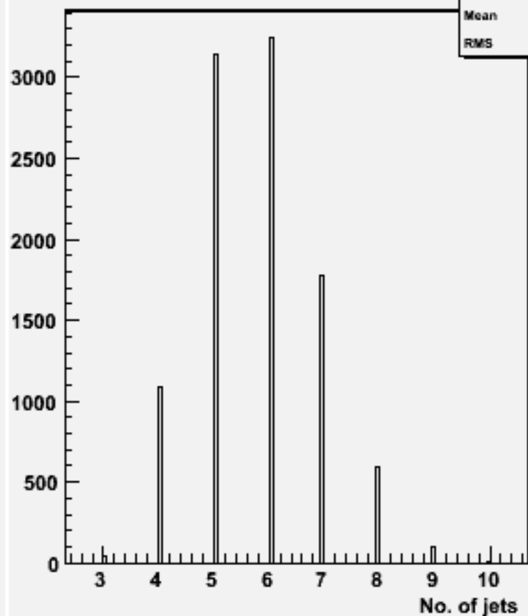
No. jets (ycut=0.001) : w100864 e2e2ude3n3_o
