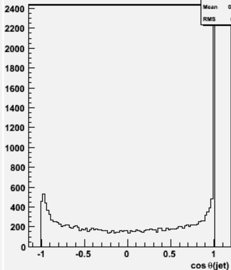
cos \theta for 2-jets :w100864 e2e2ude3n3_o
