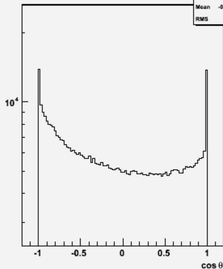
Particle \cos\theta : w100864 e2e2ude3n3_o
