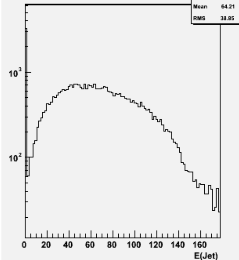
Jet energies(All jets)w100864 e2e2ude3n3_o
