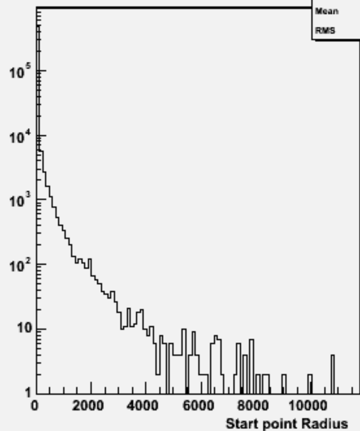
Start point R : w100864 e2e2ude3n3_o
