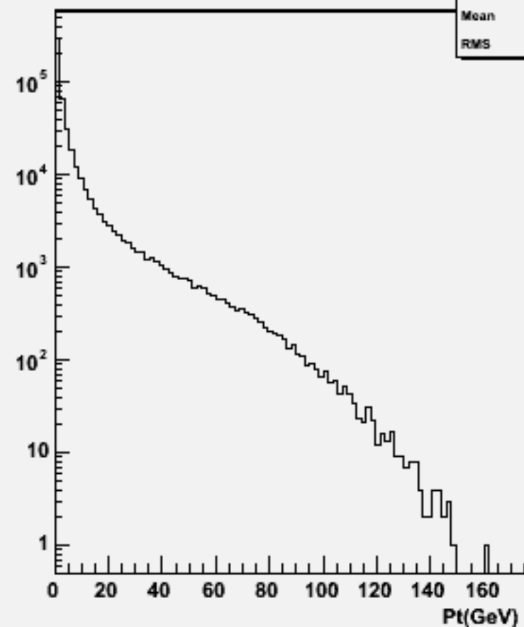
Start point Z : w100864 e2e2ude3n3_o
