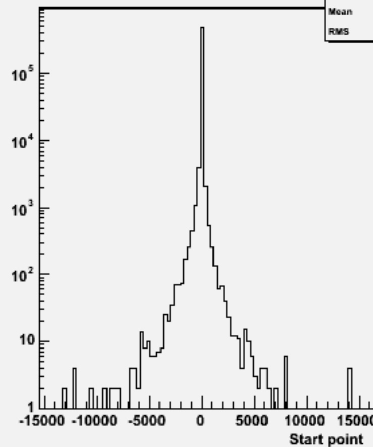
Start point Z : w100864 e2e2ude3n3_o
