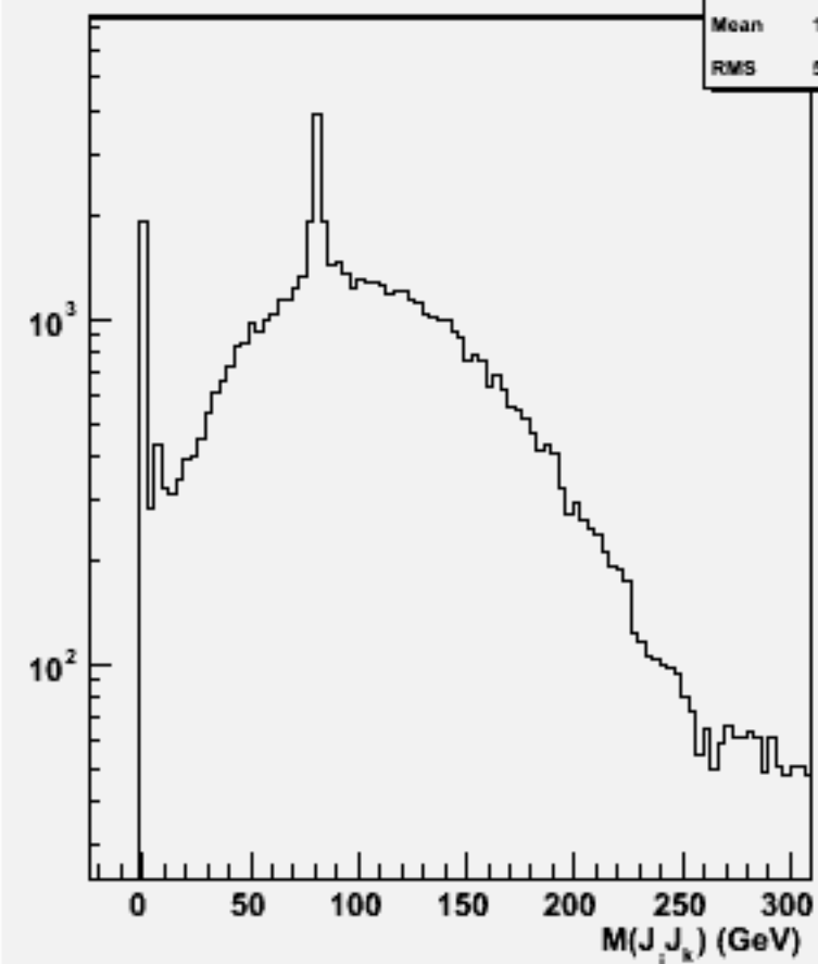
2jets mass(All comb)w100860 e2e2ude2n2_o
