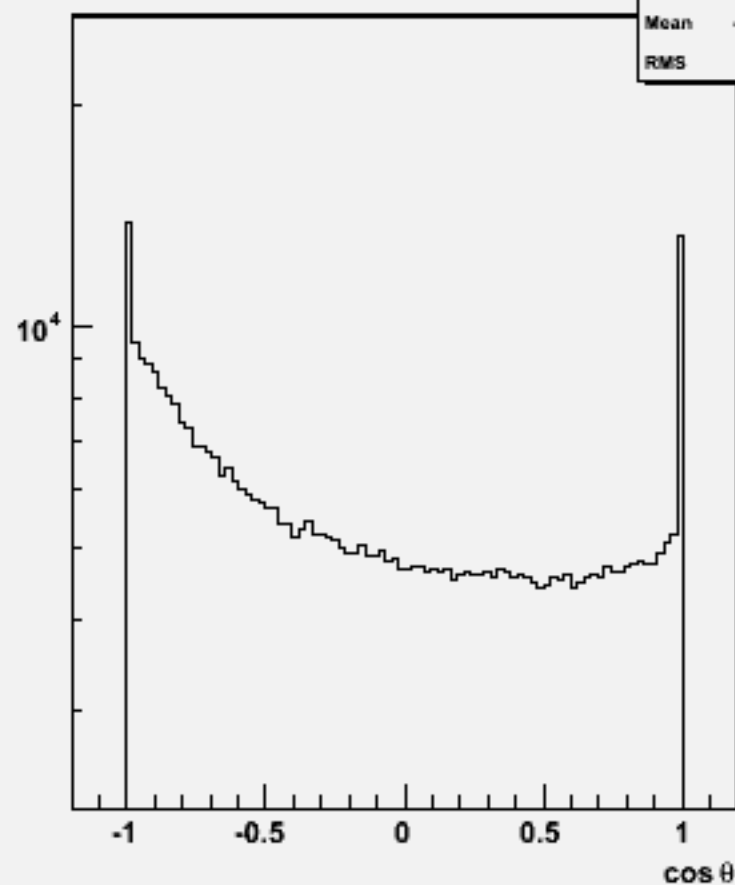
Particle cos \theta : w100860 e2e2ude2n2_o
