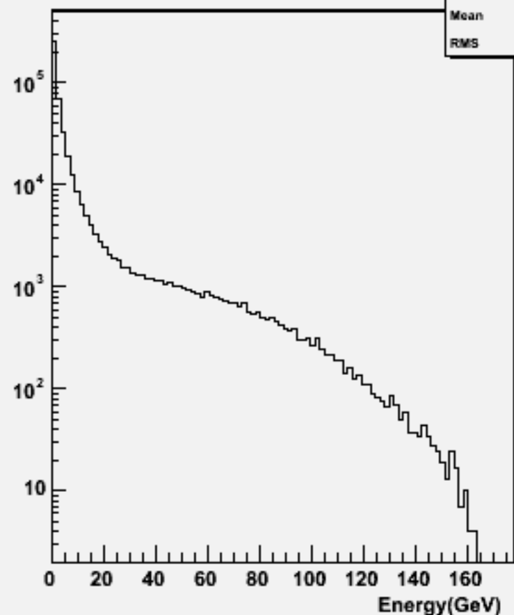
Particle Energy : w100860 e2e2ude2n2_o
