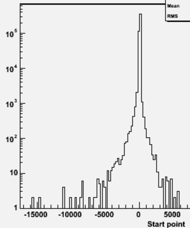
Start point Z : w100860 e2e2ude2n2_o
