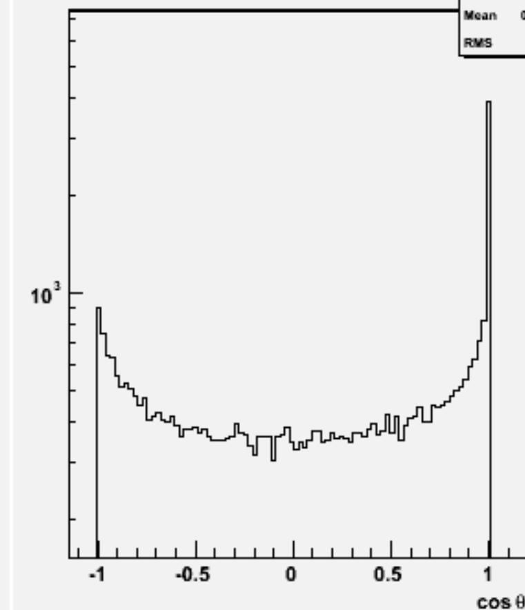
Jet cos \theta (All jets)w100860 e2e2ude2n2_o
