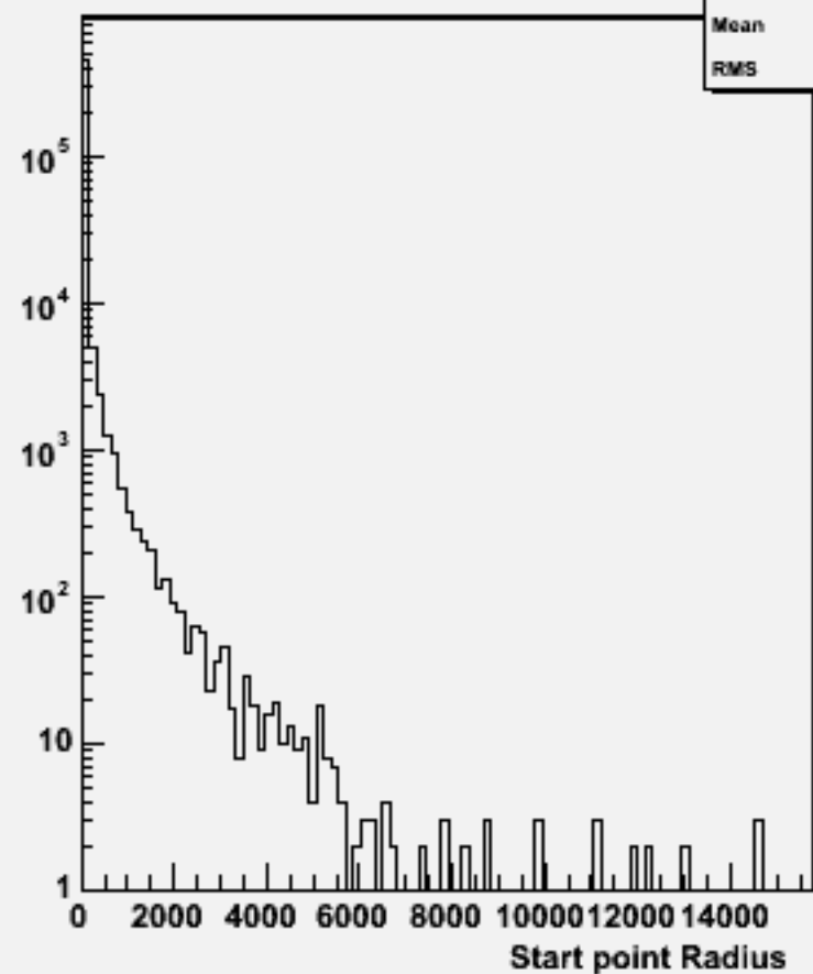
Start point R : w100860 e2e2ude2n2_o
