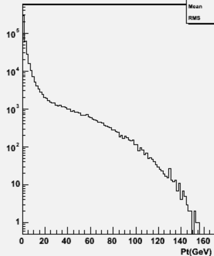
Particle Pt : w100860 e2e2ude2n2_o
