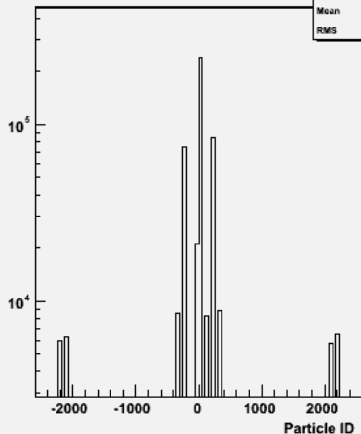
Particle ID : w100860 e2e2ude2n2_o
