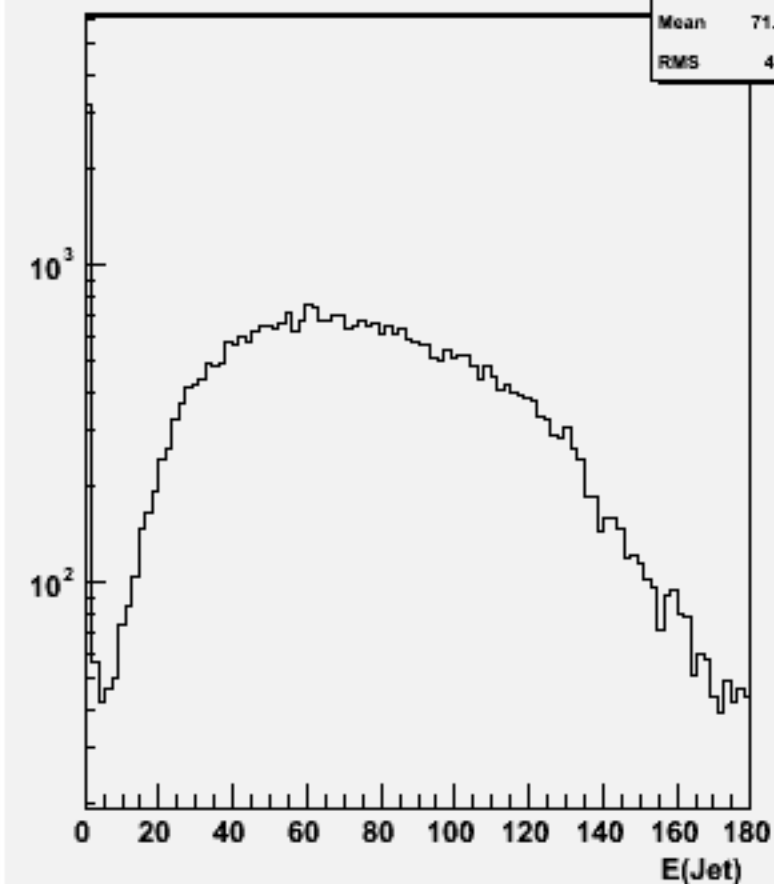
Jet energies(All jets)w100860 e2e2ude2n2_o
