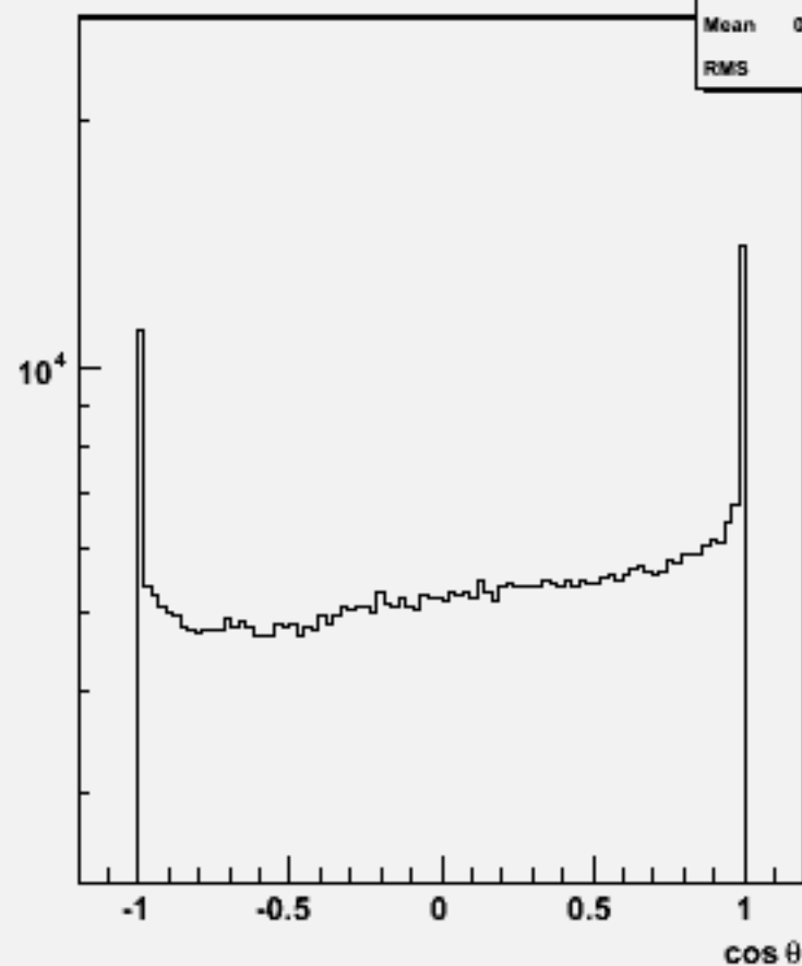
Particle cosθ : w100857 e2e2ude1n1_o
