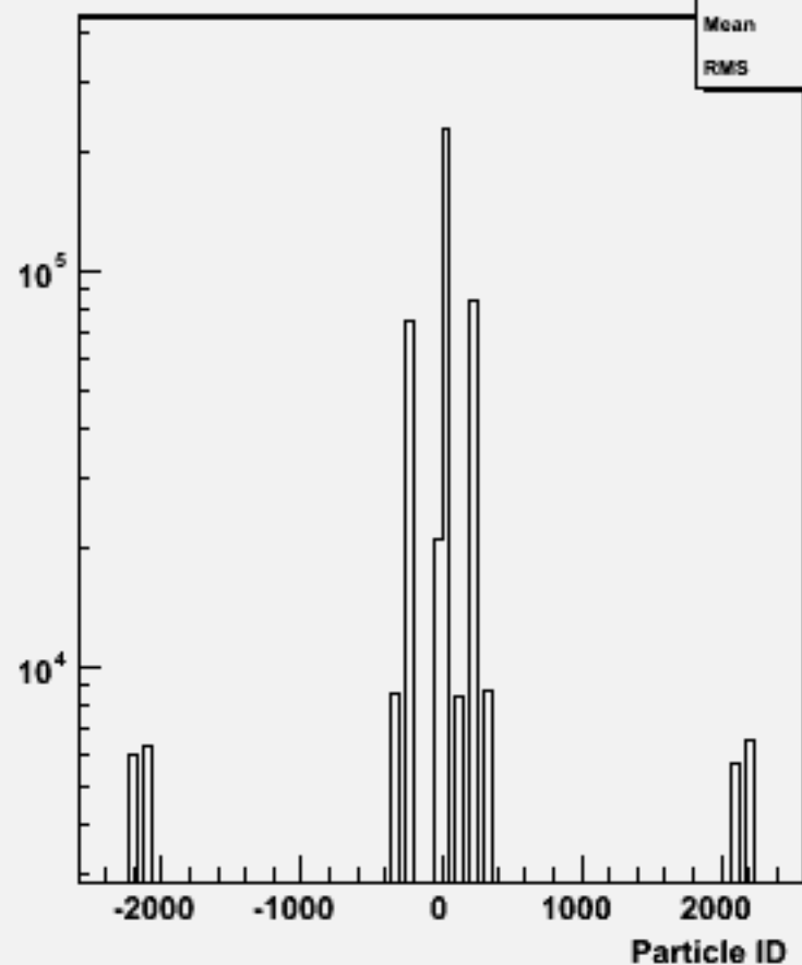
Particle ID : w100857 e2e2ude1n1_o
