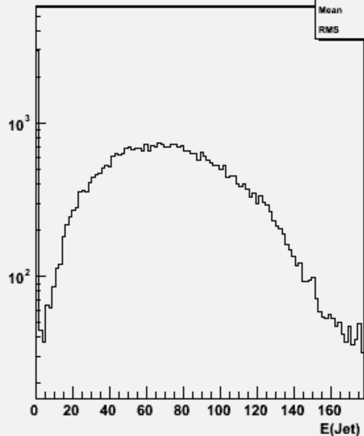
Jet energies(All jets)w100857 e2e2ude1n1_o
