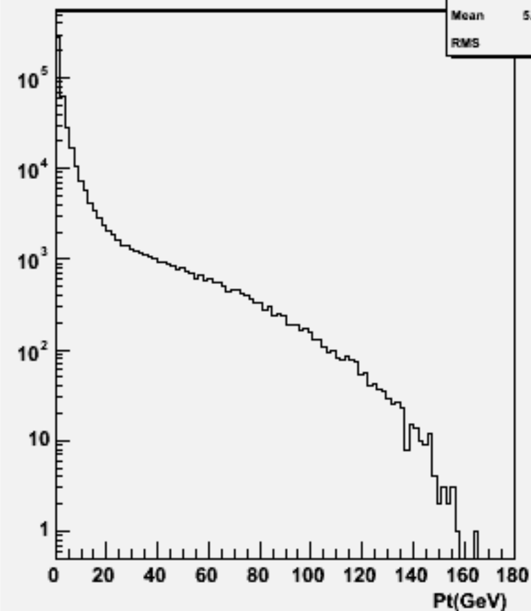
Particle Pt : w100857 e2e2ude1n1_o
