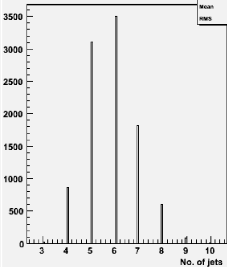
No. jets (ycut=0.001) : w100857 e2e2ude1n1_o
