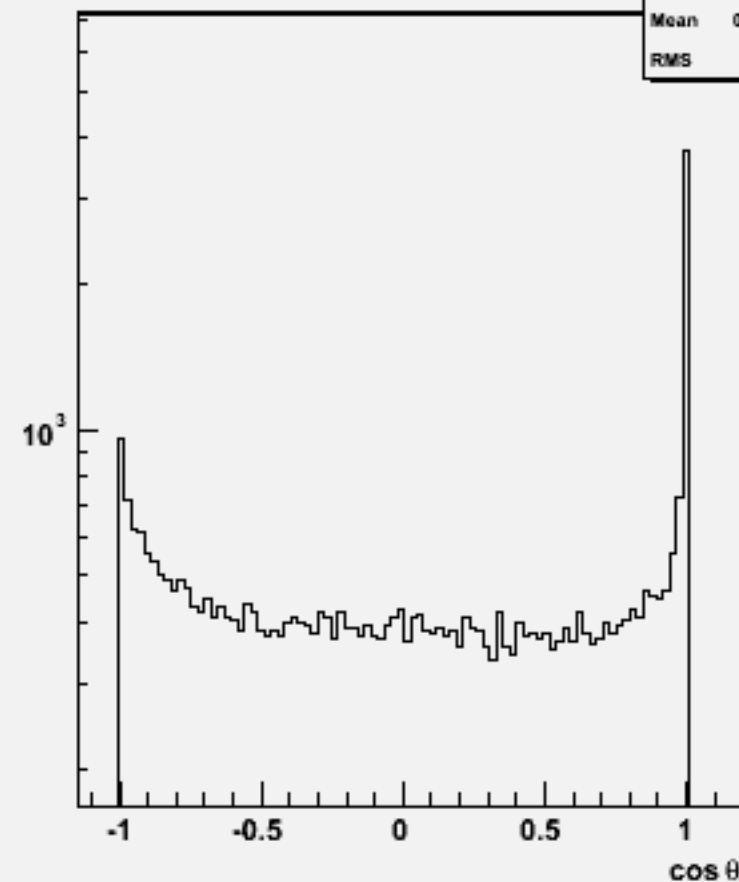
Jet cos \theta (All jets)w100857 e2e2ude1n1_o
