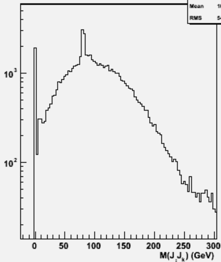
2jets mass(All comb)w100857 e2e2ude1n1_o
