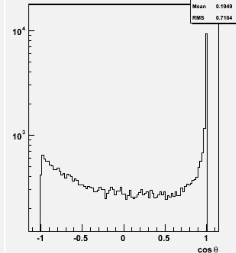
Jet cos \theta (All jets)w100856 e2e2ude1n1_o
