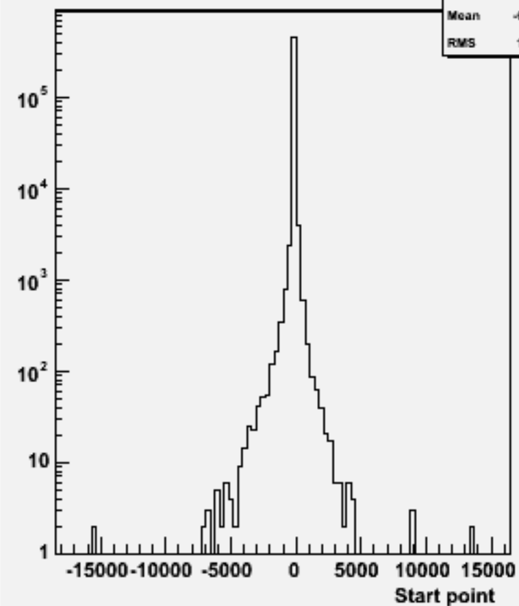
Start point Z : w100856 e2e2ude1n1_o
