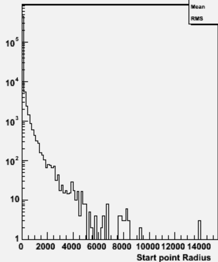
Start point R : w100856 e2e2ude1n1_o
