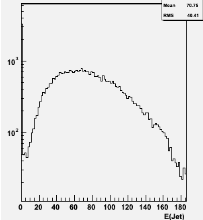
Jet energies(All jets)w100856 e2e2ude1n1_o
