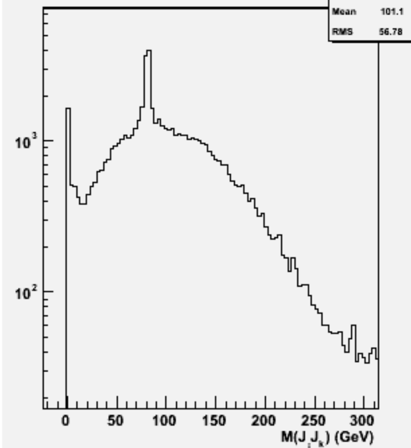
2jets mass(All comb)w100856 e2e2ude1n1_o
