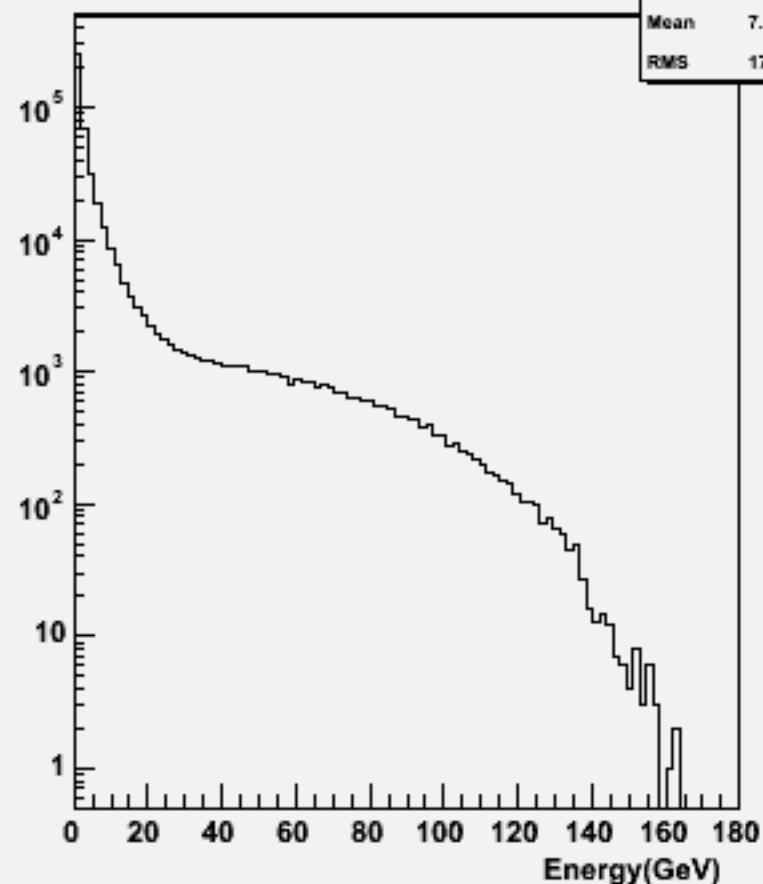
Start point R : w100856 e2e2ude1n1_o
