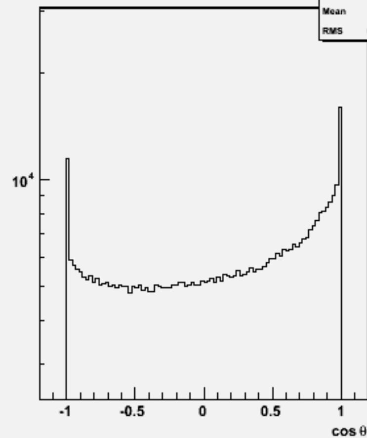
Particle cos \theta : w100848 e2e2n3e3du_o
