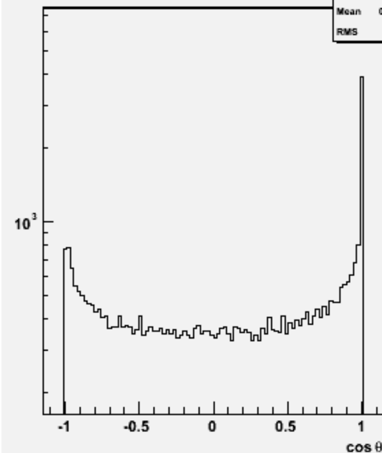
Jet cos \theta (All jets)w100848 e2e2n3e3du_o
