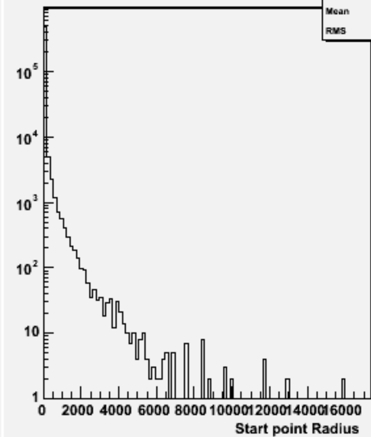
Start point R : w100848 e2e2n3e3du_o
