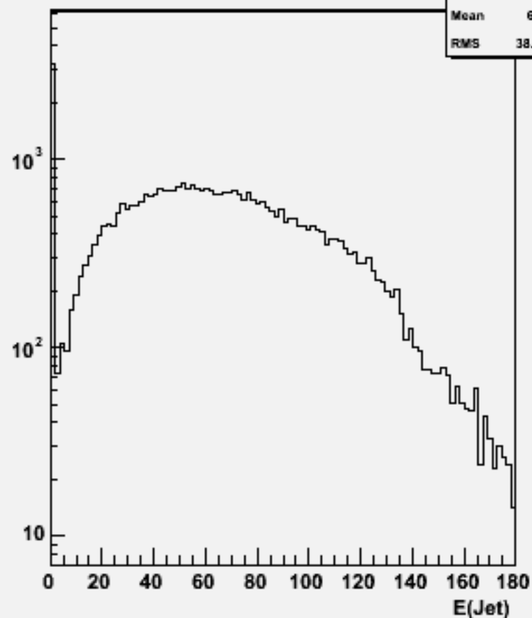
Jet energies(All jets)w100848 e2e2n3e3du_o
