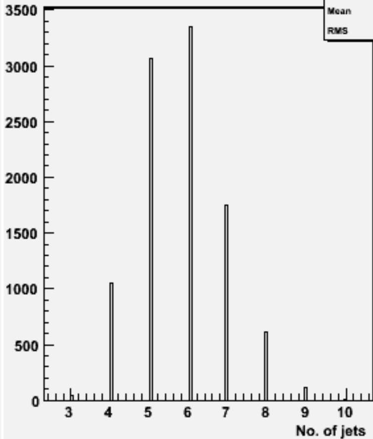
No. jets (ycut=0.001) : w100848 e2e2n3e3du_o
