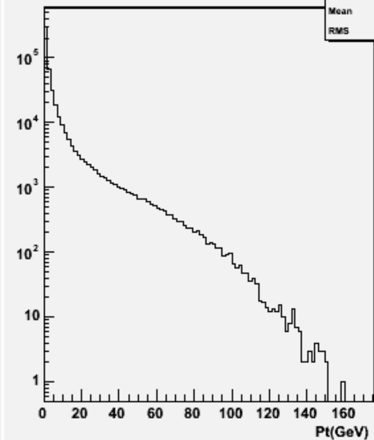
Start point Z : w100848 e2e2n3e3du_o
