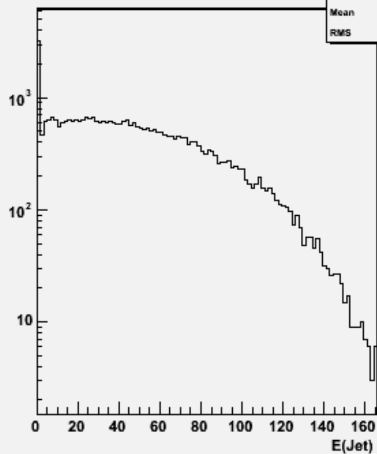
Jet energies(All jets)w100841 e2e2n3e3e2n2_o
