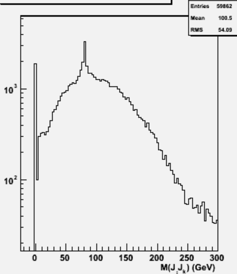
2jets mass(All comb)w100833 e2e2n2e2sc_o
