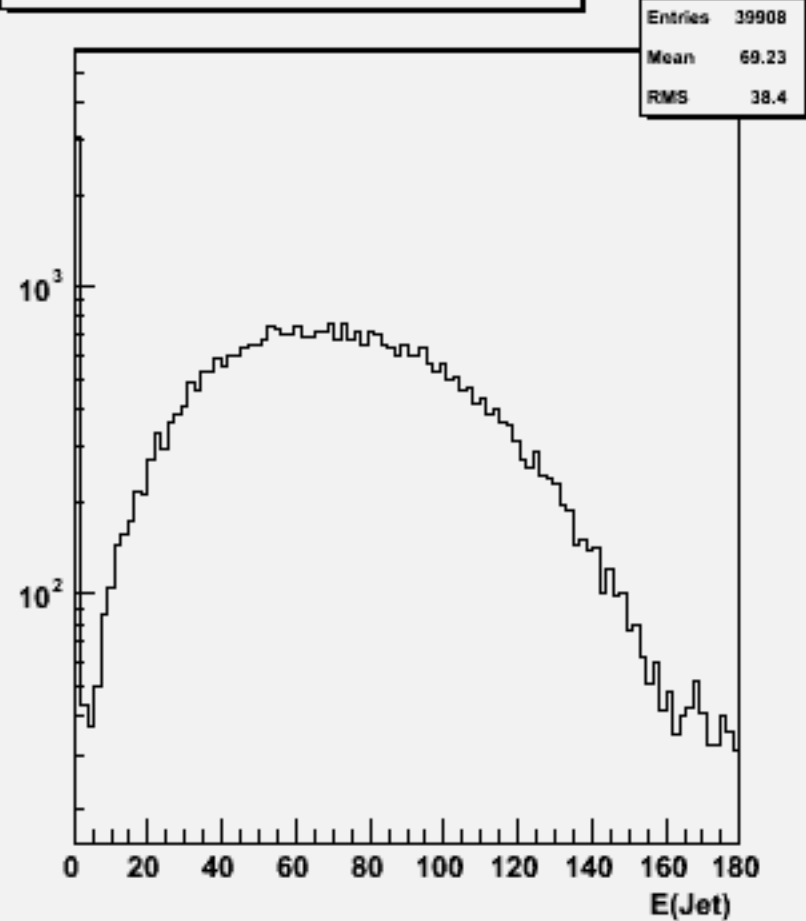
Jet energies(All jets)w100833 e2e2n2e2sc_o
