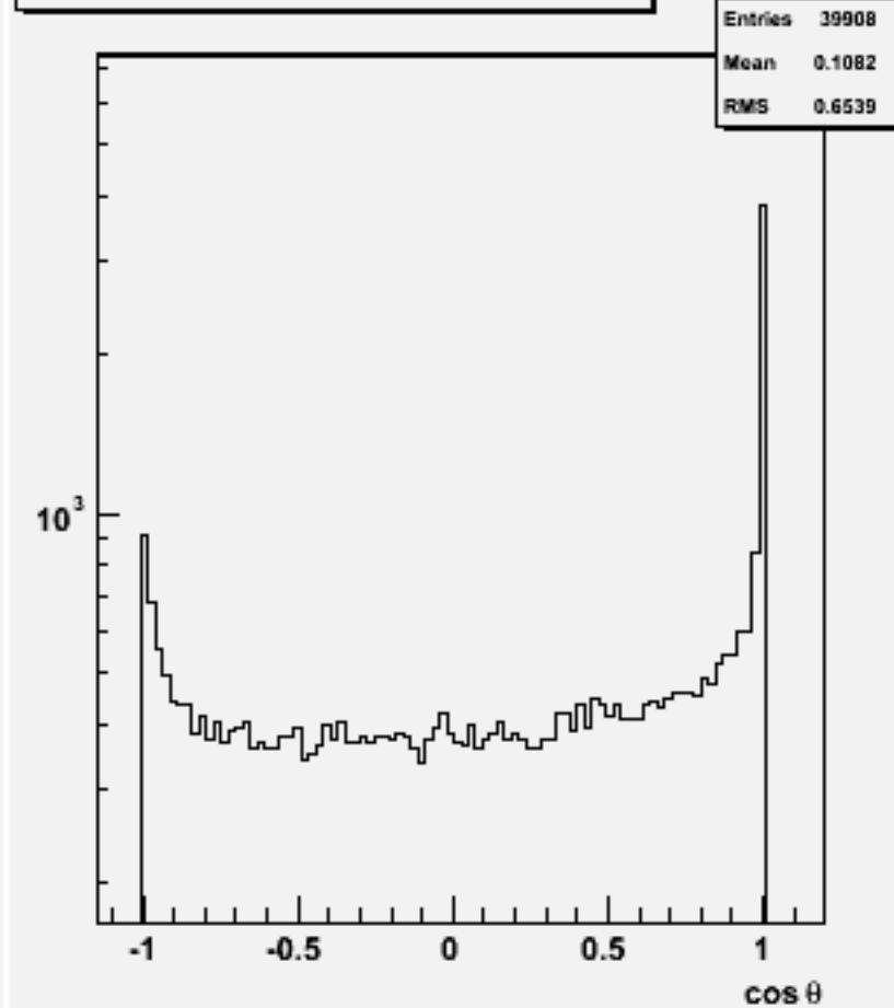
Jet cos \theta (All jets)w100833 e2e2n2e2sc_o
