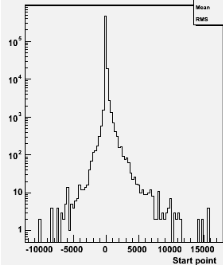
Start point Z : w100832 e2e2n2e2sc_o
