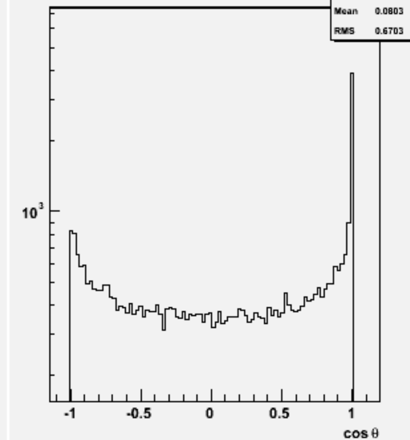
Jet cos \theta (All jets)w100832 e2e2n2e2sc_o
