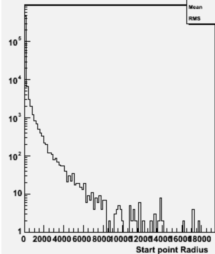
Start point R : w100832 e2e2n2e2sc_o
