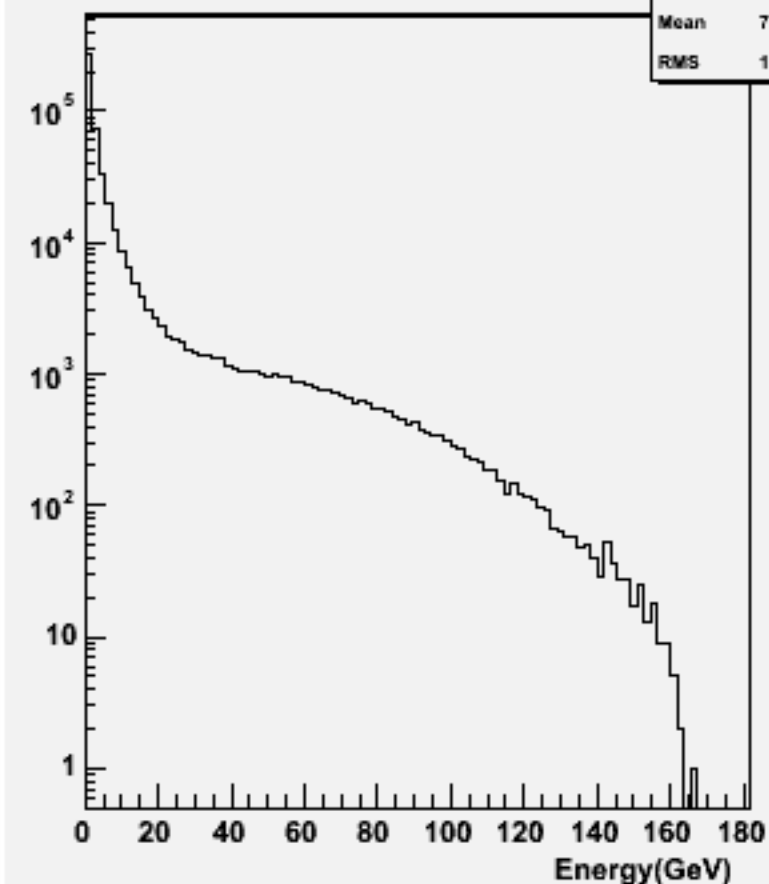
Particle Energy : w100832 e2e2n2e2sc_o
