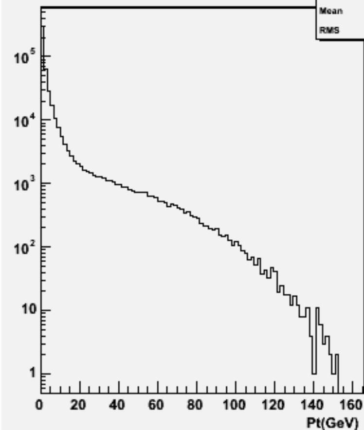
Particle Pt : w100832 e2e2n2e2sc_o
