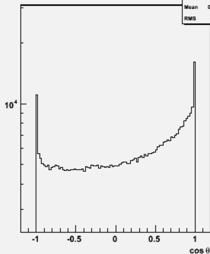
Particle cosθ : w100832 e2e2n2e2sc_o
