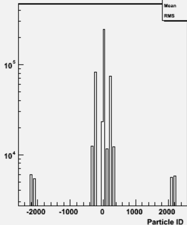
Particle ID : w100832 e2e2n2e2sc_o
