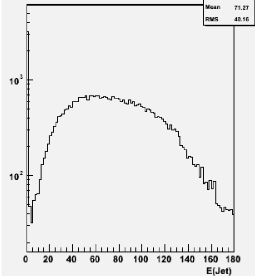
Jet energies(All jets)w100832 e2e2n2e2sc_o
