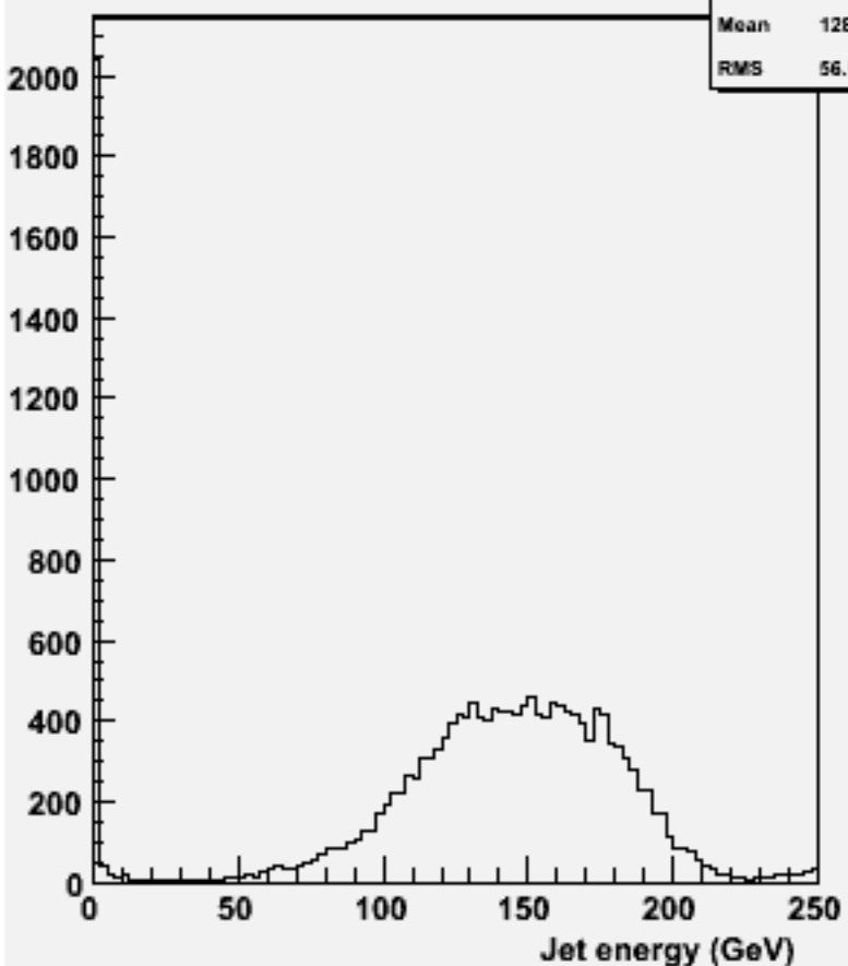
energy for 2-jets :w100828 e2e2n2e2du_o
