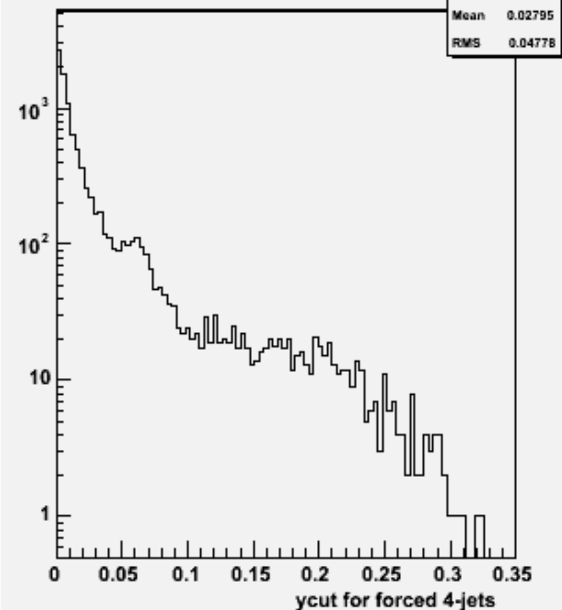
Ycut for 4-jets :w100828 e2e2n2e2du_o
