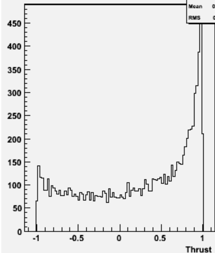
cos \Theta (thrust) w100828 e2e2n2e2du_o
