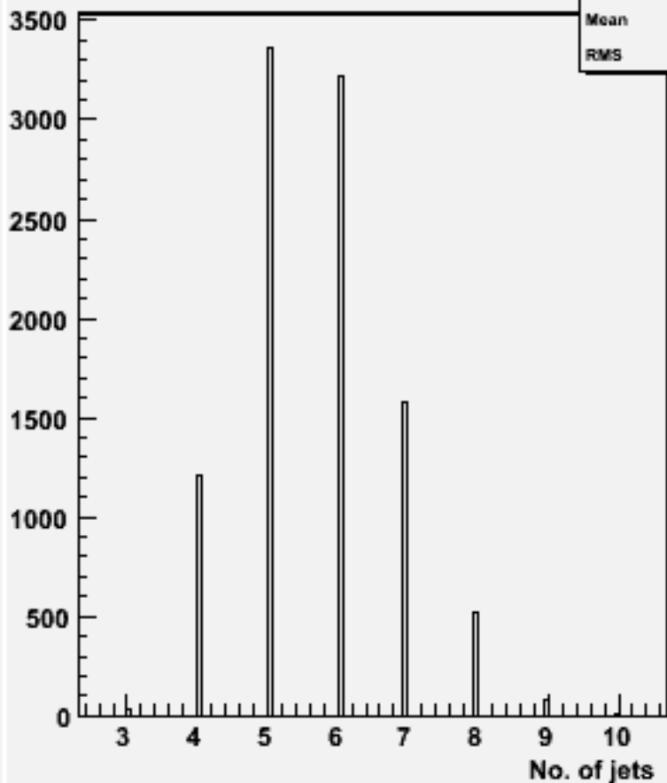
No. jets (ycut=0.001) : w100828 e2e2n2e2du_o
