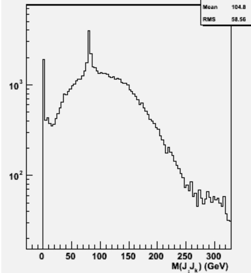
2jets mass(All comb)w100828 e2e2n2e2du_o
