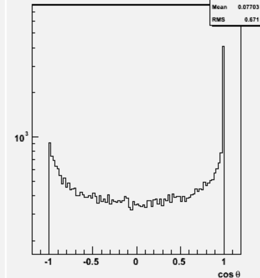
Jet cos \theta (All jets)w100828 e2e2n2e2du_o
