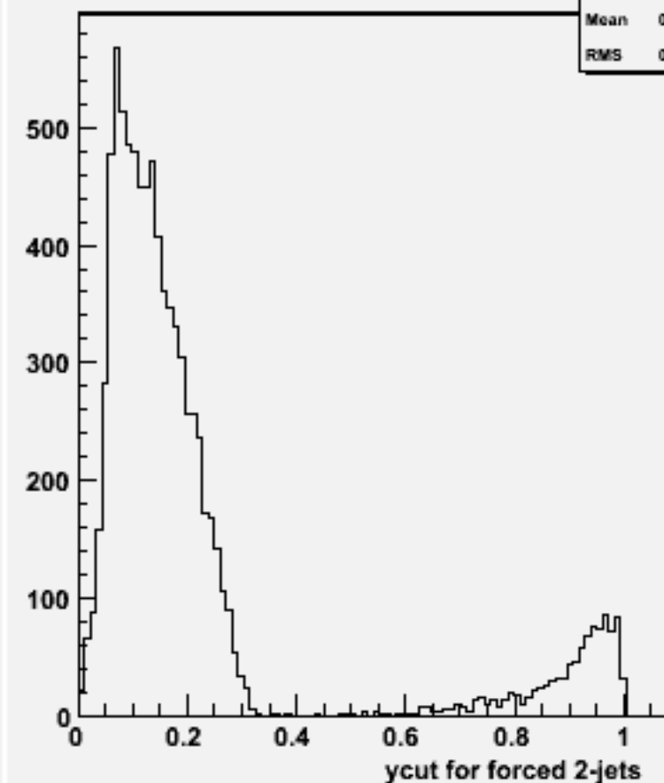
Ycut for 2-jets :w100828 e2e2n2e2du_o
