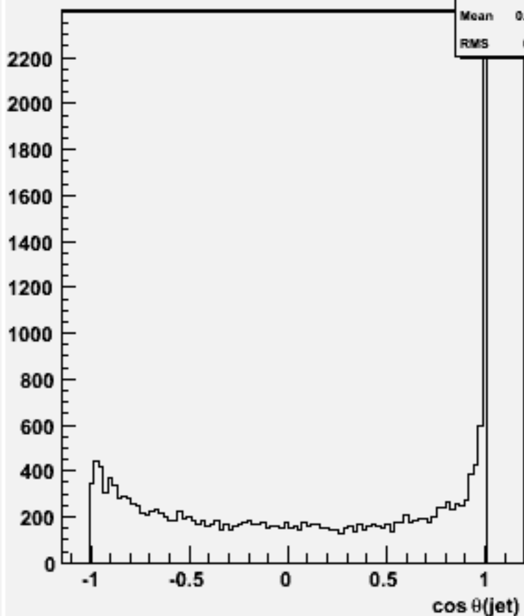
cos \theta for 2-jets :w100828 e2e2n2e2du_o
