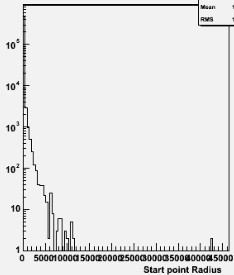
Start point R : w100828 e2e2n2e2du_o
