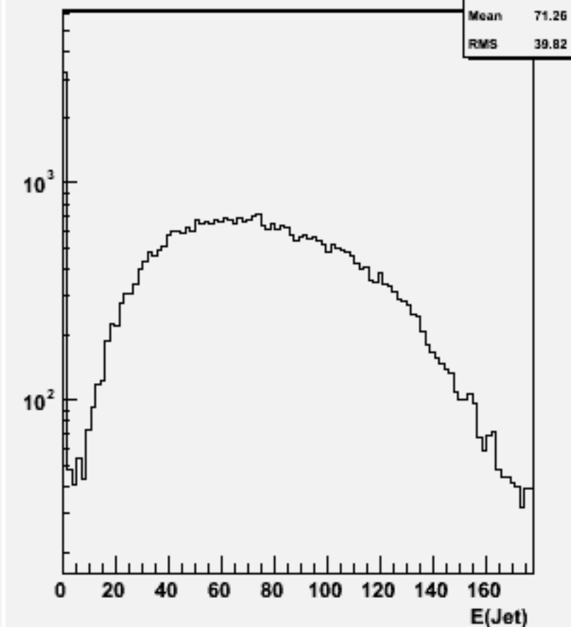
Jet energies(All jets)w100828 e2e2n2e2du_o
