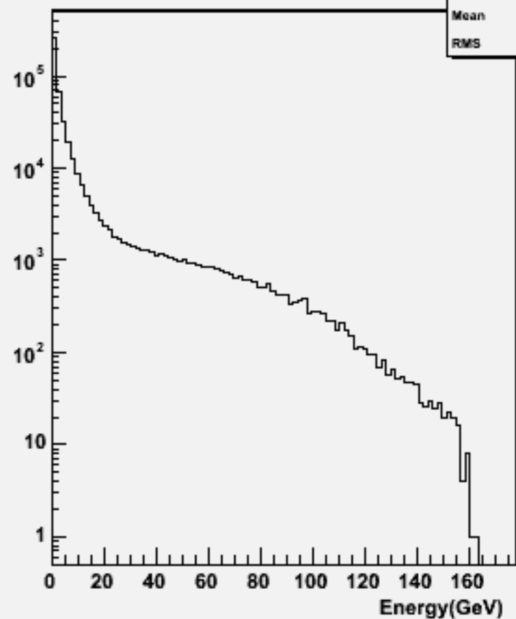
Start point R : w100828 e2e2n2e2du_o
