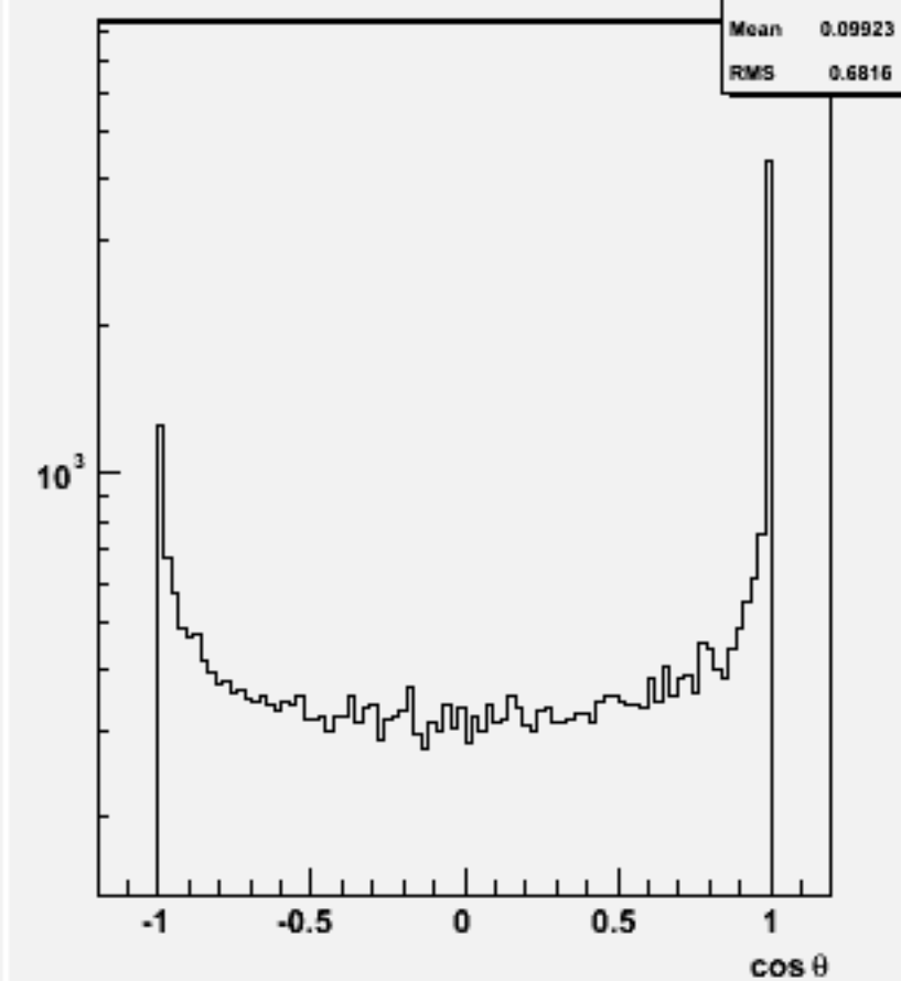
Jet cos theta (All jets)w100825 e2e2n2e2e3n3_o
