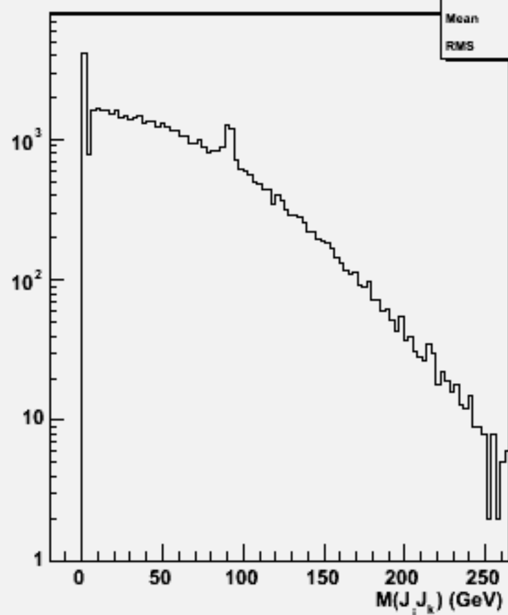
2jets mass(All comb)w100825 e2e2n2e2e3n3_o
