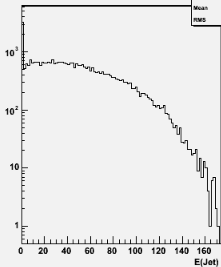
Jet energies(All jets)w100825 e2e2n2e2e3n3_o
