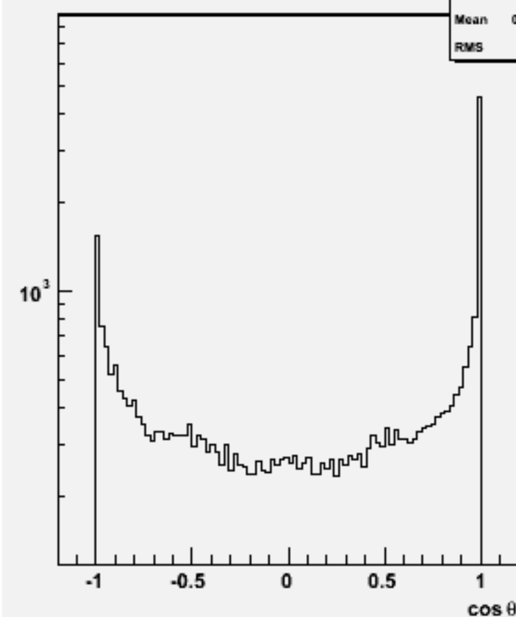
Jet cos \theta (All jets)w100821 e2e2n2e2e2n2_o
