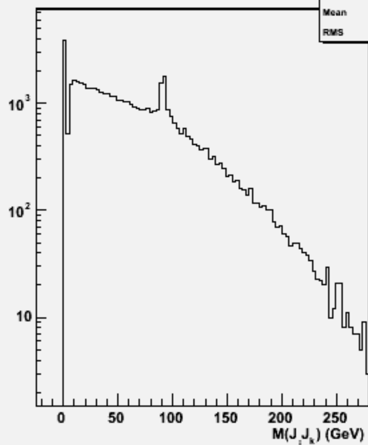
2jets mass(All comb)w100821 e2e2n2e2e2n2_o
