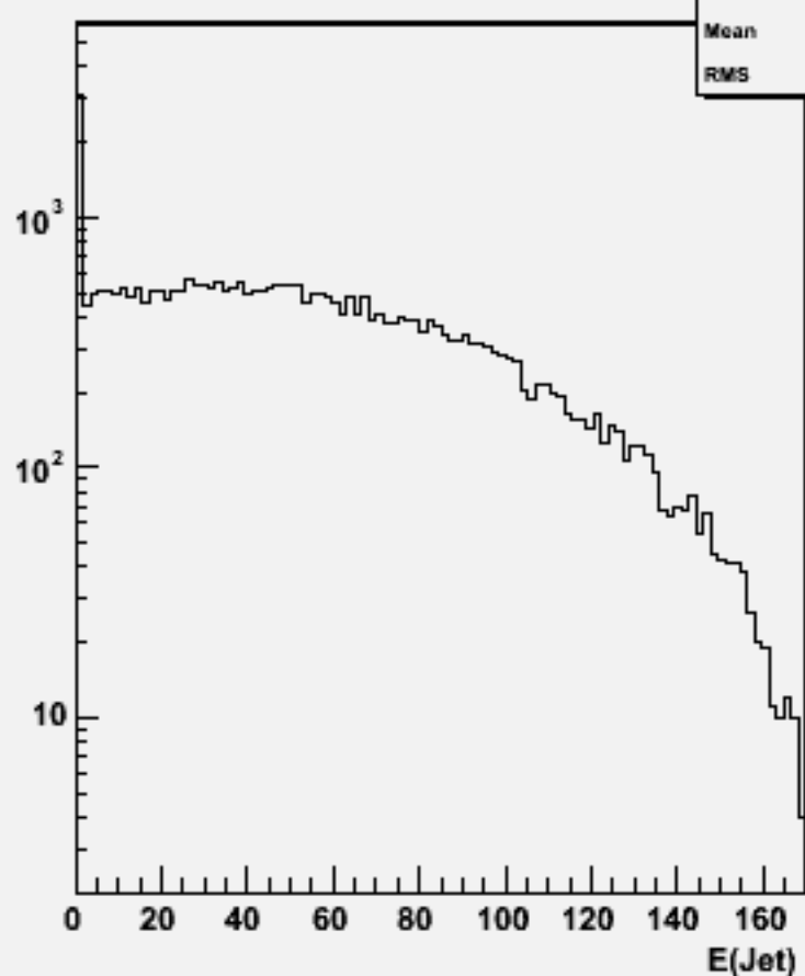
Jet energies(All jets)w100821 e2e2n2e2e2n2_o
