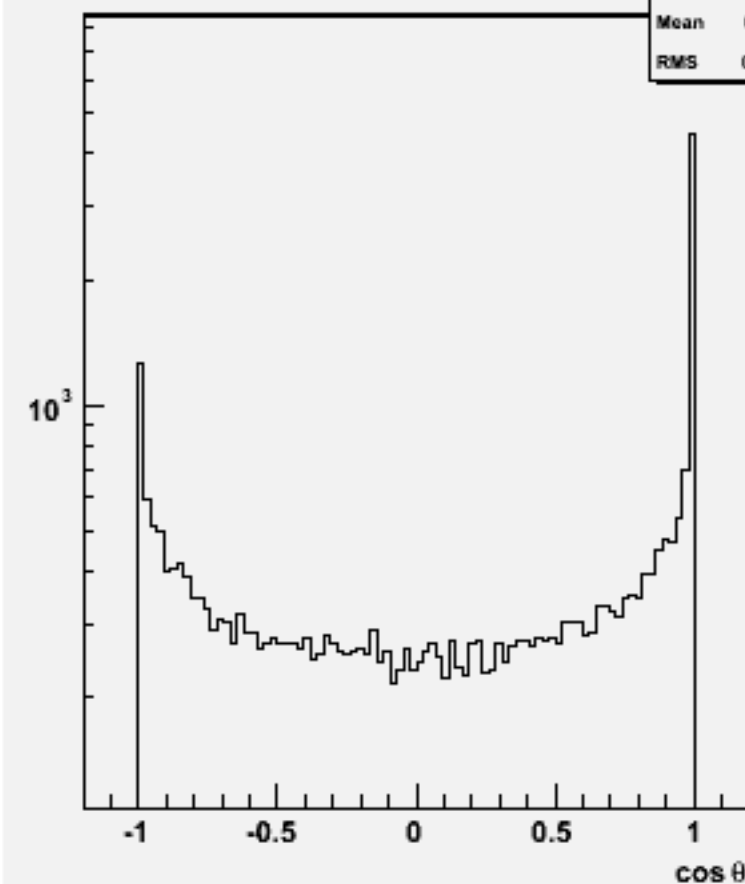
Jet cos \theta (All jets)w100820 e2e2n2e2e2n2_o
