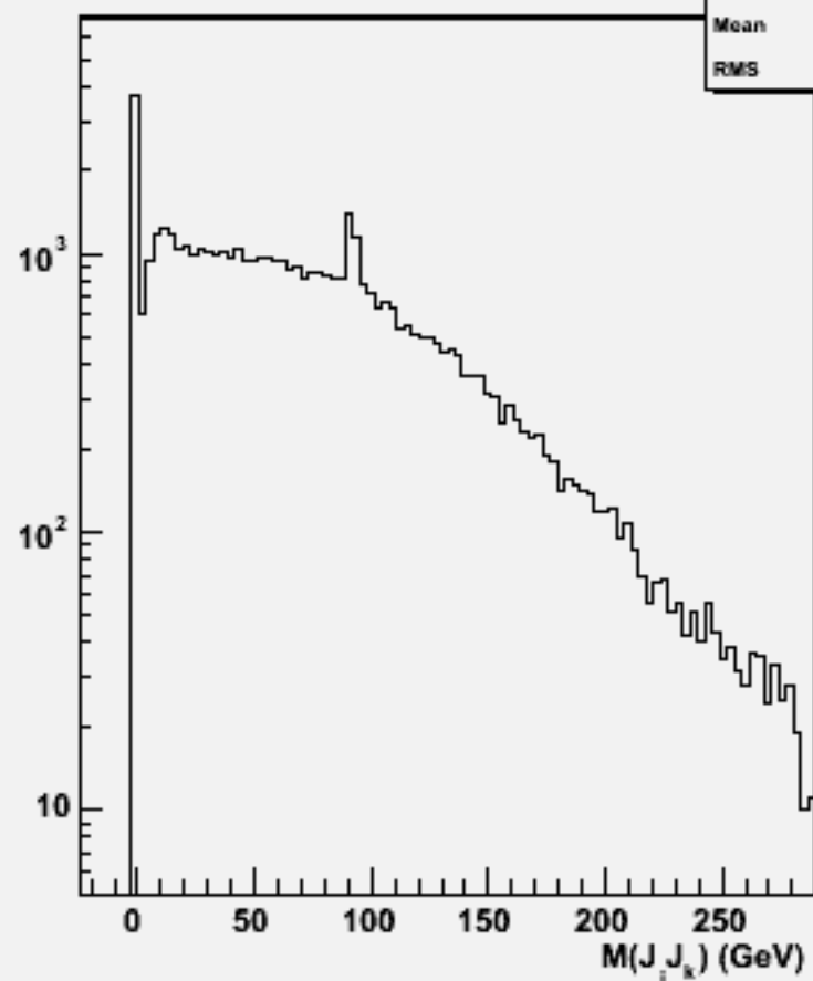
2jets mass(All comb)w100820 e2e2n2e2e2n2_o
