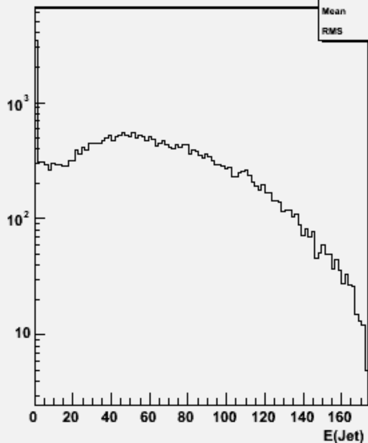
Jet energies(All jets)w100820 e2e2n2e2e2n2_o
