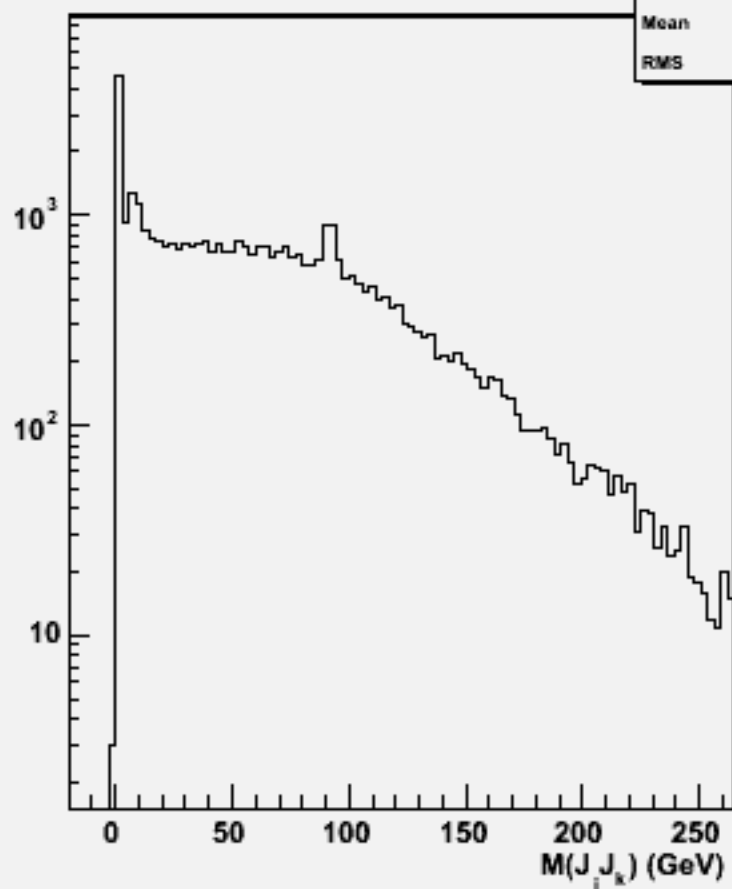
2jets mass(All comb)w100816 e2e2n2e2e1n1_o
