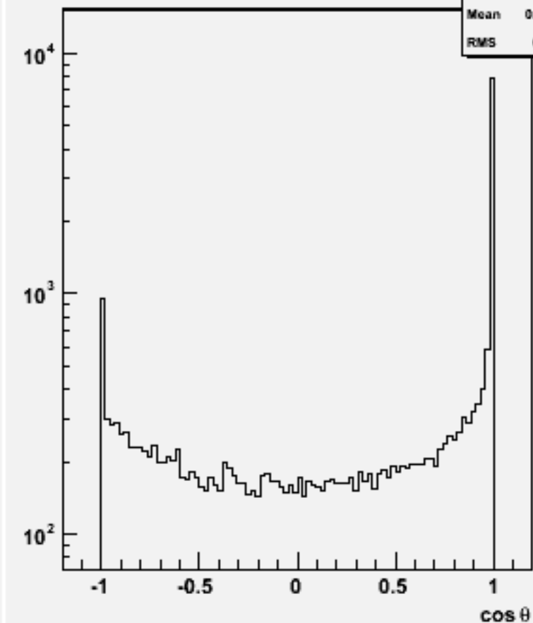
Jet cos \theta (All jets)w100816 e2e2n2e2e1n1_o
