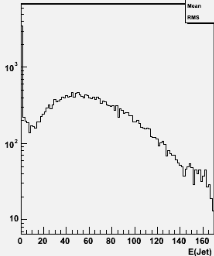
Jet energies(All jets)w100816 e2e2n2e2e1n1_o
